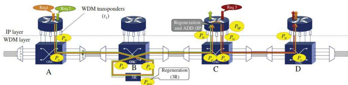
2.1. ábra. A Tl-IPoWDM hálózati illusztrációja [22]
