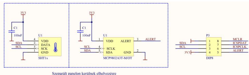
22. ábra: Hőmérsékletérzékelő szenzorok
