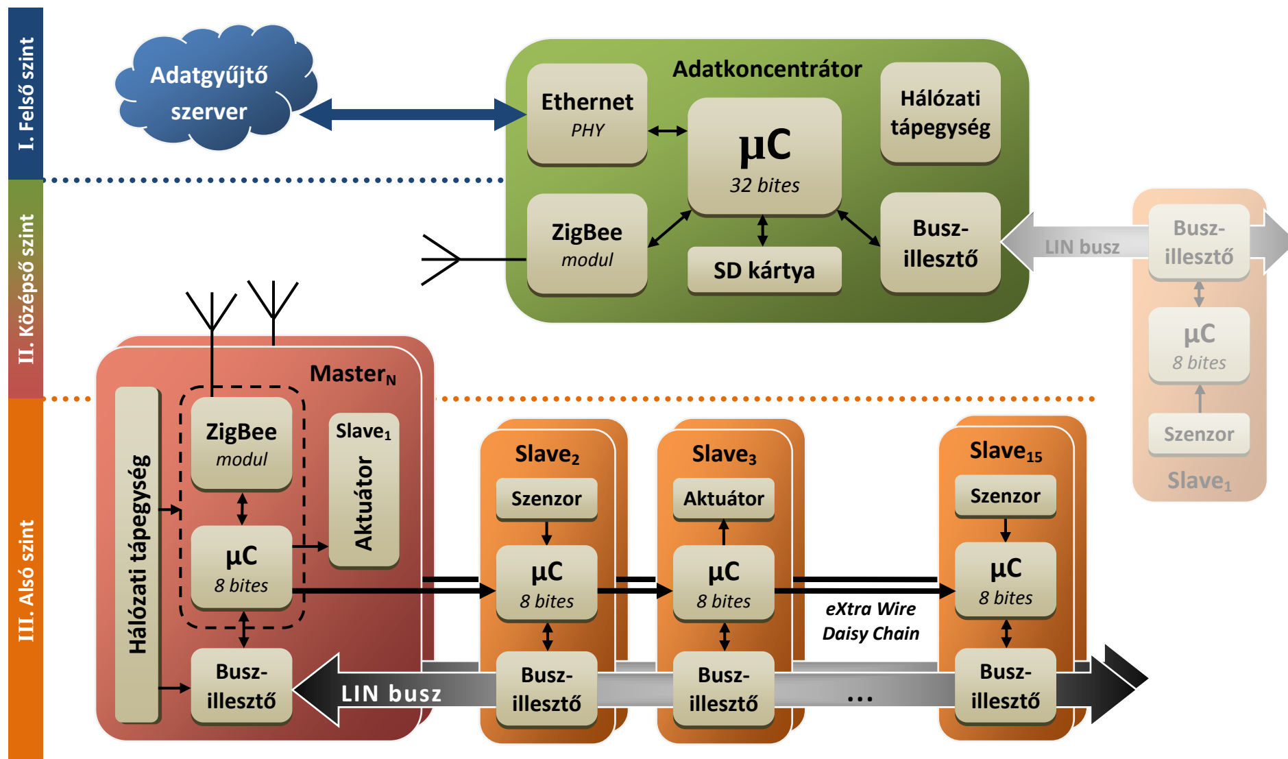
14. ábra: Hardver rendszerterv
