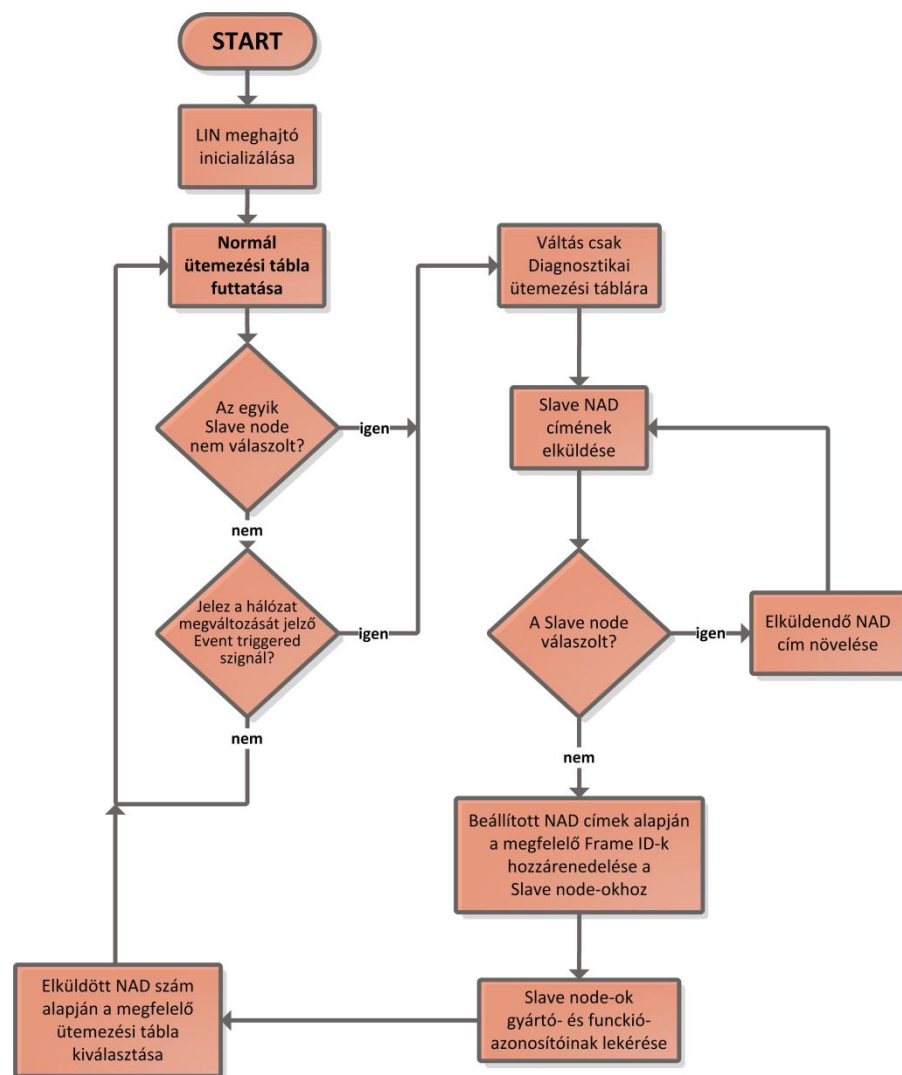
28. ábra: A Master egység LIN inicializálásának folyamatábrája
