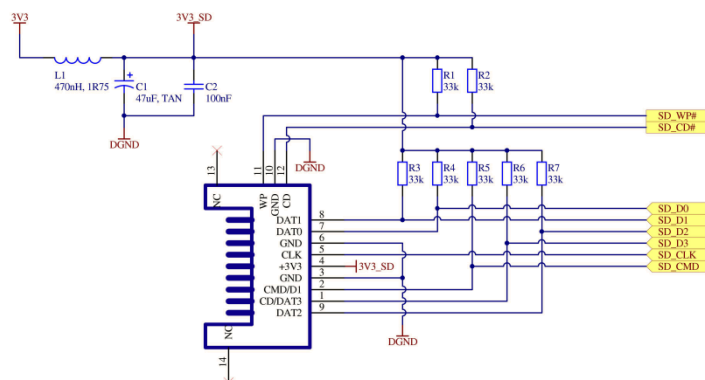
27. ábra: 4-bites SD kártya interfész
