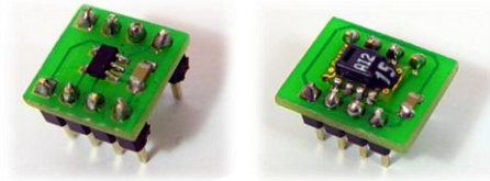
23. ábra: MCP9800 és SHT1x szenzorokhoz készített adapter panelek
