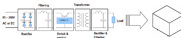
16. ábra: myrra gyártmányú tápegység kocka blokkvázlata [20]
