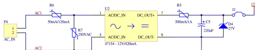
17. ábra: A Master egység hálózati tápegysége
