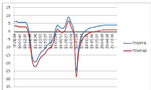
47. ábra Elektronika doboz - AD és PS hőmérsékletei
