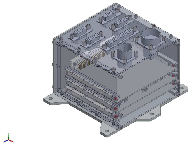
23. ábra Elektronika doboz
