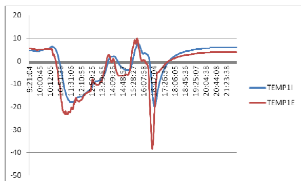
49. ábra Optikai doboz külső és belső hőmérséklete
