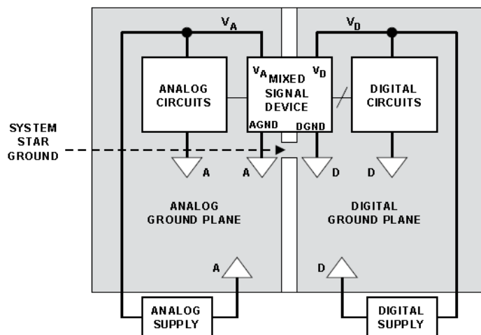
29. ábra Földelés kialakítása
