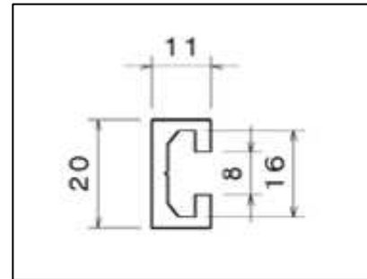
8. ábra BEXUS15 gondola, és a sín mechanikai méretei
