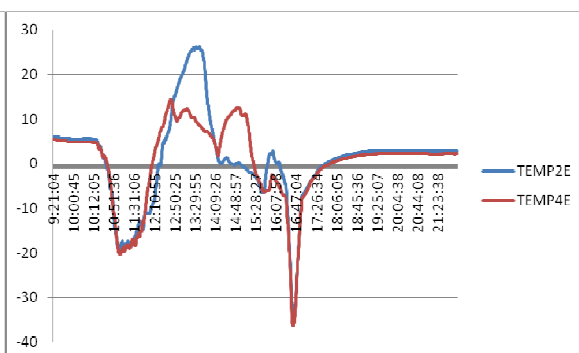
50. ábra Azonos alapllemezen levő optikai dobozok külső hőmérséklete
