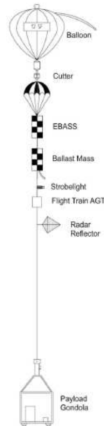
7. ábra BEXUS15 felépítése
