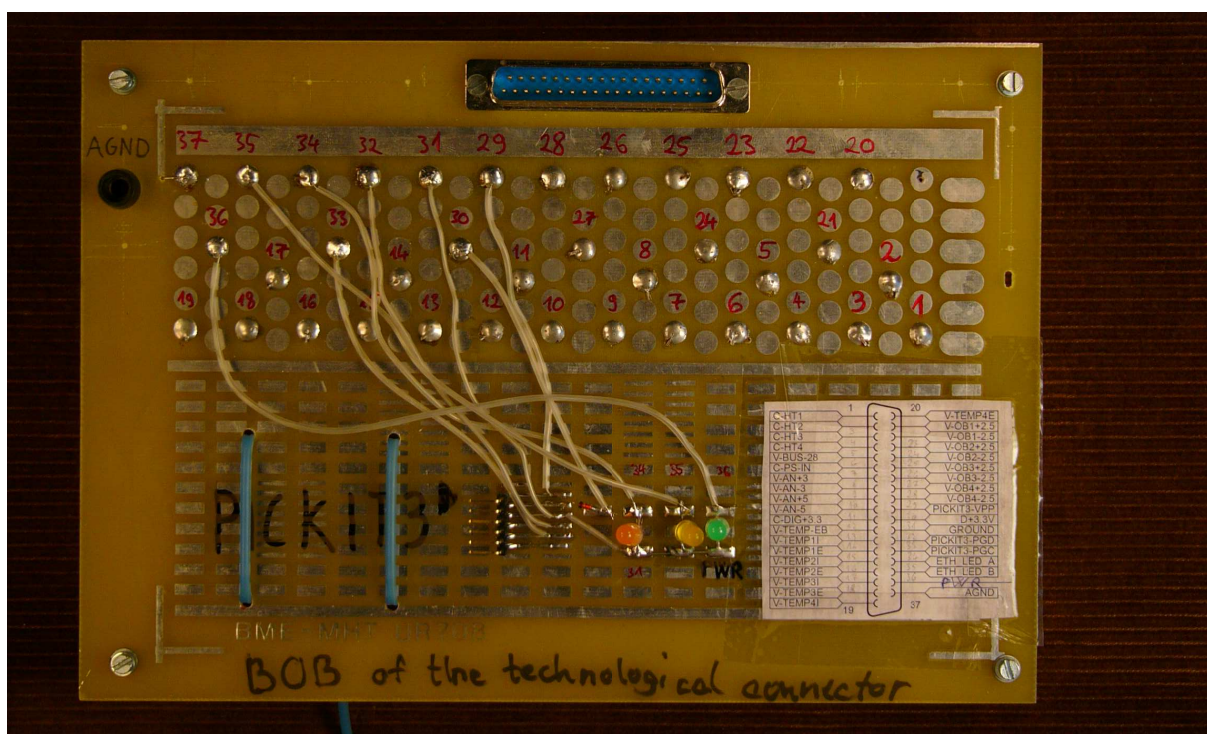
41. ábra Break out box
