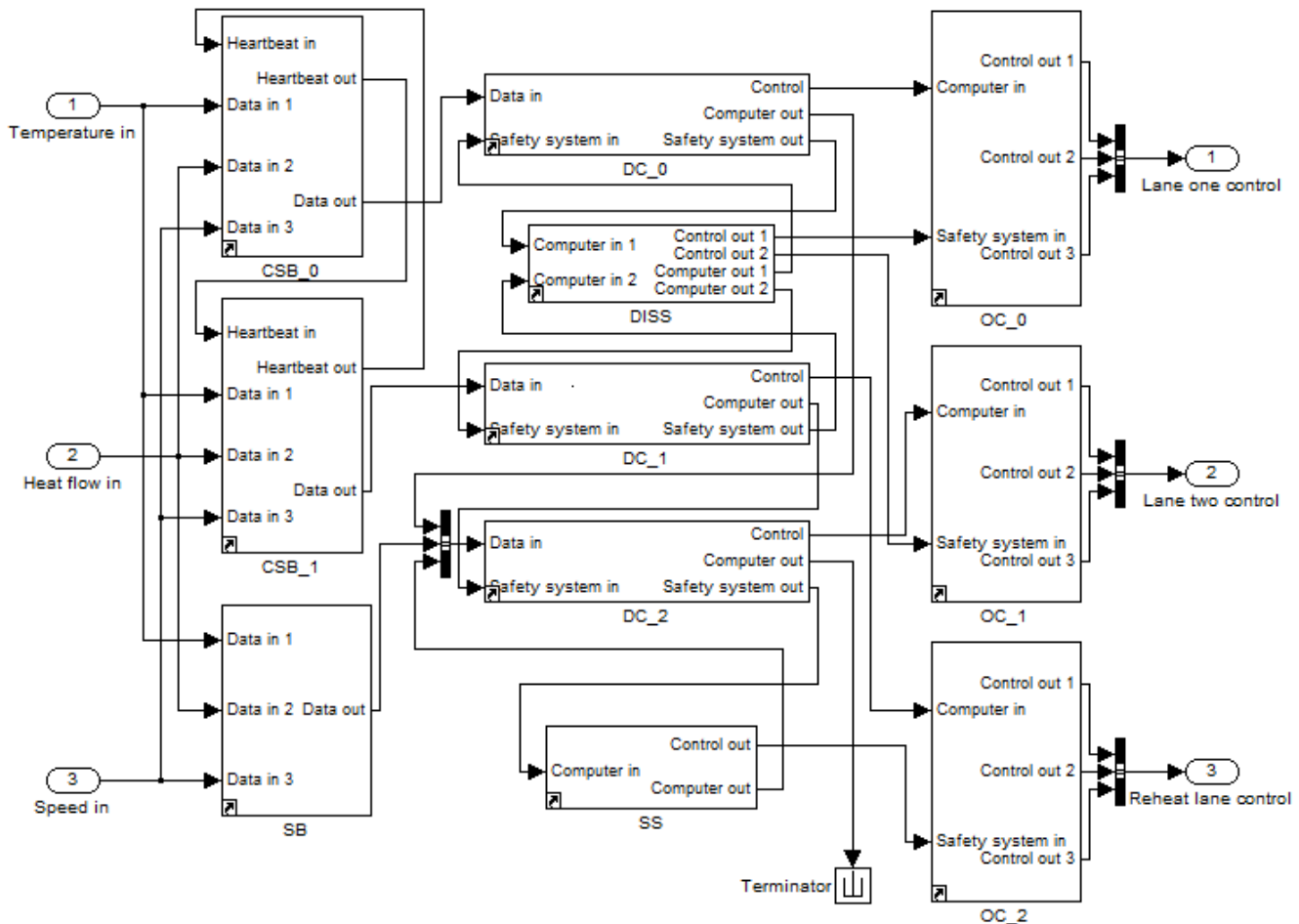
2.3. ábra. Az RB199 motorvezérlő SIMULINK modellje
