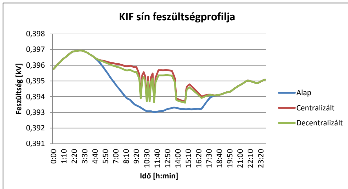
16. ábra: A KIF sín feszültségprofilja a különböző napelem elrendezési esetekben nyári felhős adatokkal.
