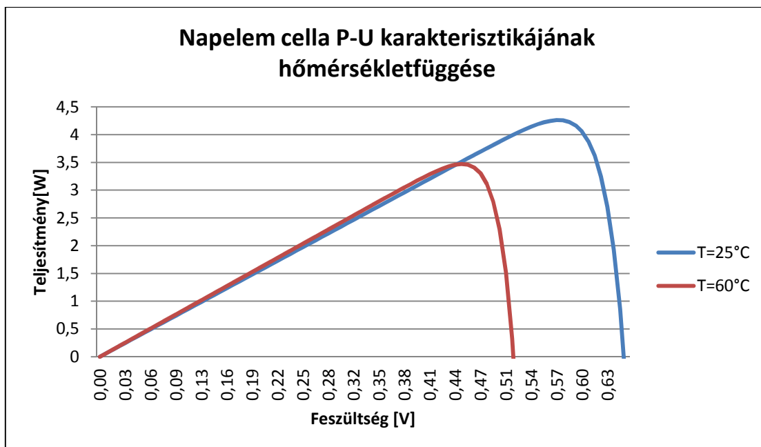
4. ábra: A napelem P-U karakterisztikája különböző hőmérsékleteken, de ugyanazon napfényintenzitású besugárzással ( I_L=7,81\text{A} ).
