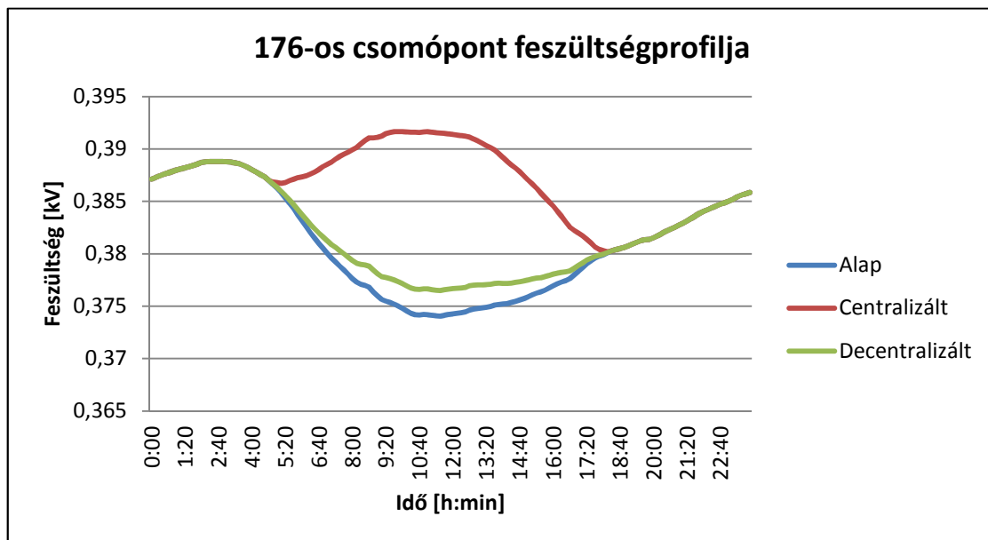
11. ábra: A 176-os csomópont feszültségprofilja a különböző napelem elrendezések esetében nyári adatokkal.
