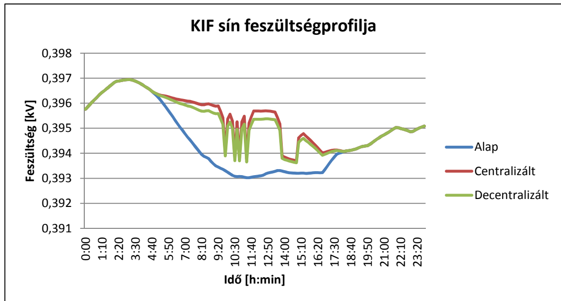
16. ábra: A KIF sín feszültségprofilja a különböző napelem elrendezések esetében nyári felhős adatokkal.
