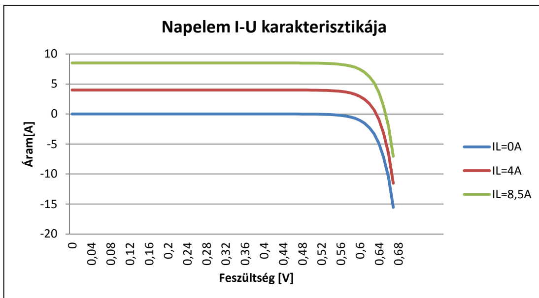
2. ábra: A napelem I-U karakterisztikája különböző megvilágításokra.
