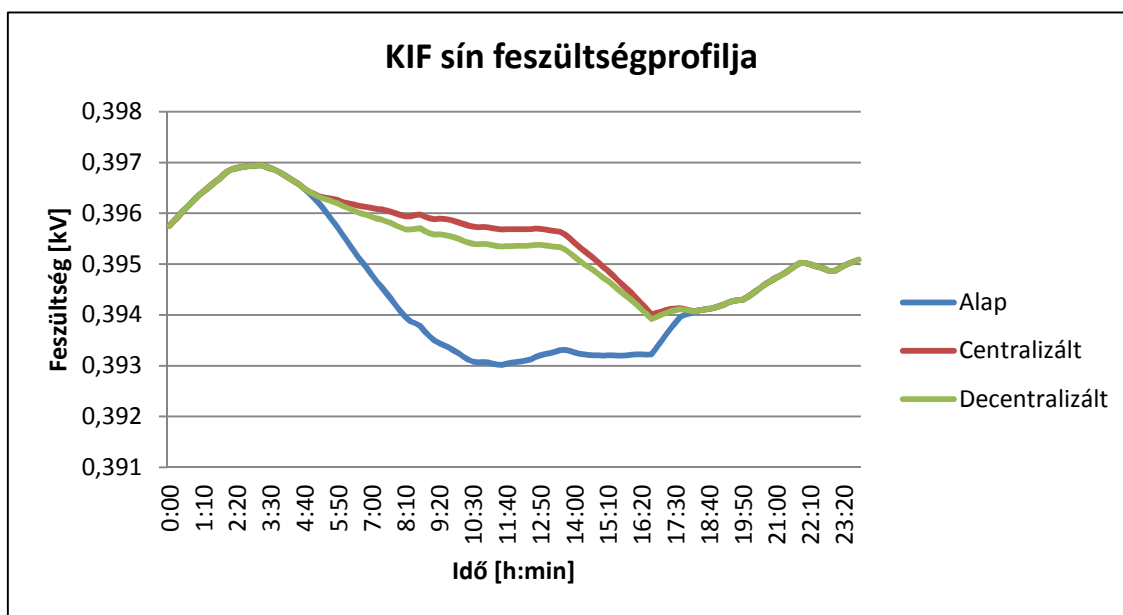
13. ábra: A KIF sín feszültségprofilja a különböző napelem elrendezéses esetekben nyári adatokkal.
