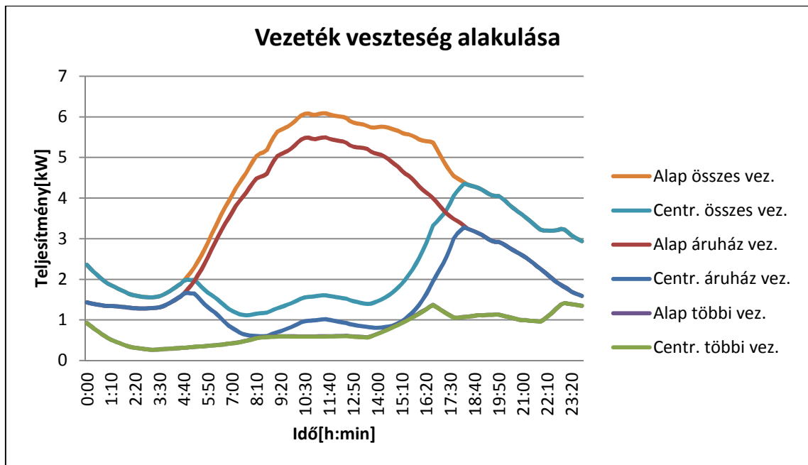
20. ábra: Az elosztóhálózat vezetékeinek veszteségei a centralizált napelem elrendezés és a napelemek nélküli topológia esetében.
