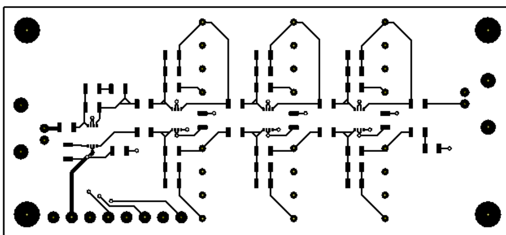
49. ábra: az áramkör elülső lapjának fémezése
