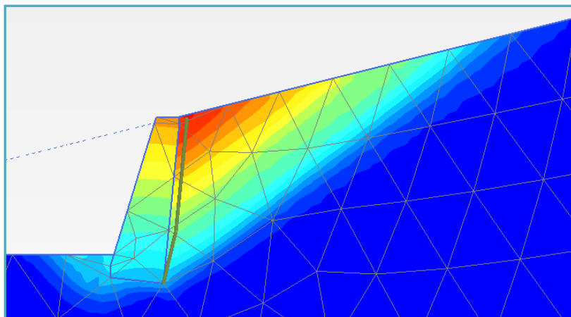
22. ábra: Végesseleemes számítás eredménye. Látható a fal teteje mögötti fellazult föld
