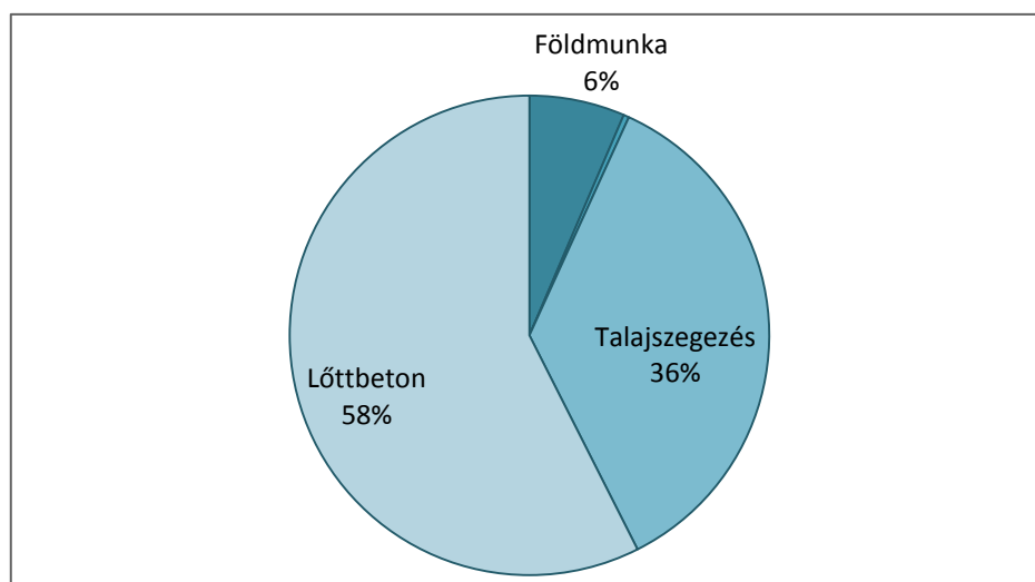
39. ábra: A talajszegezés költségeinek egymás közötti megoszlása, 6 méteres magas, homok talaj esetében
