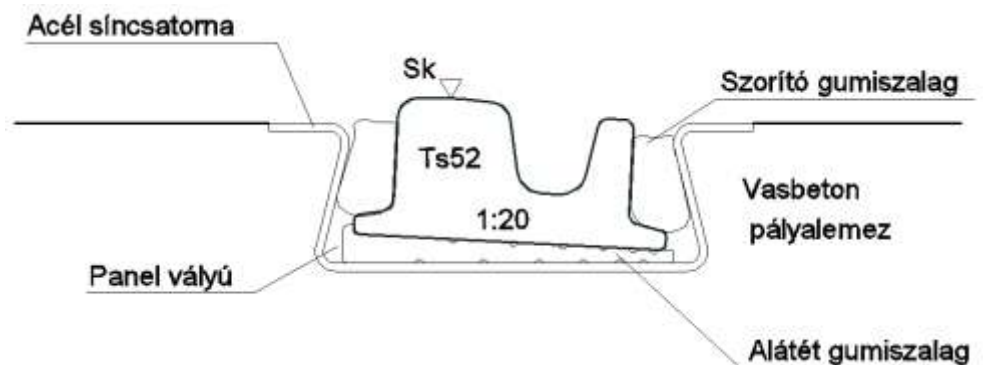
13. ábra: Ékes-alátét gumiszalagos kialakítású síncsatorna
