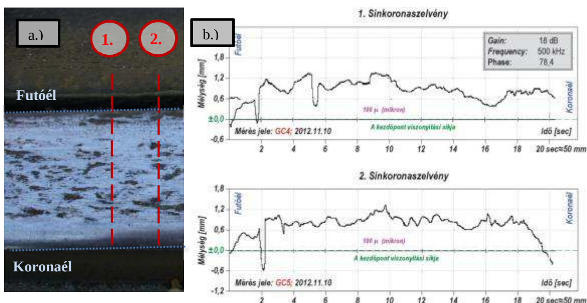
20. ábra: Felületi meghibásodások keresztirányú sínszelvények mérése a Kálvin téren örvényáramos műszerrel
