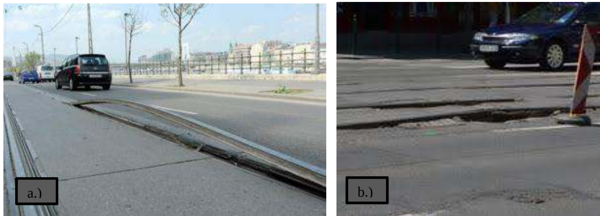
9. Fénykép: A sínszál függőleges kivetődés nagypaneles (a), és RAFS felépítményben.(b)
