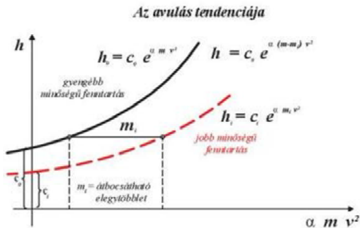
4. ábra: Vágányszabályozás hatása a romlási folyamatra [9]
