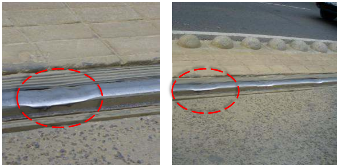
14. Fénykép: Periodikus kivölgyelődés a sínkoronán
