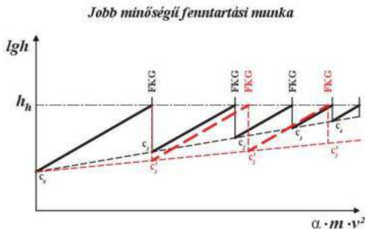
8. ábra: Jobb fenntartási munka lassítja az avulási folyamatot [9]
