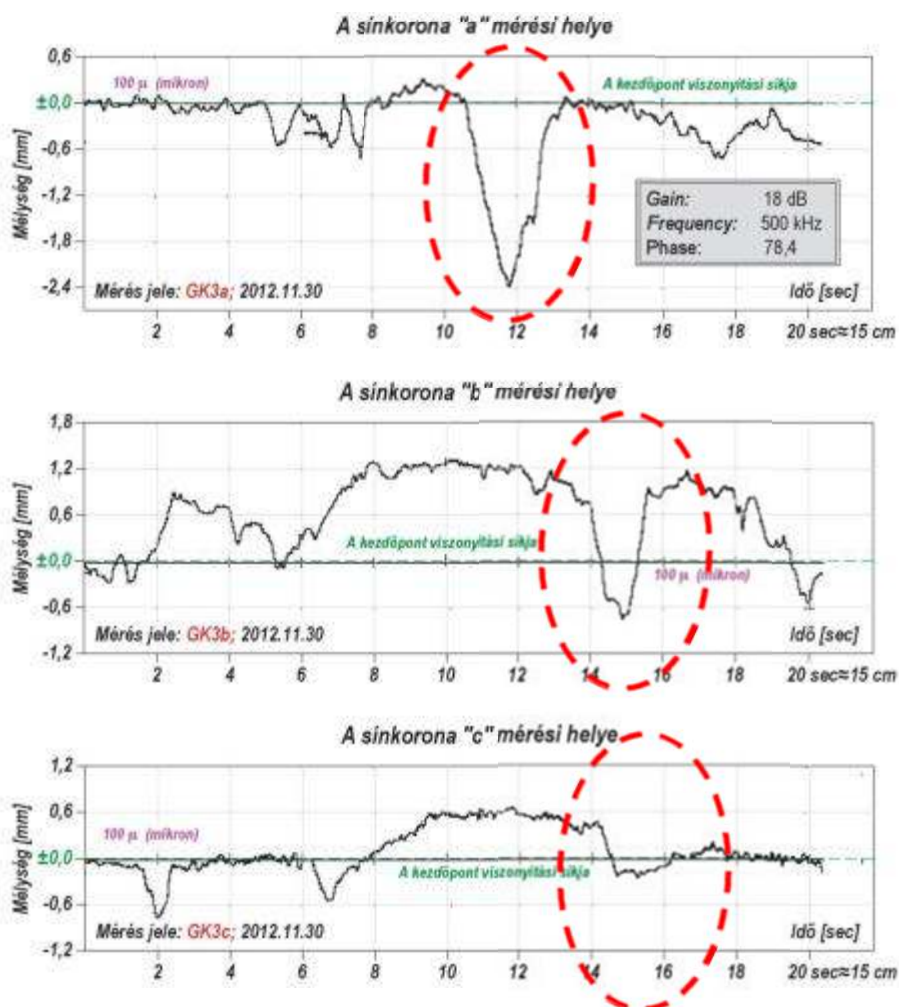
8. ábra: A második hajtott forgóváz megállási helye Szent Gelért téren Kelenföld felé
