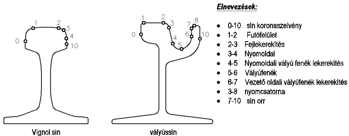
15. ábra: Közúti vasúti sínkorona profil egyes szakaszainak elnevezése
