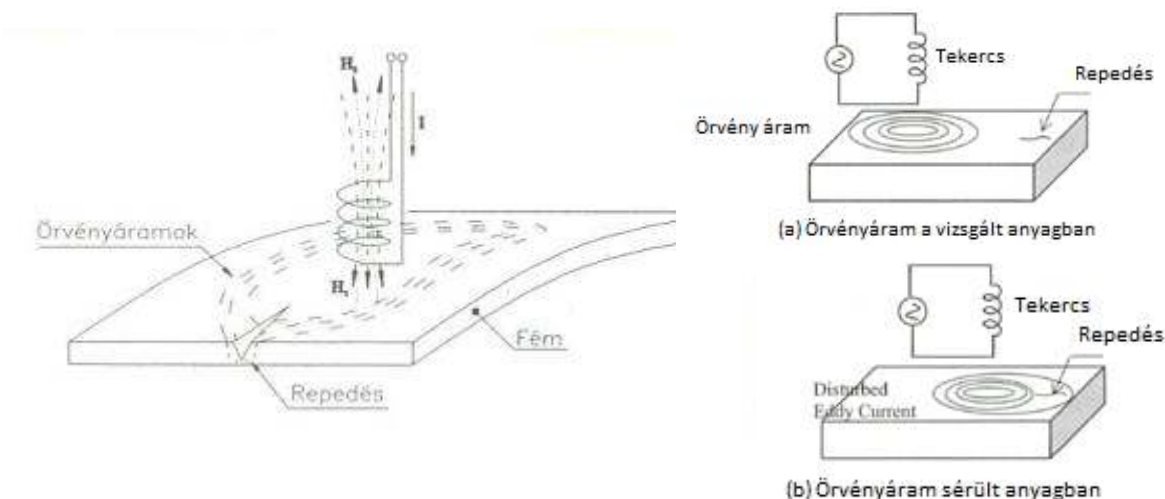
19. ábra: Örvényáramos vizsgálat elve
