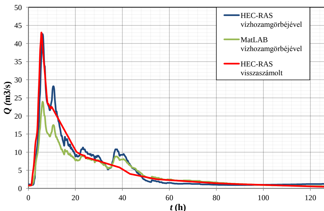
8. ábra: 2010. májusi árhullám vízhozam idősorai. (Kékkel a HEC-RAS vízhozamgörbéjével számított, zölddel a MatLAB vízhozamgörbéjével számított, pirossal a HEC-RAS-ban visszaszámított vízhozamok).
