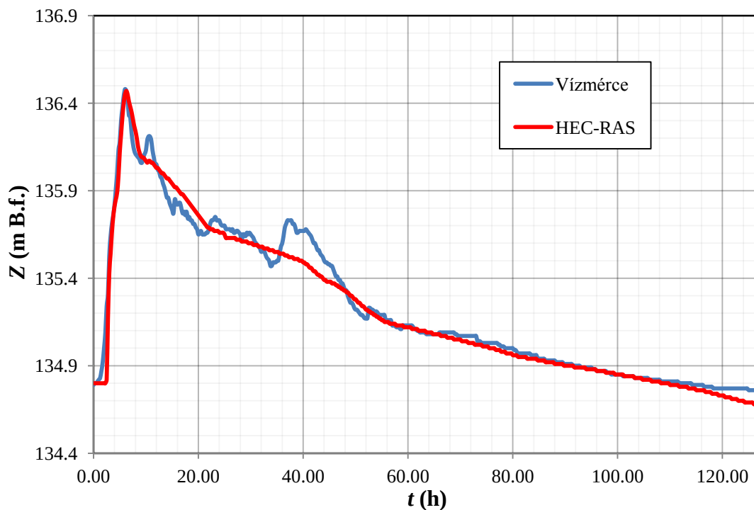
7. ábra: 2010. májusi árhullám vízállás idősora (kékkel a vízmérce szelvényében regisztrált értékek, pirossal a HEC-RAS által számolt értékek).
