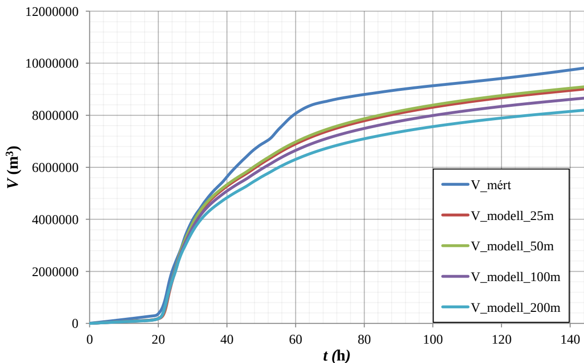
28. ábra: 2010. májusi árhullám során, a patakon levonuló kumulált víztérfogatok, különböző felbontású rácsháló (25, 50, 100, 200 m) esetén.
