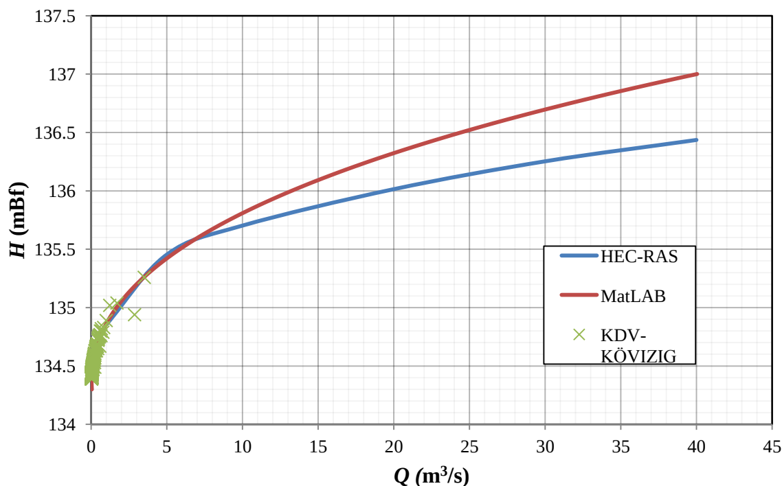
5. ábra: Vízhozamgörbék (pirossal a 2009-es év MatLAB segítségével számított vízhozamgörbéje, kékkel a HEC-RAS által, permanens futás esetén számított, a KDV-KÖVIZIG által mért értékek zöld pontokkal).
