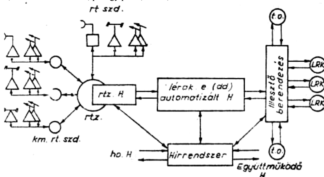
23. ábra Légvédelmi rakéta egység automatizált irányítási rendszere 267
