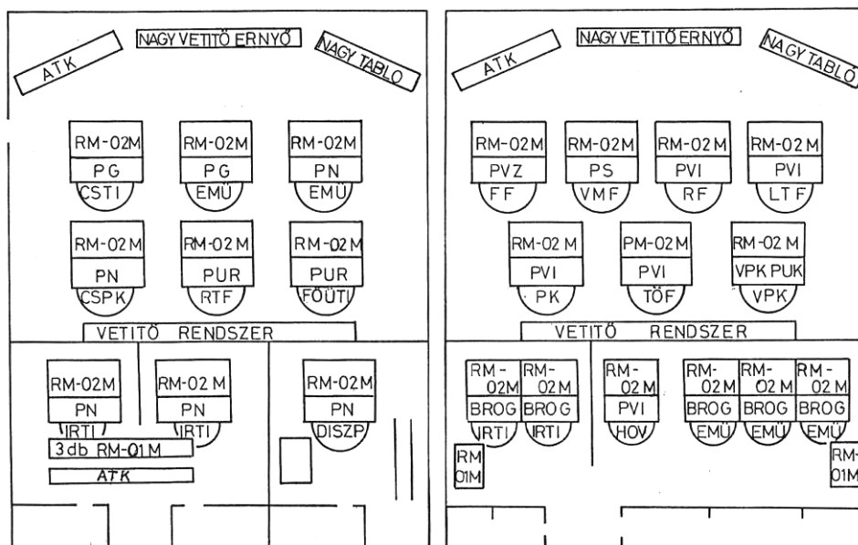
30. ábra Az ALMAZ-2 komplexum rádiólokációs és hadműveleti termeinek elvi vázlata 311
