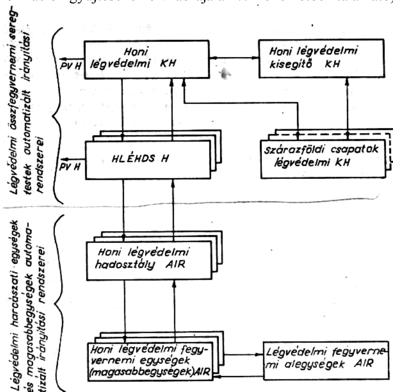
20. ábra Szovjet automatizált rendszerek elvi kapcsolata 247
