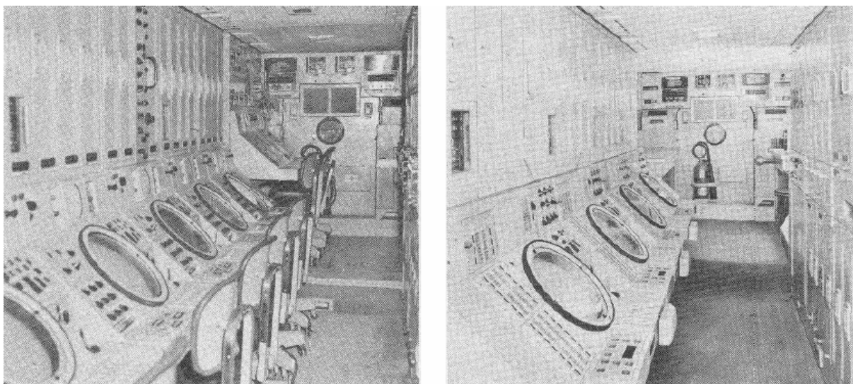
19. ábra A Missile Monitor harcvezetési kabinjának berendezései 240
