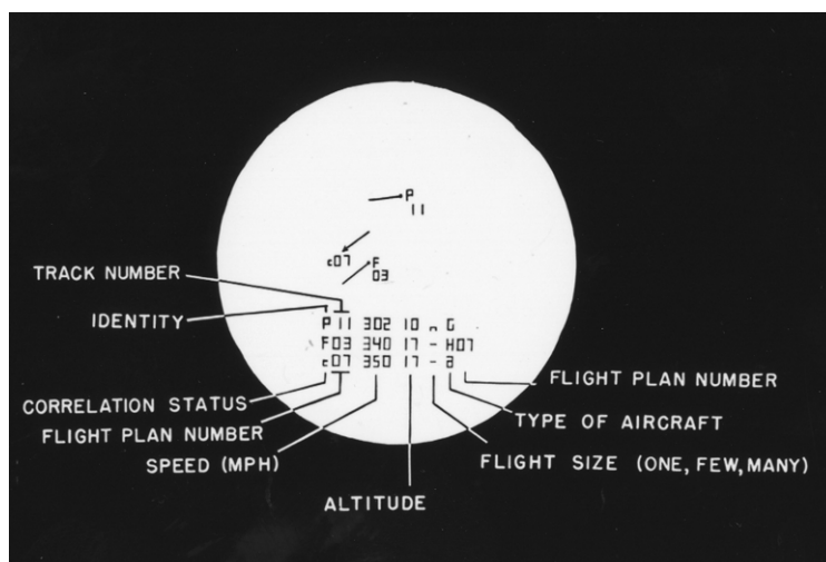
11. ábra Az azonosító indikátor képe 149
