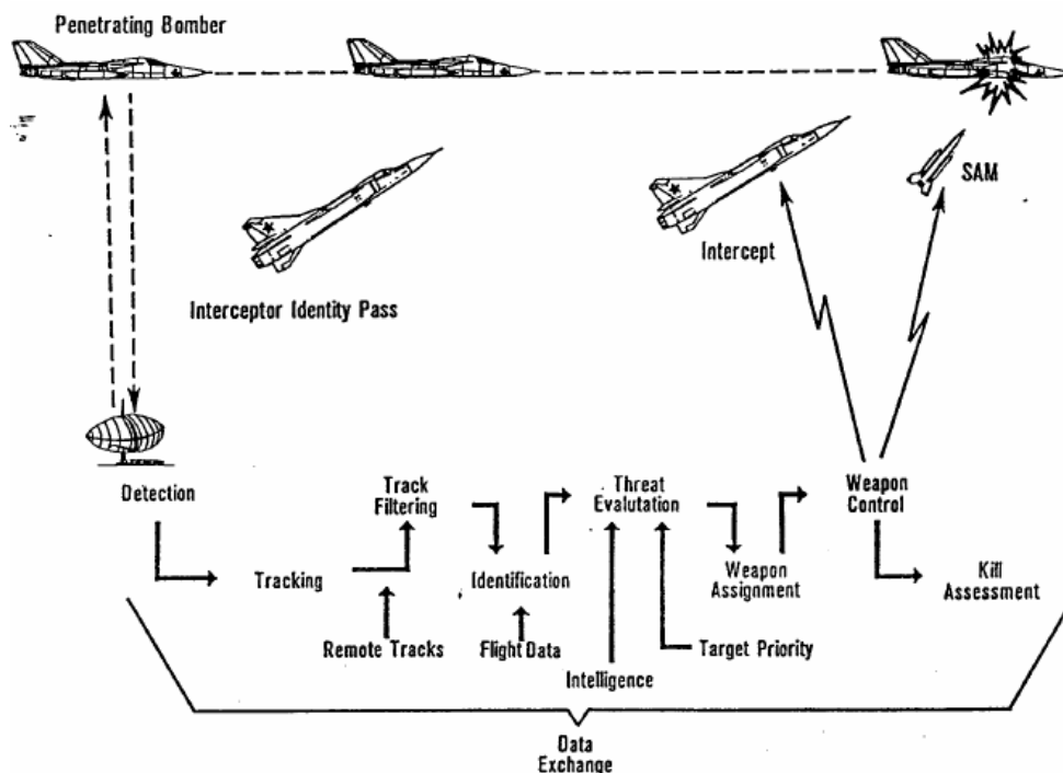
6. ábra A légvédelmi rendszer funkciói 73
