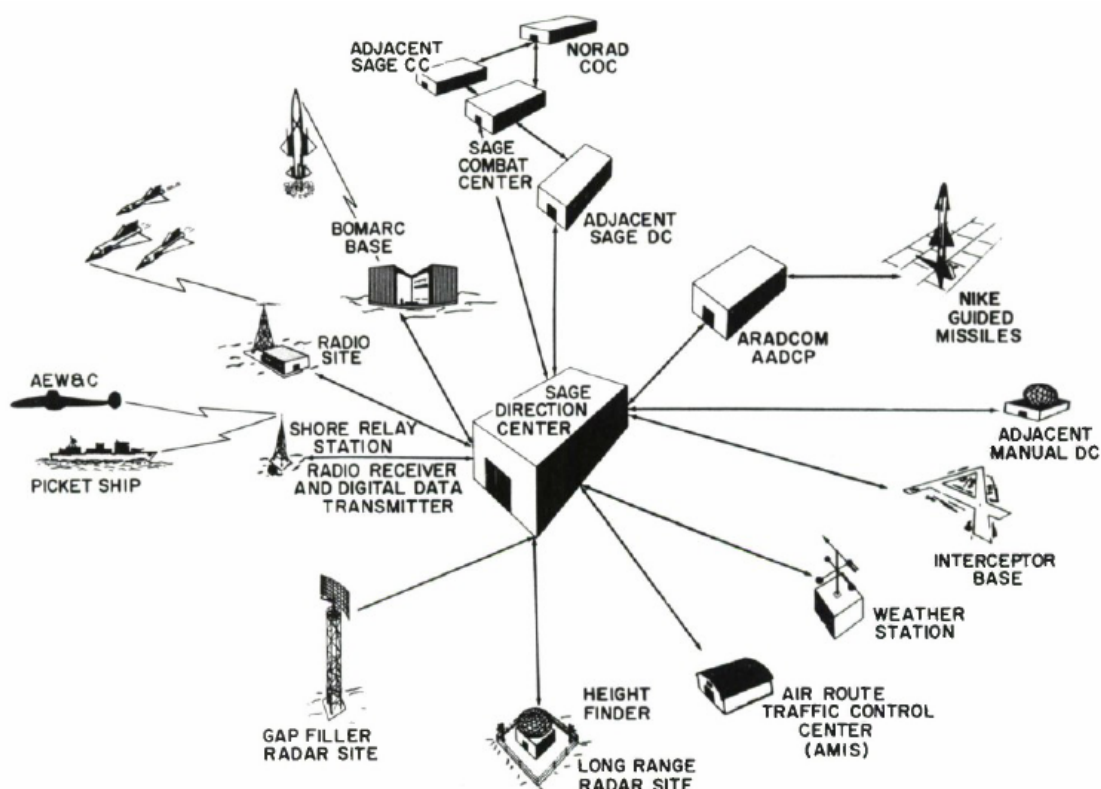
9. ábra A SAGE DC adatkapcsolati rendszer 139
