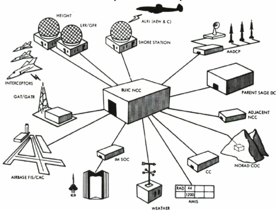
16. ábra A BUIC harcálláspont adatkapcsolatai 197
