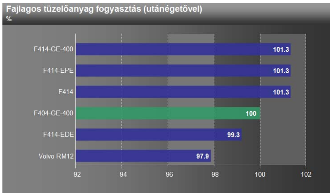
15. ábra: Fajlagos tüzelőanyag fogyasztások a referenciaként jelölt hajtóműhöz viszonyítva. 41
