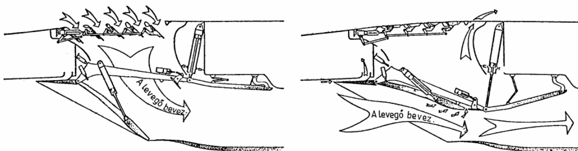
23. ábra: A MiG-29 levegő-beömlőnyílás működése 200km/h alatt (bal) és felett (jobb). 55
