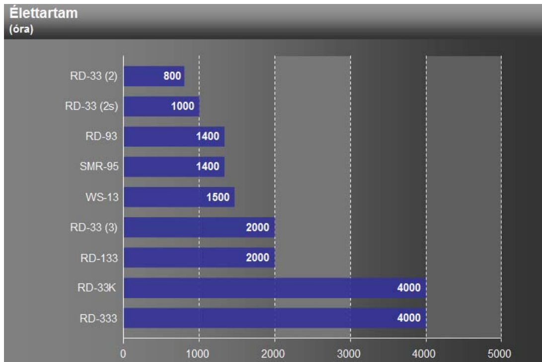
35. ábra: A Klimov hajtóműcsalád tagjainak élettartama. 72
