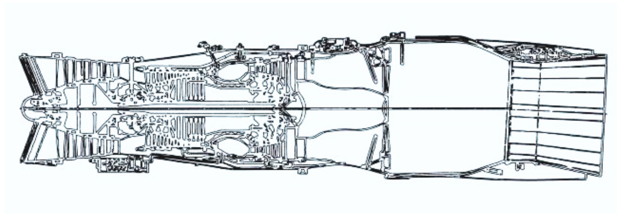
20. ábra: Figyeljük meg, hogy a hajtómű nem teljesen tengelyszimmetrikus.
