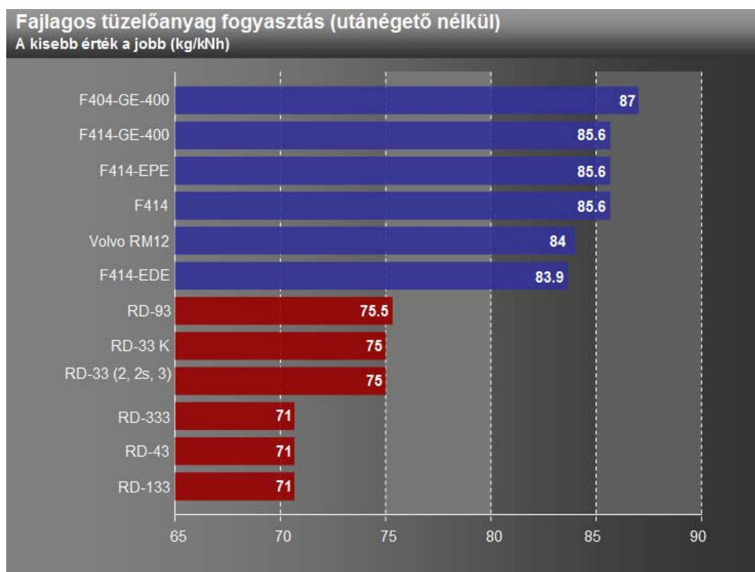
36. ábra: A fajlagos tüzelőanyag fogyasztás utánégetés nélkül. 73
