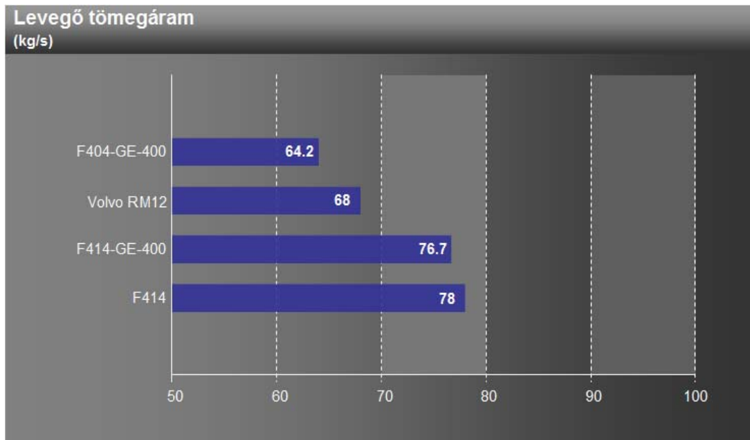
12. ábra: Levegő tömegáram. 38
