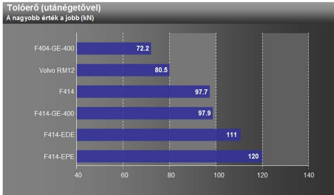
17. ábra: Tolóerő utánégetővel. 43
