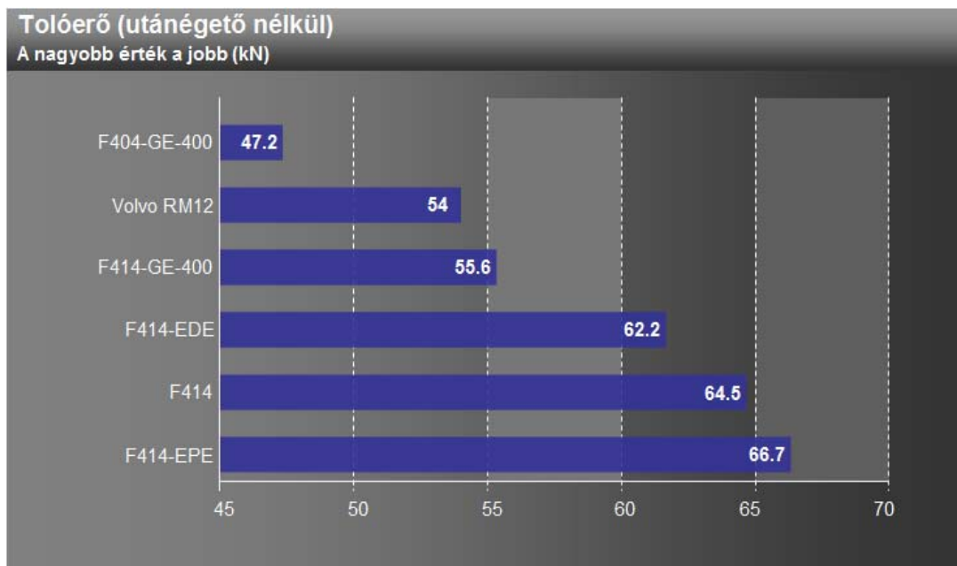
16. ábra: Tolóerő utánégető nélkül. 42
