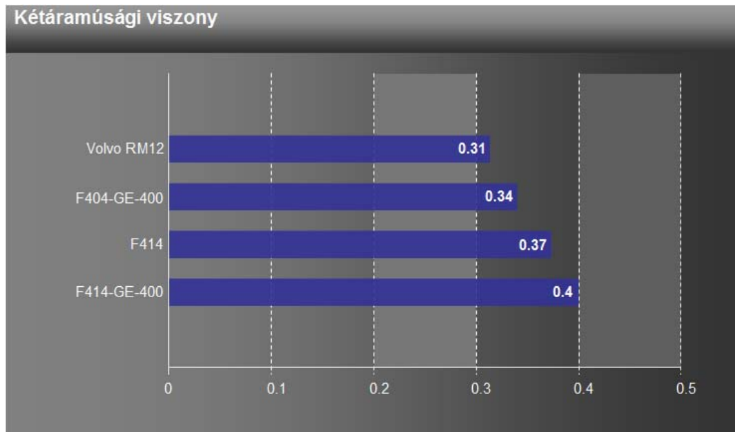
11. ábra: A kétáramúsági viszony. 37
