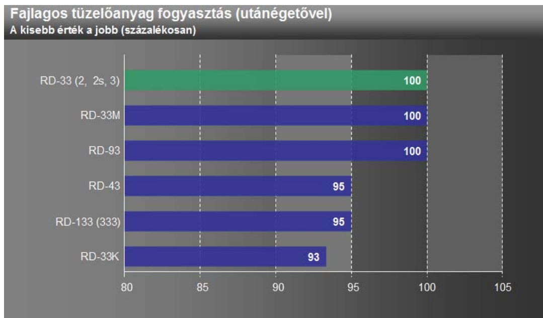
32. ábra: Fajlagos tüzelőanyag fogyasztások a referenciaként jelölt hajtóműhöz viszonyítva. 69
