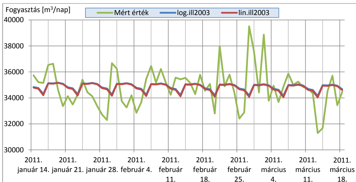
4.2.8-as ábra: Téli időszak becsült és mért fogyasztási értékei
