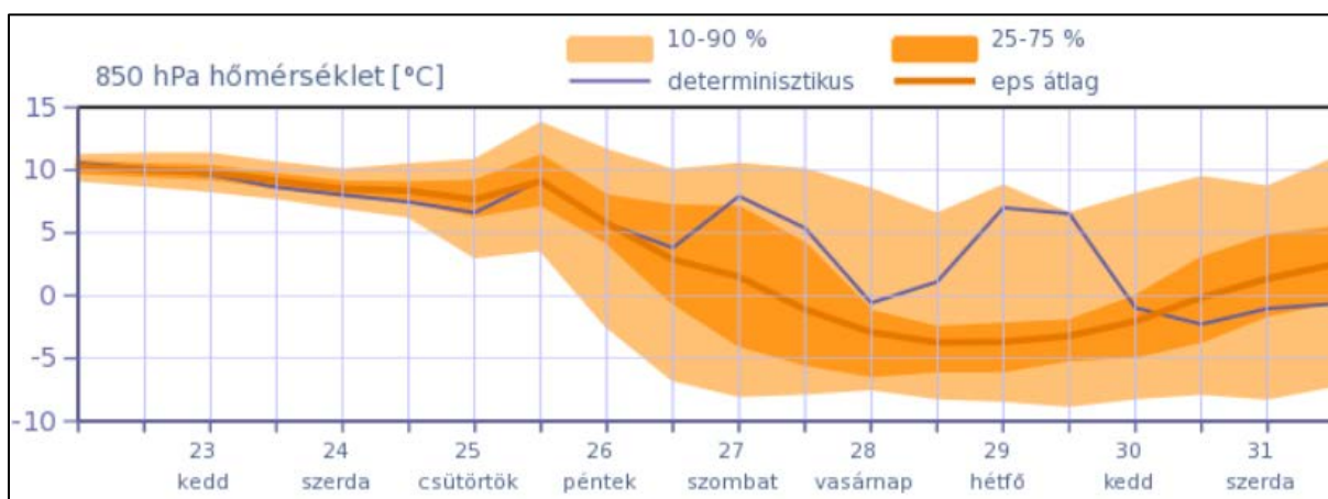
6.1.2-es ábra: Hőmérséklet előrejelzés pontossága (forrás: www.met.hu )
