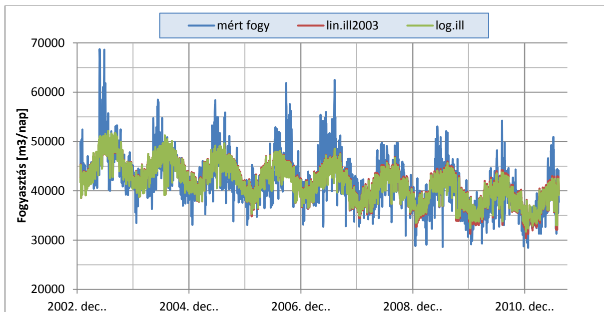
4.2.4-es ábra –2003-tól számított lineáris és logaritmikus regresszió
