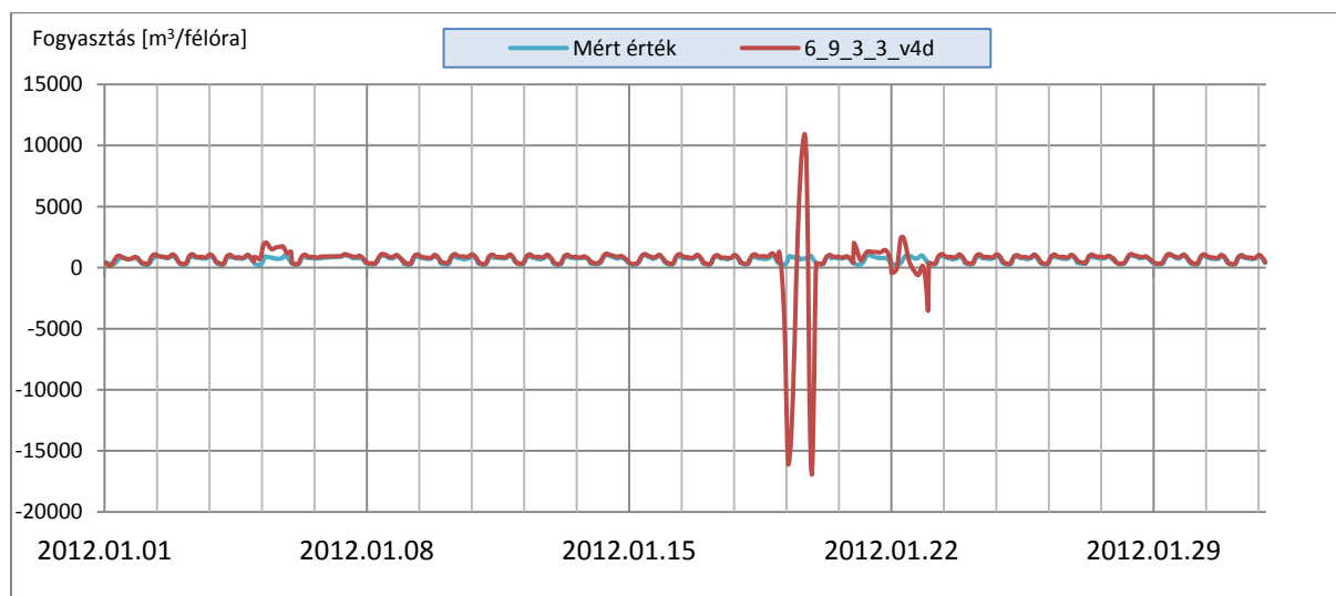
5.5.1-es ábra: Téli független időszak ellenőrzése
