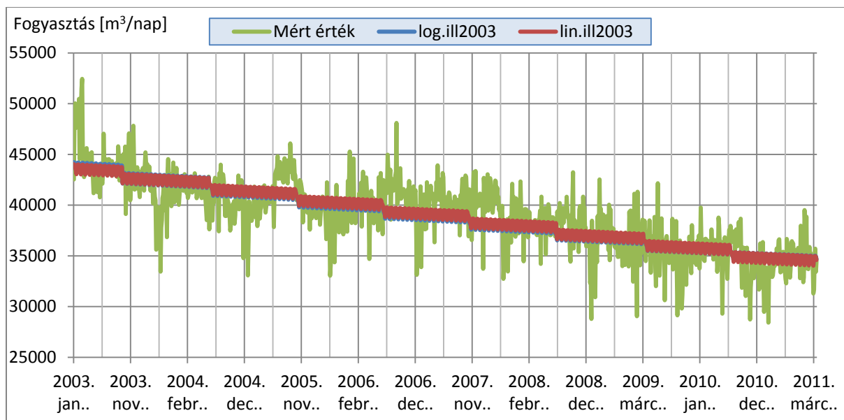
4.2.7-es ábra: Téli időszak becsült és mért fogyasztási értékei
