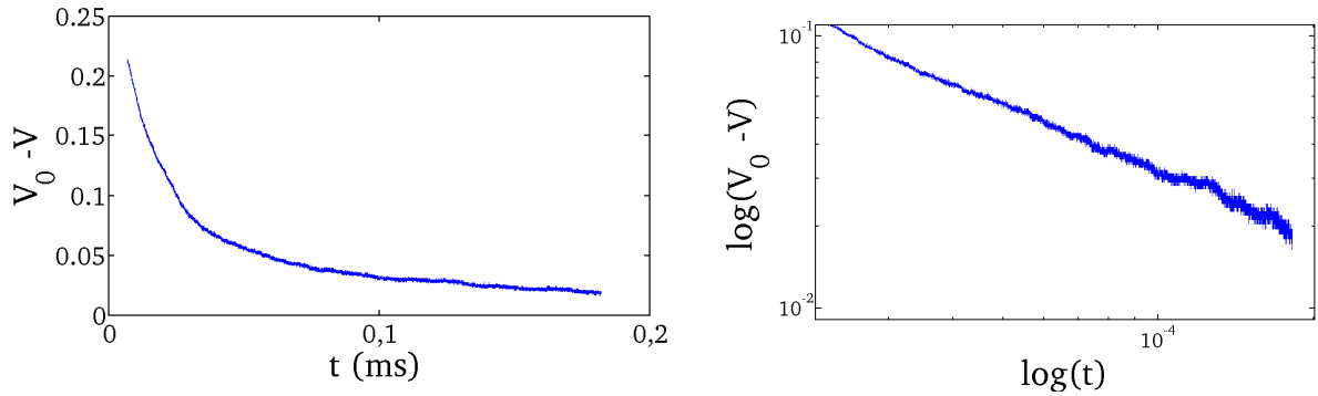
5.9. ábra. Ellentétes irányú kapcsolás relaxációja
