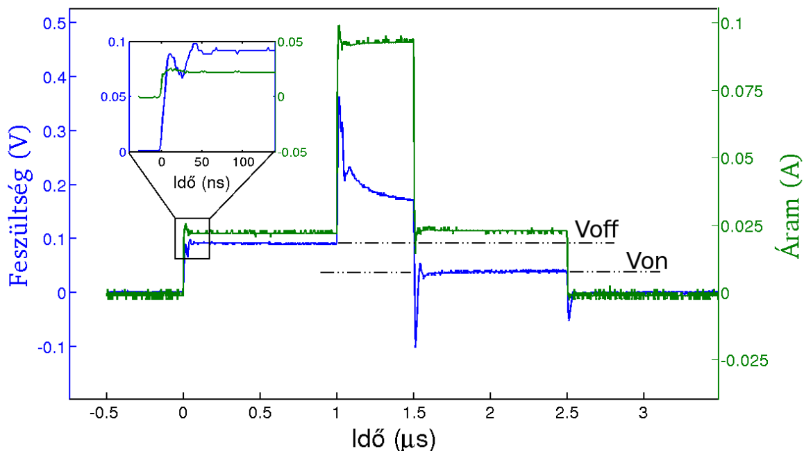
5.5. ábra. Rövid impulzus hatására végbemenő változás, 10 egymás utáni kapcsolás átlaga.
