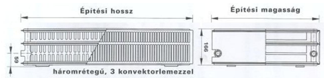
2.1.f. ábra. Három rétegű, három konvektorlemezes lapradiátor.
