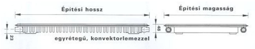
2.1.b. ábra. Egyrétegű, hátfal nélküli, konvektorlemezes lapradiátor.
