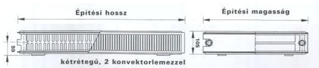
2.1.e. ábra. Kétrétegű, két konvektorlemezes lapradiátor.
