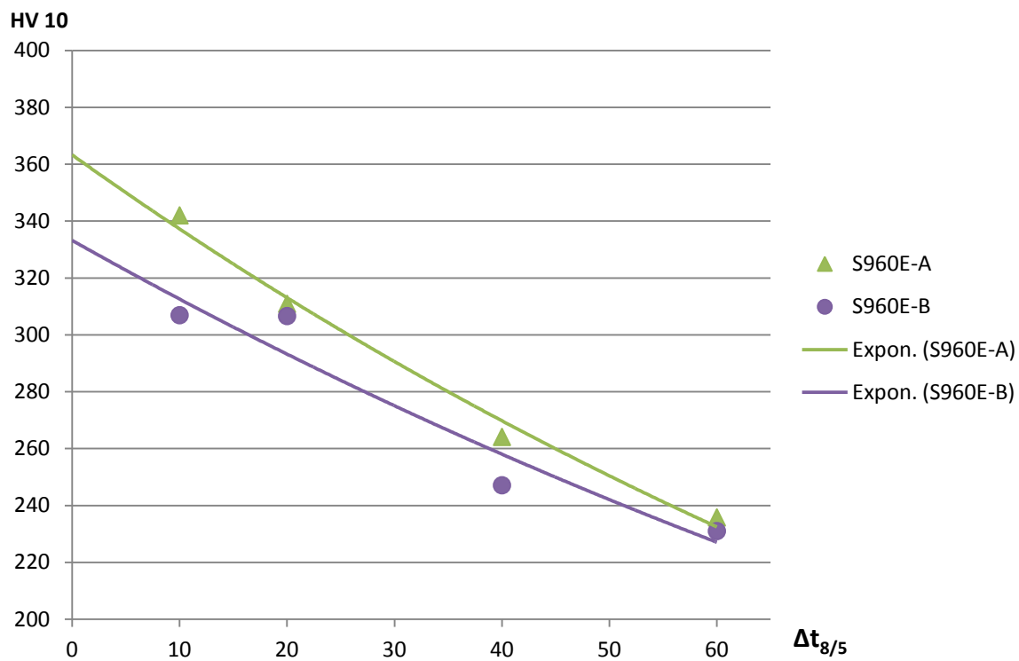
15. ábra Mérési eredmények ábrázolása S960QE anyagra, a keménység a \Delta t_{8/5} függvényében
