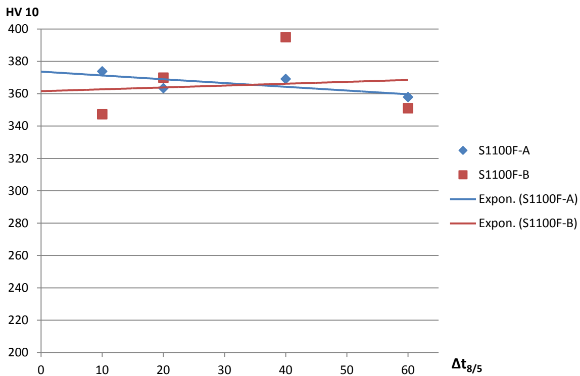
16. ábra Mérési eredmények ábrázolása S1100F anyagra, a keménység a \Delta t_{8/5} függvényében
