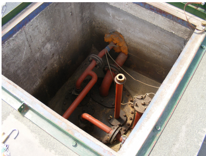
12. ábra a föld alatti tartály teteje
