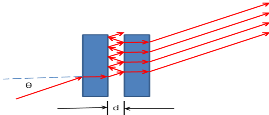
6. ábra: Fabry-Perot interferométer sematikus rajza
