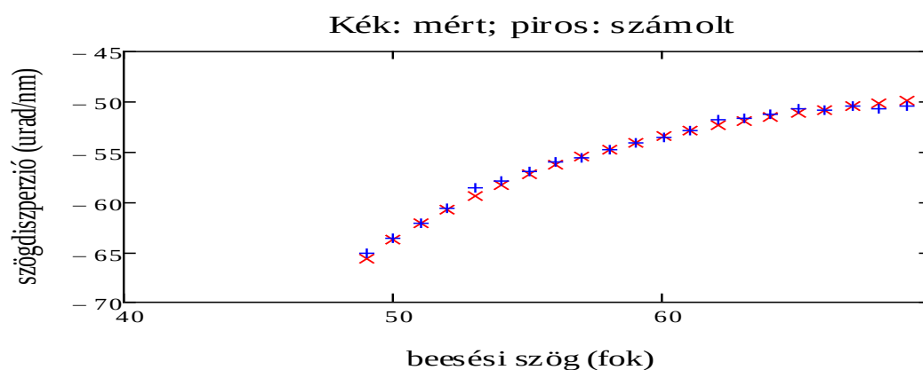
16.ábra Vízszintesen álló prizma szögdiszperziója leképező spektrográffal
