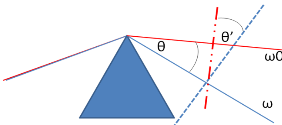
1. ábra: Síkhullámok esetén a két különböző frekvenciához tartozó fázisfront, és terjedési irány által bezárt szög megegyezik
