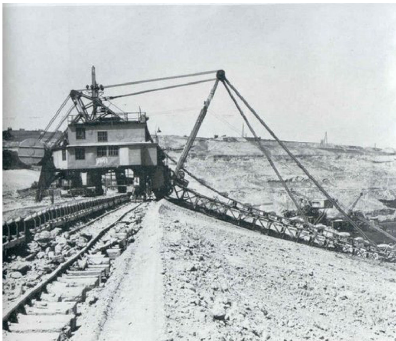
Merítéklétrás kotrógép meddő letakarítása közben az ecsed i külfejtésben (Mátraaljai Szénbányák)
