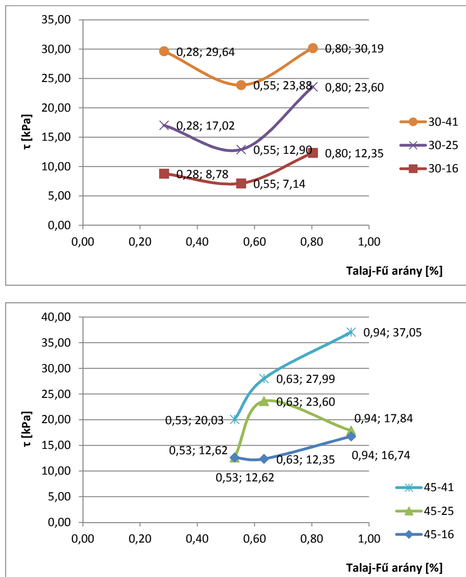
7. ábra Gyökérsűrűség és a feszültség kapcsolata
