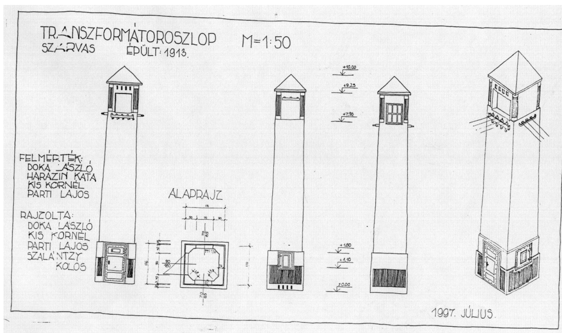
9. Transzformátortorony alaprajz (Felmérték: Doka László, Harazin Kata, Kis Kornél, Parti Lajos. Szarvas, 1997, július)
