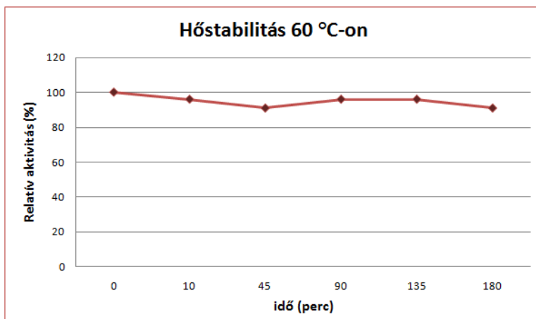
20. ábra - A T. cellulosilytica TB100 törzs Man5A enzimének hőstabilitás mérése 60 °C-on
