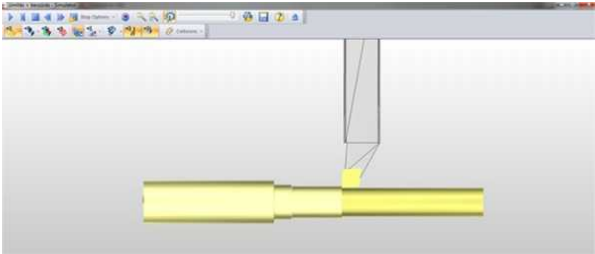
13. ábra. Az „a” felület simító hosszesztergálása.
