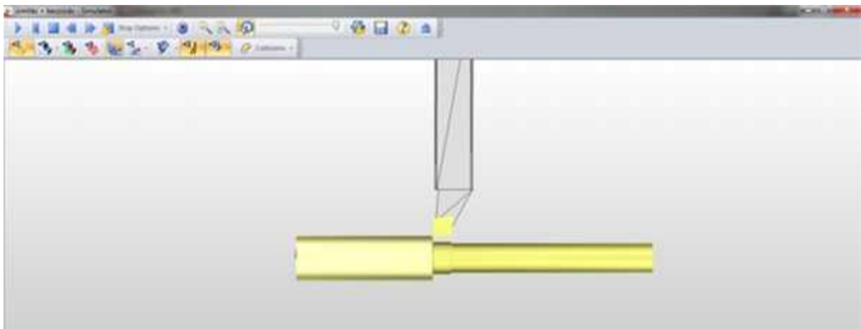
14. ábra. Az „b” felület simító hosszesztergálása.
