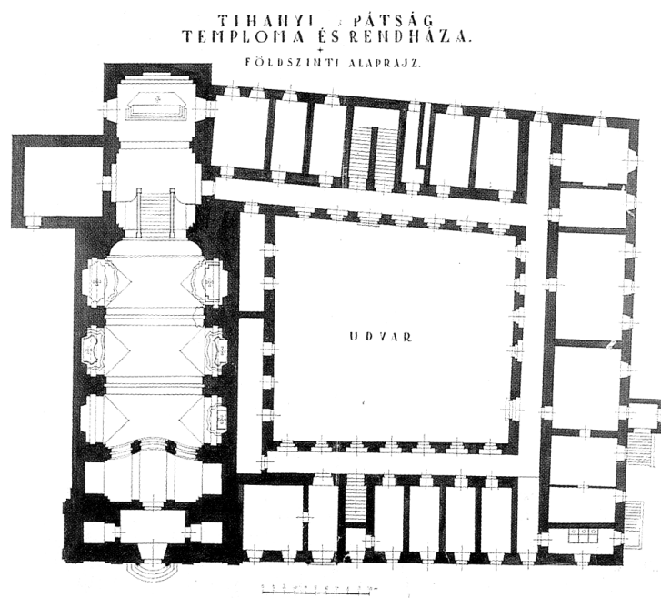
/10.rajz/ Tihany, a templom és a kolostor alaprajza /Budapest, OMvH Tervtár/
