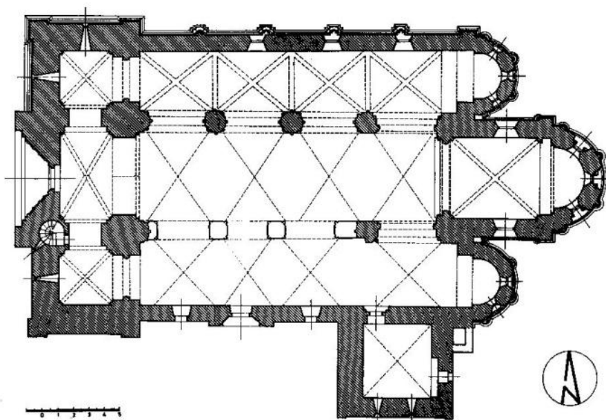
/12.rajz/ Ják , a templom alaprajza
