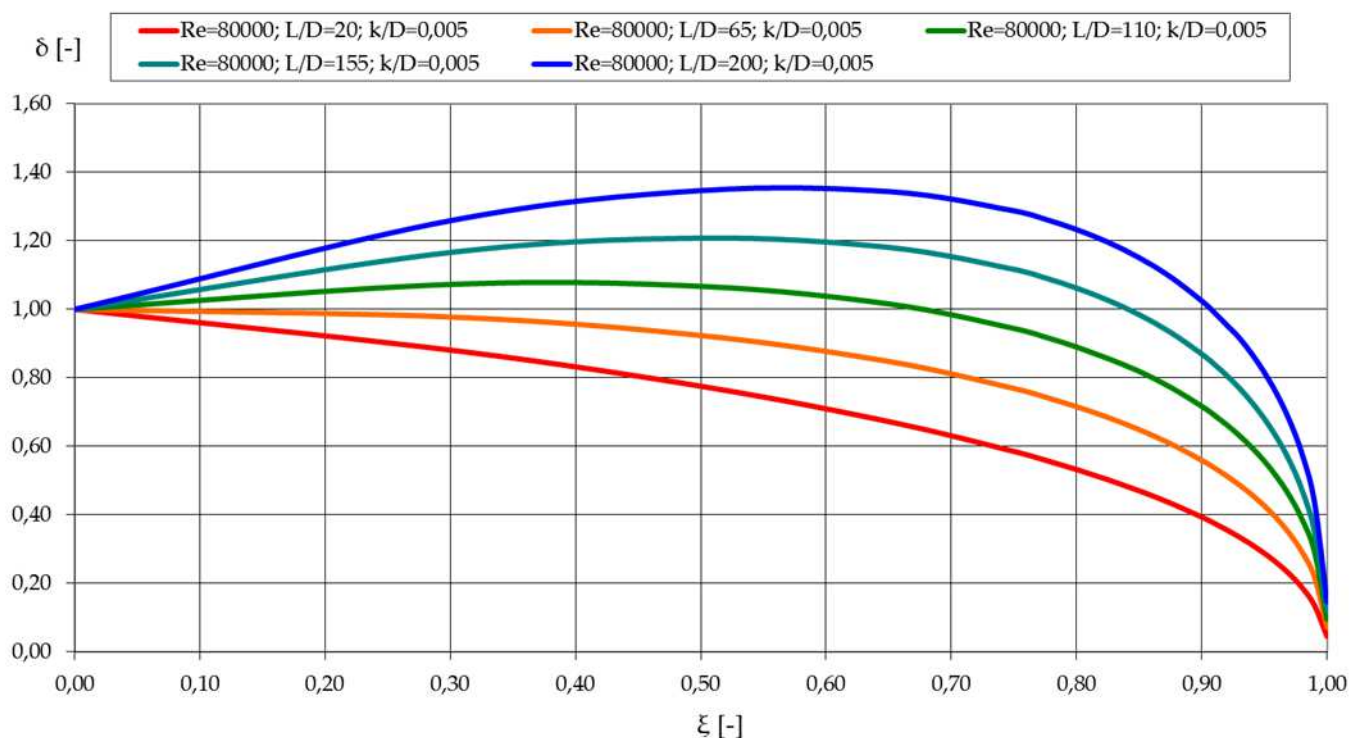
6.14. diagram: A dimenziótlán átmérő változása a dimenziótlán hosszúság függvényében.
