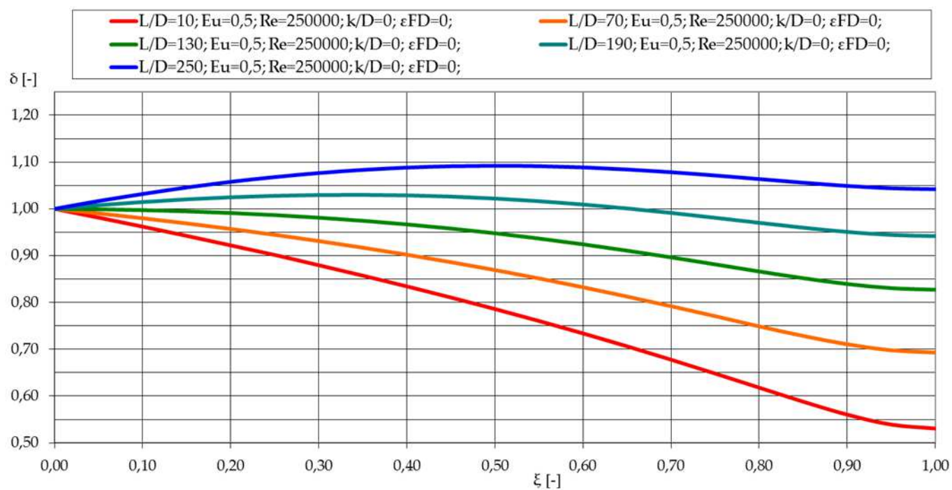
7.19. diagram , A dimenziótlán átmérő változása a dimenziótlán hosszúság függvényében.
