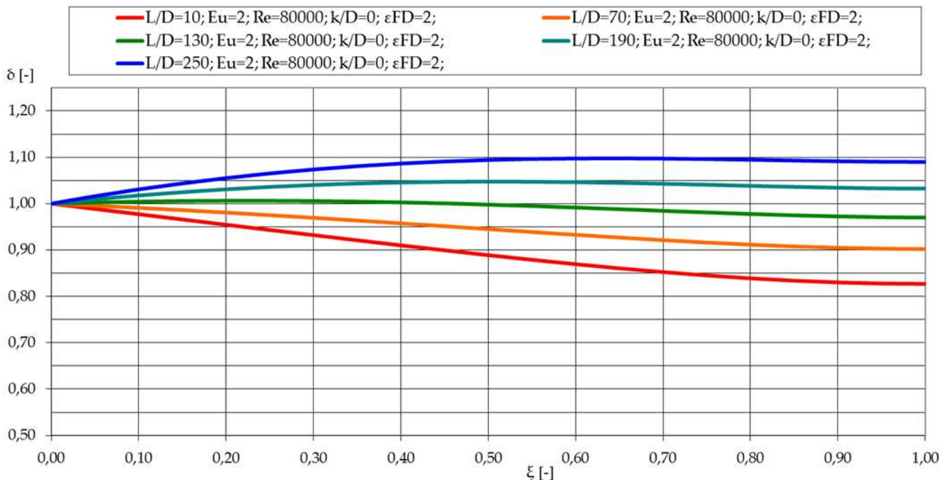
7.16. diagram: A dimenziótlan átmérő változása a dimenziótlan hosszúság függvényében.
