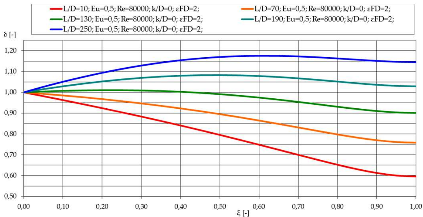
7.18. diagram: A dimenziótlan átmérő változása a dimenziótlan hosszúság függvényében.
