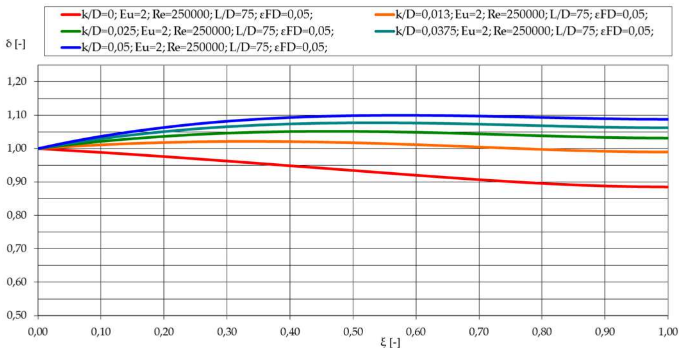
7.26. diagram: A dimenzióatlan átmérő változása a dimenzióatlan hosszúság függvényében.
