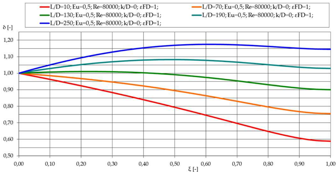
7.17. diagram: A dimenziótlan átmérő változása a dimenziótlan hosszúság függvényében.
