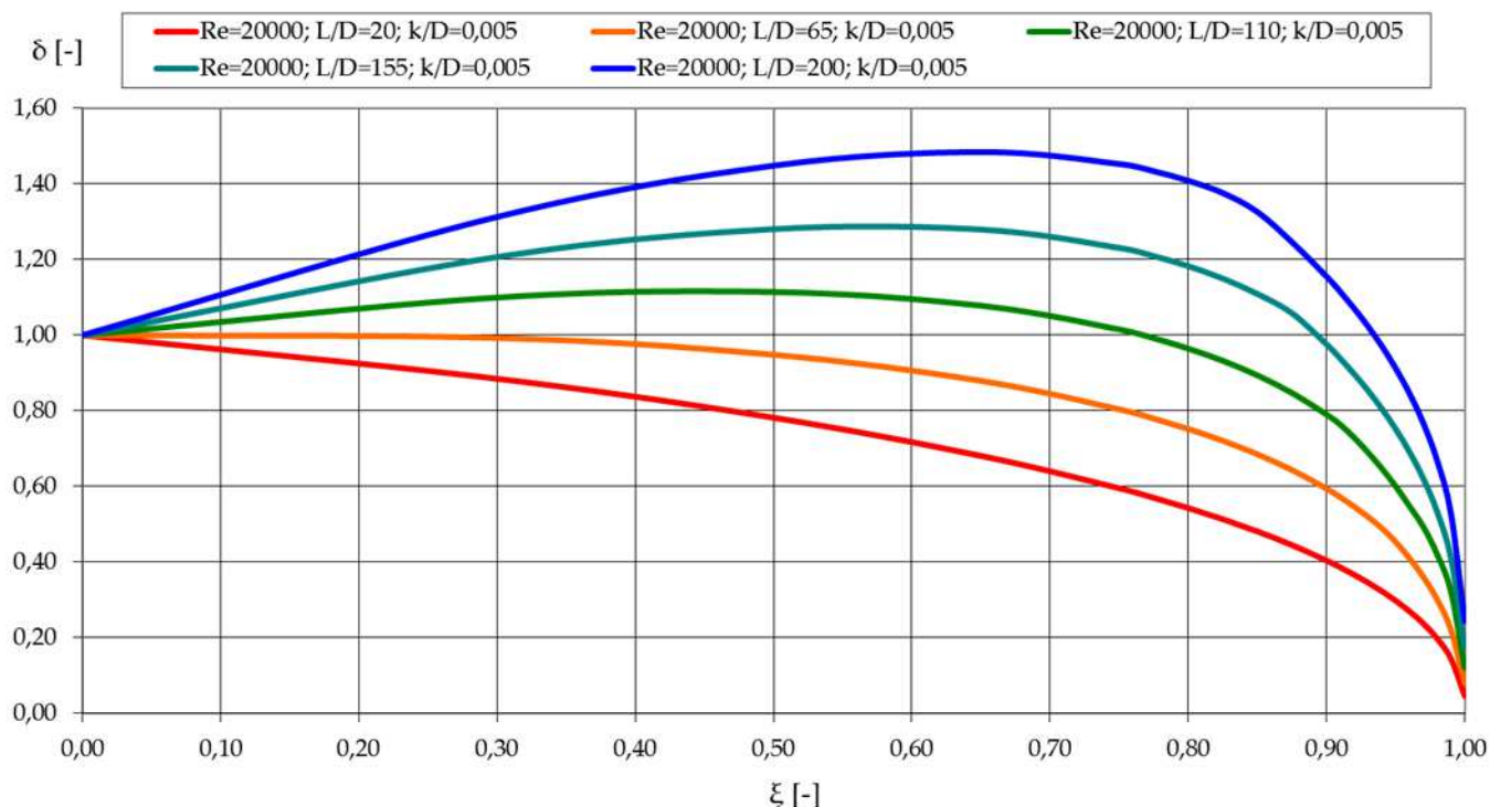
6.13. diagram: A dimenziótlán átmérő változása a dimenziótlán hosszúság függvényében.
