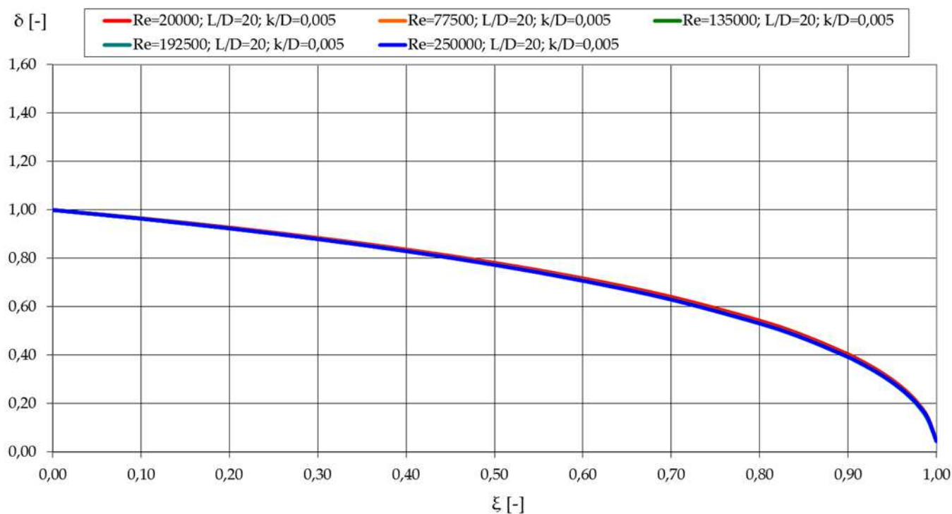
6.4. diagram: A dimenziótlan átmérő változása a dimenziótlan hosszúság függvényében.
