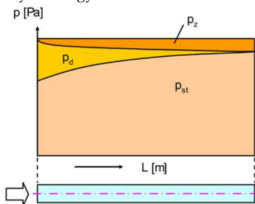
1.3. ábra: A nyomás tipikus változása egy textil légcsatornában, p_z : a veszteségek, p_d : a dinamikus nyomás, p_{st} : a statikus nyomás, [1].
