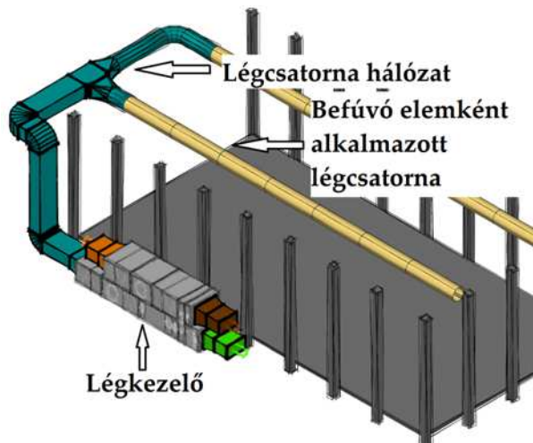
1.1. ábra: Légtechnikai rendszer vázlatos felépítése.
