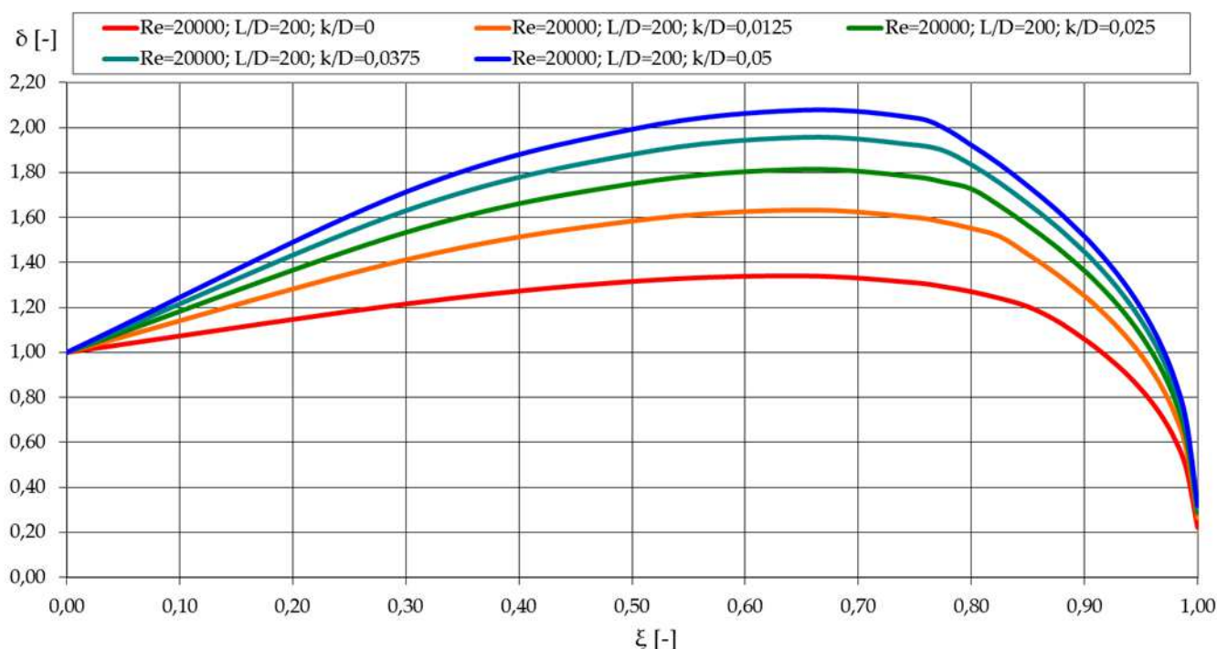
6.8. diagram: A dimenziótlan átmérő változása a dimenziótlan hosszúság függvényében.
