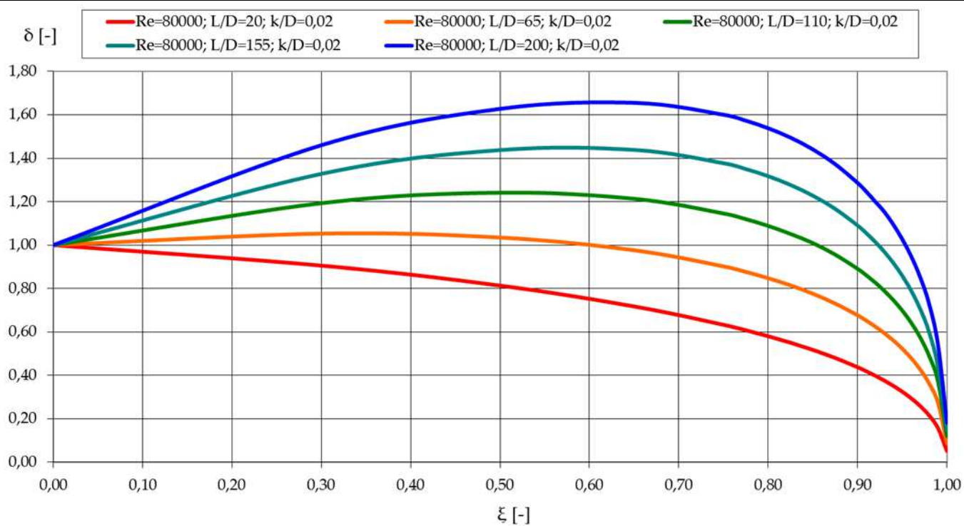
6.19. diagram: A dimenziótlán átmérő változása a dimenziótlán hosszúság függvényében.
