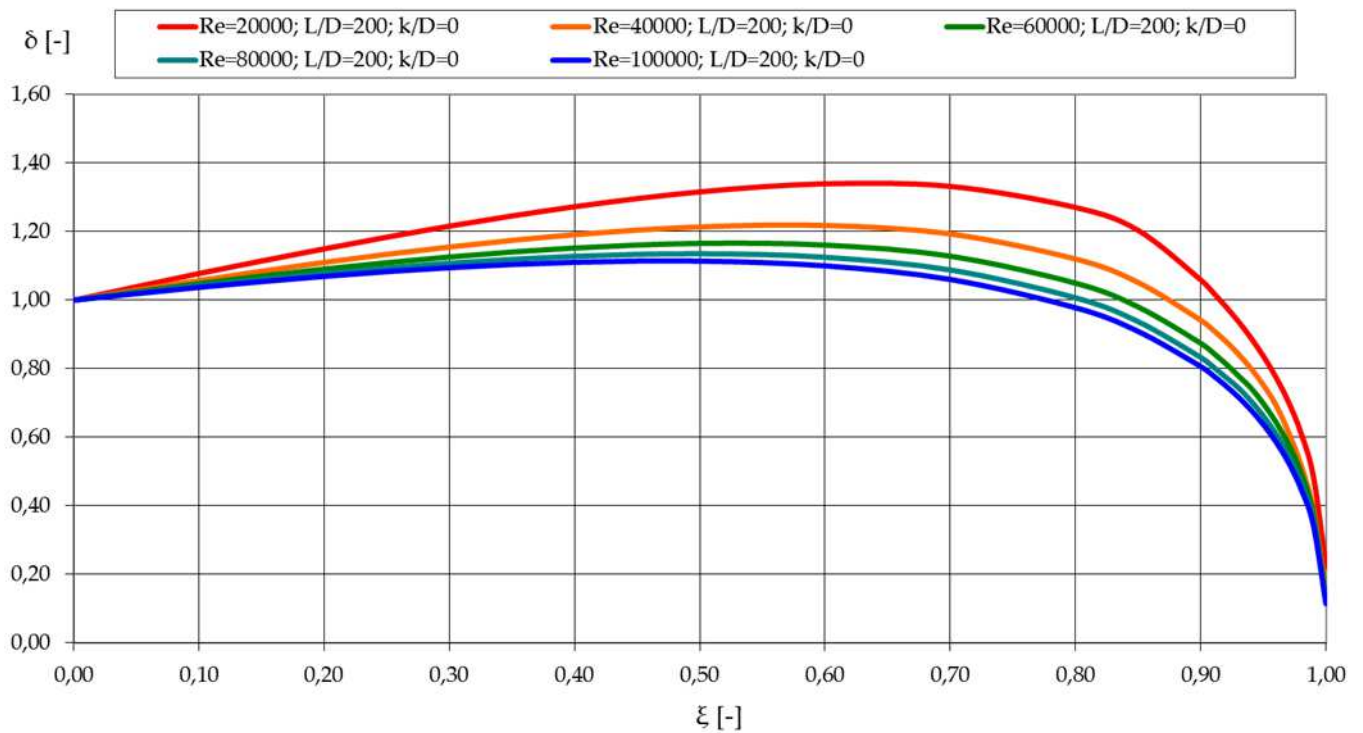
6.3. diagram: A dimenziótlan átmérő változása a dimenziótlan hosszúság függvényében.
