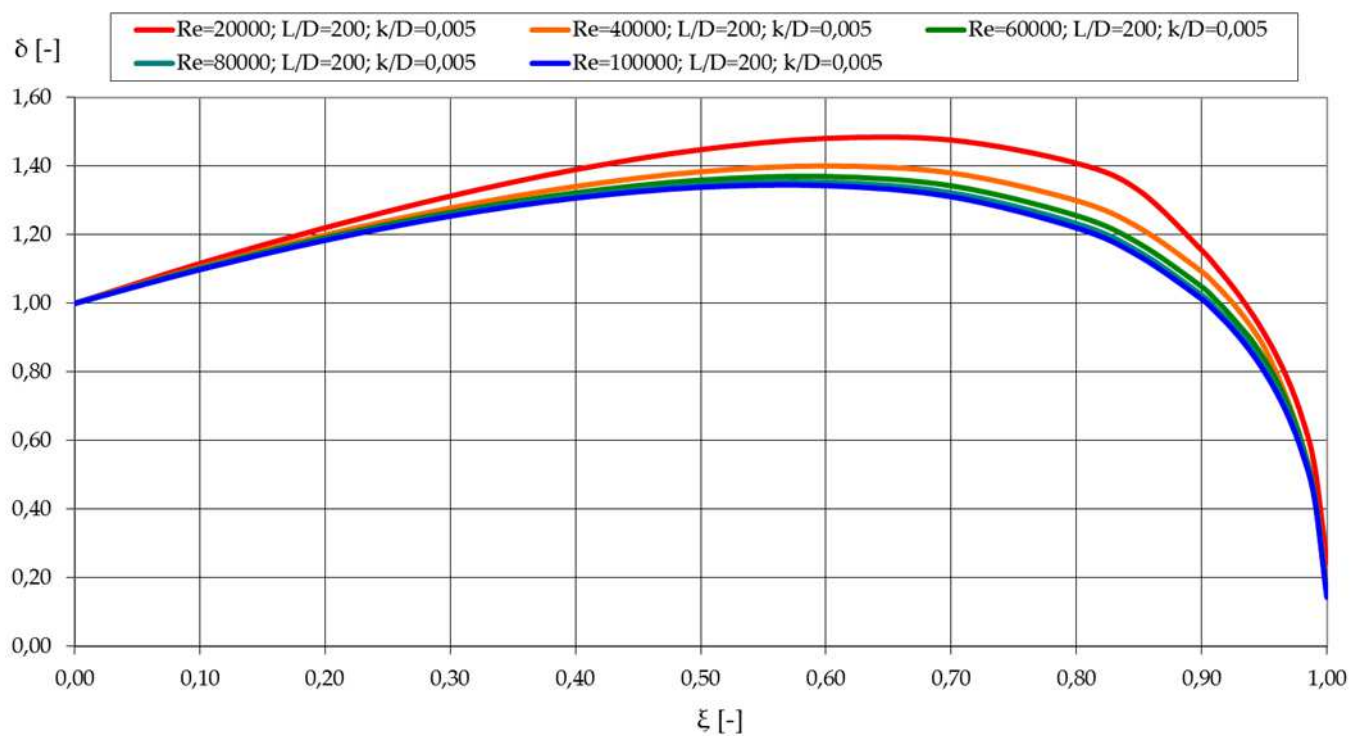
6.6. diagram: A dimenziótlan átmérő változása a dimenziótlan hosszúság függvényében.
