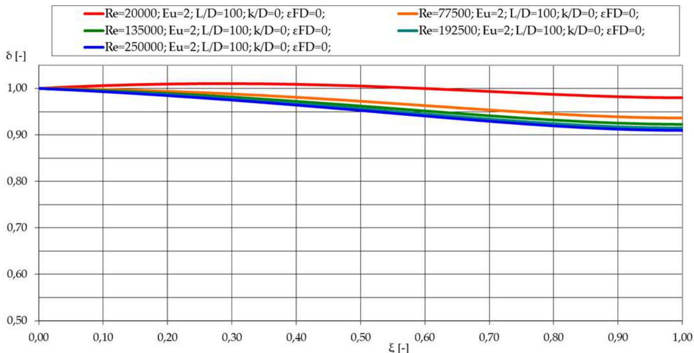
7.11. diagram: A dimenzióatlan átmérő változása a dimenzióatlan hosszúság függvényében.
