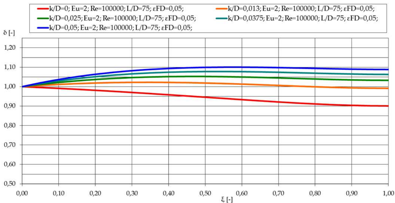
7.24. diagram: A dimenzióatlan átmérő változása a dimenzióatlan hosszúság függvényében.
