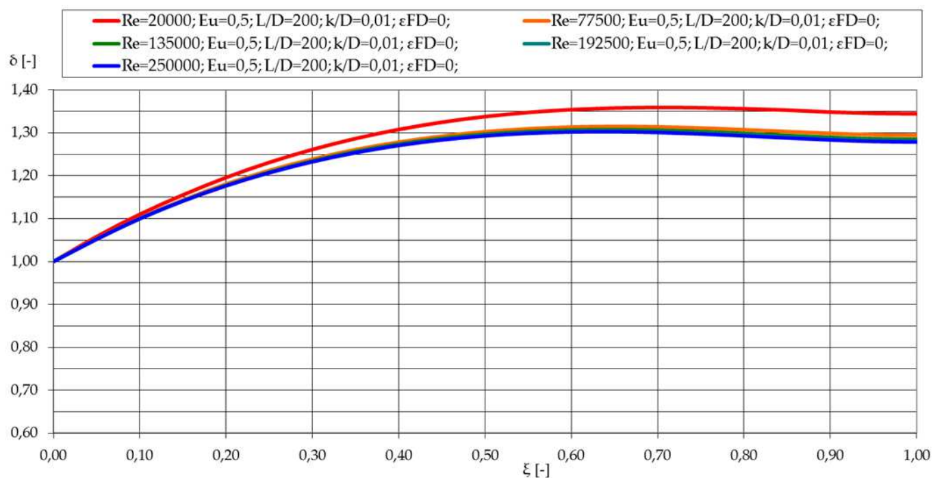
7.14. diagram: A dimenziótlan átmérő változása a dimenziótlan hosszúság függvényében.
