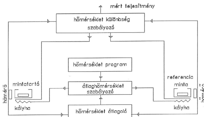
10. ábra A teljesítménykompenzációs DSC visszacsatoló rendszere [11]
