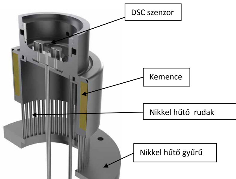
15. ábra Heat flow típusú DSC (Q2000, TA instruments) [9]
