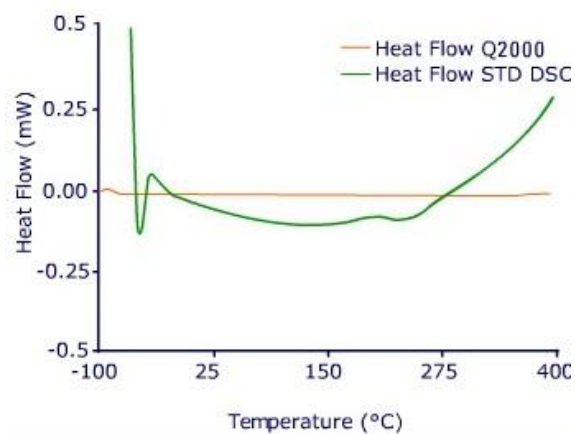
12. ábra Az alapvonal sokkal laposabb a Tzero™-val felszerelt Q2000 típusú DSC-vel (TA instruments) való mérésnél [9]
