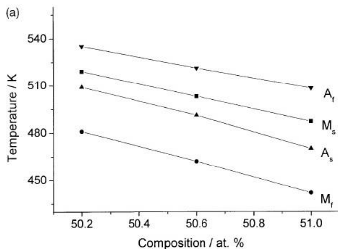
6. ábra Három különböző TiNiPd ötvözet átalakulási hőmérsékletei a Ti-tartalom függvényében
