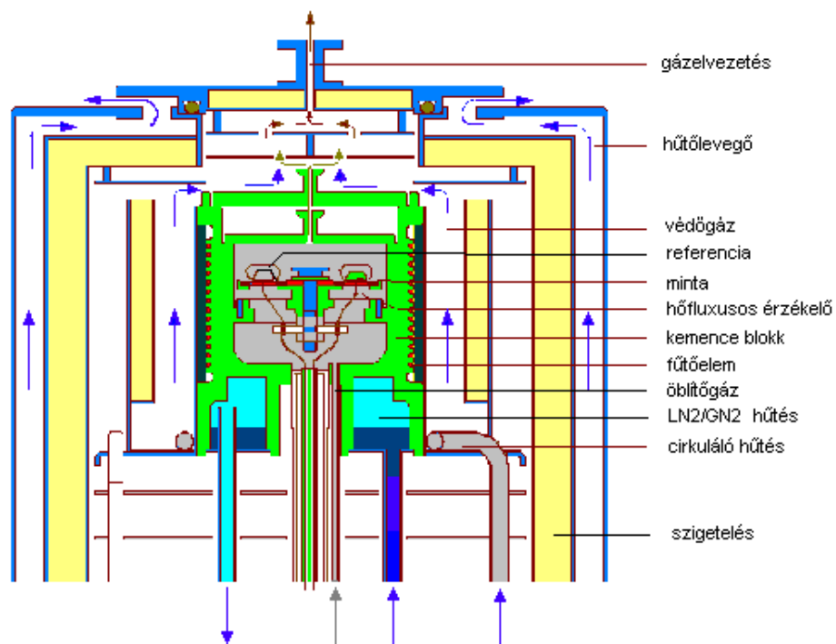
16. ábra Egy Netsch 204 típusú DSC berendezés sematikus vázlatja [15]
