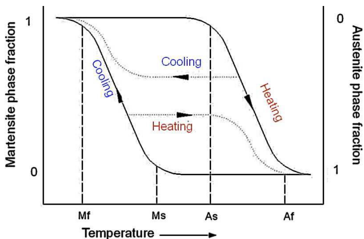
26. ábra Hiszterézis görbék [3]
