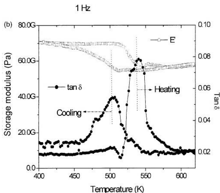
22. ábra Ti 51 Pd 30 Ni 19 ötvözet DMA görbéje [22]
