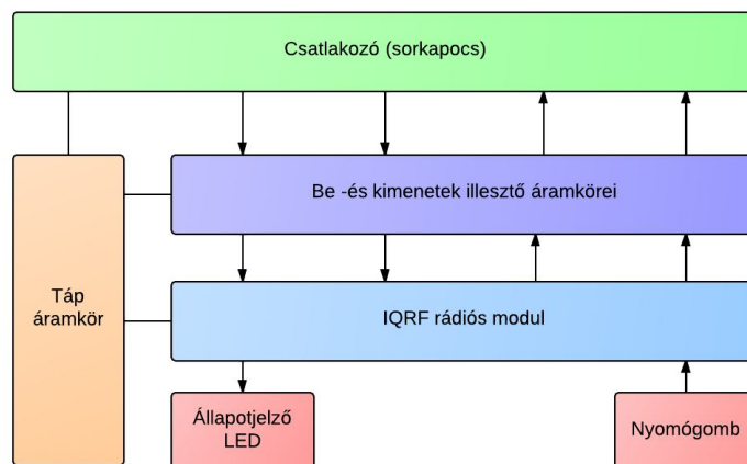
17. ábra Vezérlő eszközök felépítése
