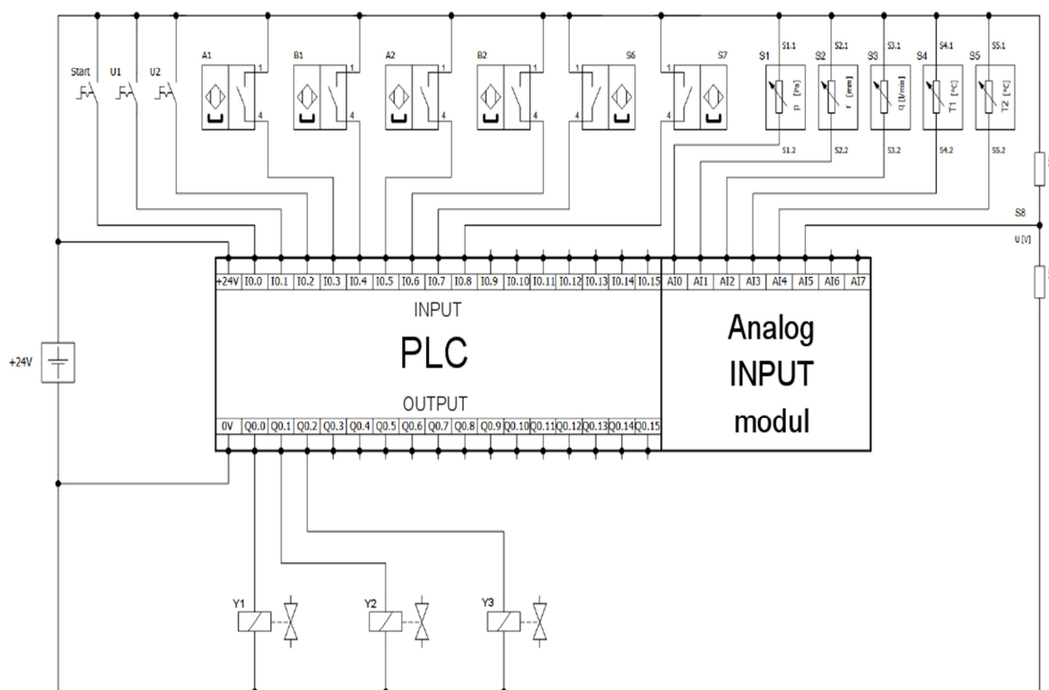
21. ábra: A járműn elhelyezett mérésadatgyűjtő és vezérlő kapcsolási rajza
