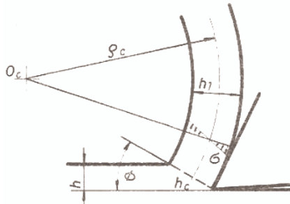
18. ábra: Forgáctörés mechanizmusa
