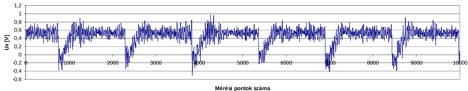
11. sz. mérés feszültséggörbéje az Y tengely mentén
