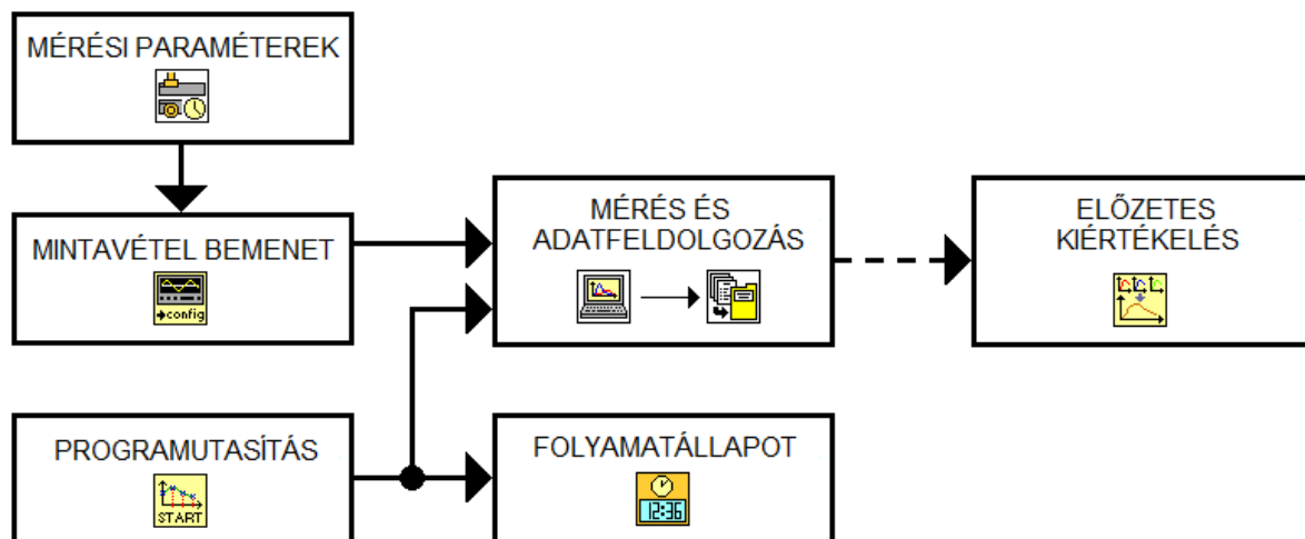
14. ábra: Főprogram blokkdiagram
