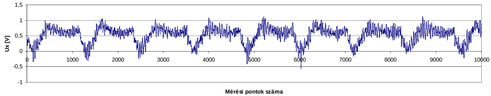
9. sz. mérés feszültséggörbéje az Y tengely mentén
