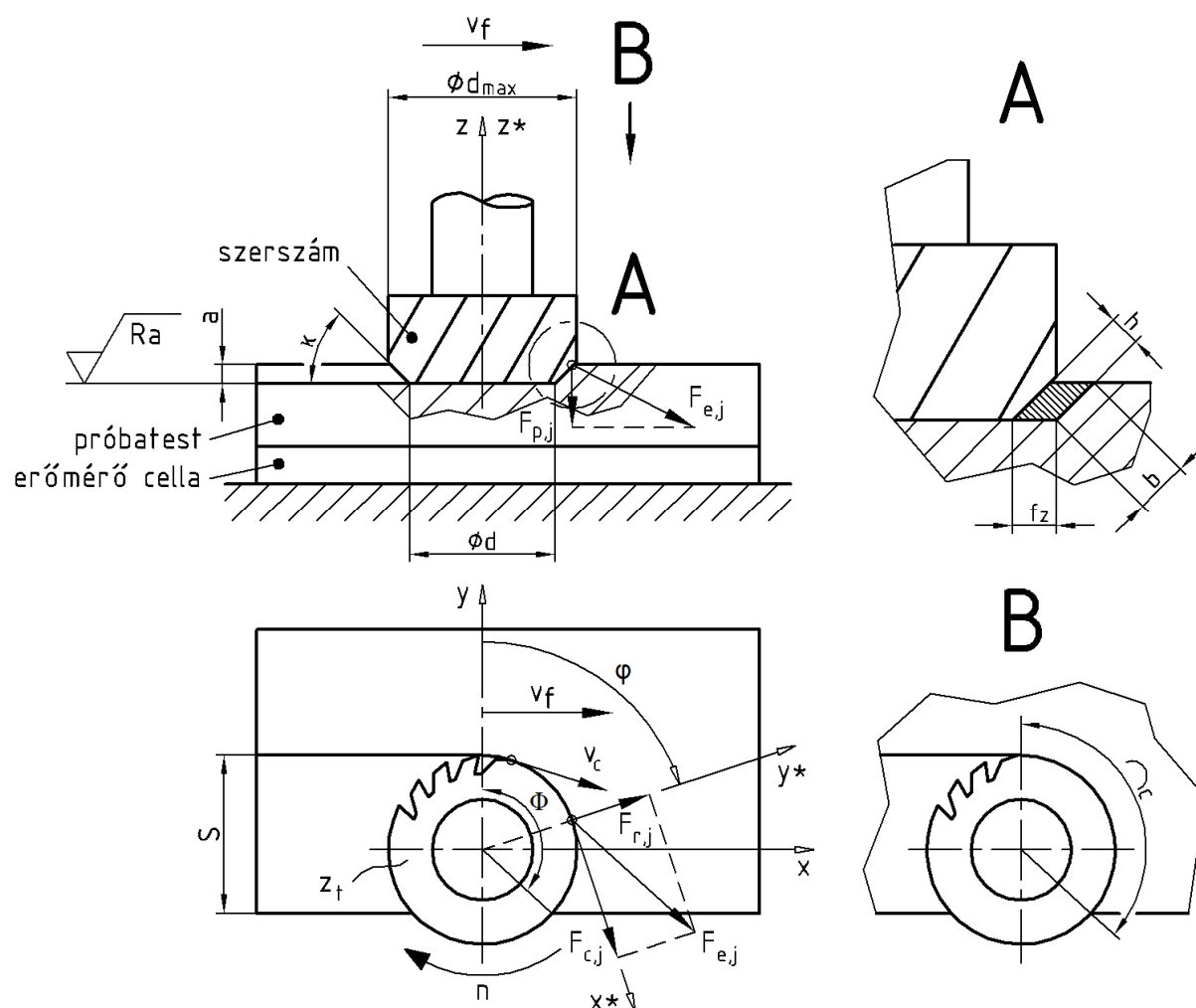
2. ábra: A programhoz tartozó mérési összeállítás vázlata
