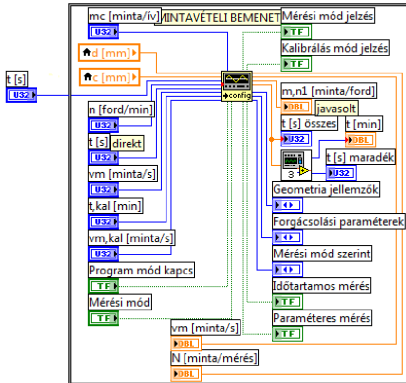
16. ábra: Mintavételi bemenet blokk
