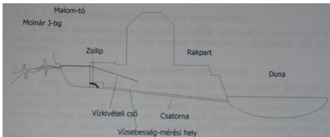
15. ábra: Sematikus ábra a Lukács-fürdő alatti csatornáról (Mádlné et al., 2001).
