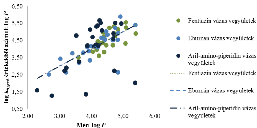
log k_{0,grad} értékekből számolt log P - Potenciometrikusan mért log P értékek korrelációja Lokális, pH 2,6
