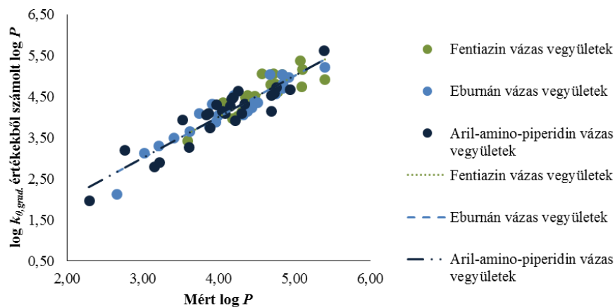
log k_{0,grad} értékekből számolt log P - Potenciometrikusan mért log P értékek korrelációja Lokális, pH 10,8
