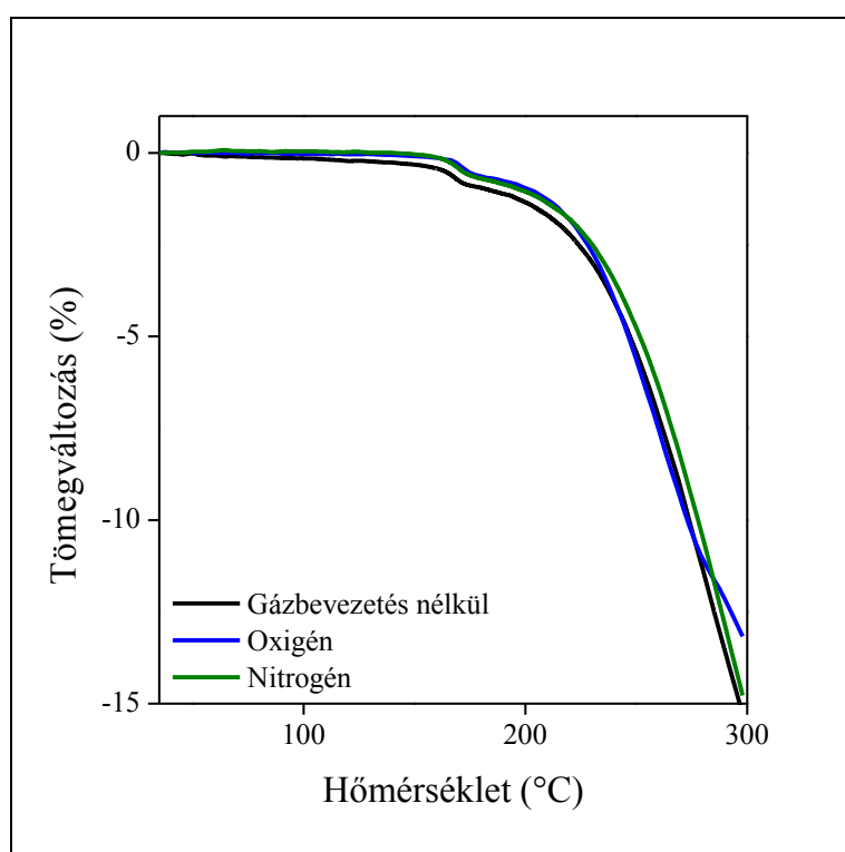
23. ábra: A kurkumin TG görbéi gázbevezetés nélkül, oxigén és nitrogén áramban, 3.5 °C/min fűtési sebességgel
