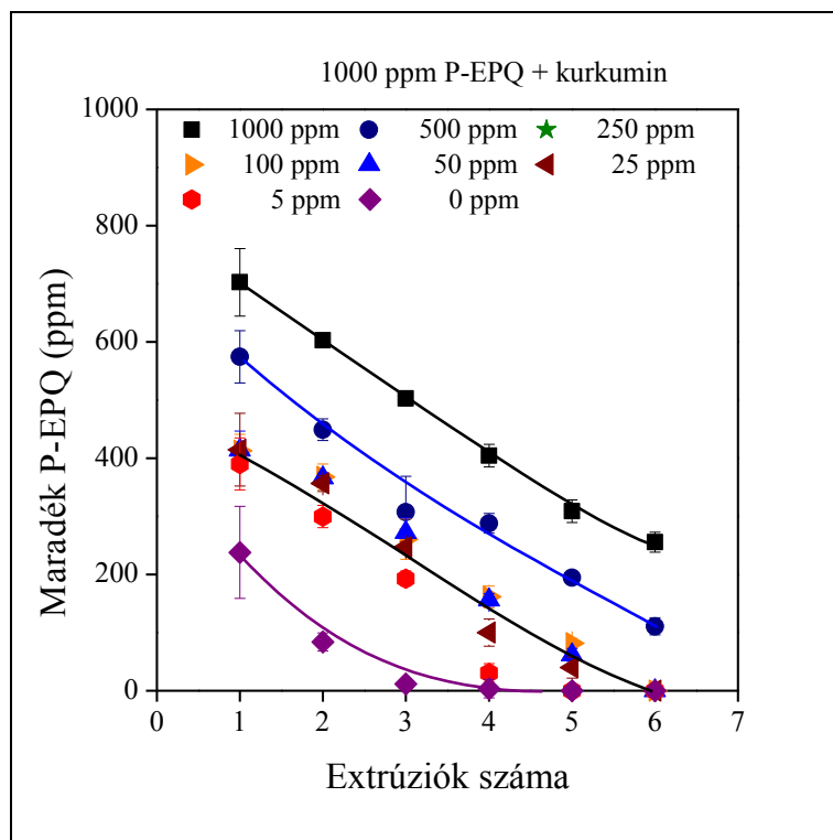
9. ábra A kurkumin mennyiségének hatása a P-EPQ fogyására a polimer többszöri extrúziója során
