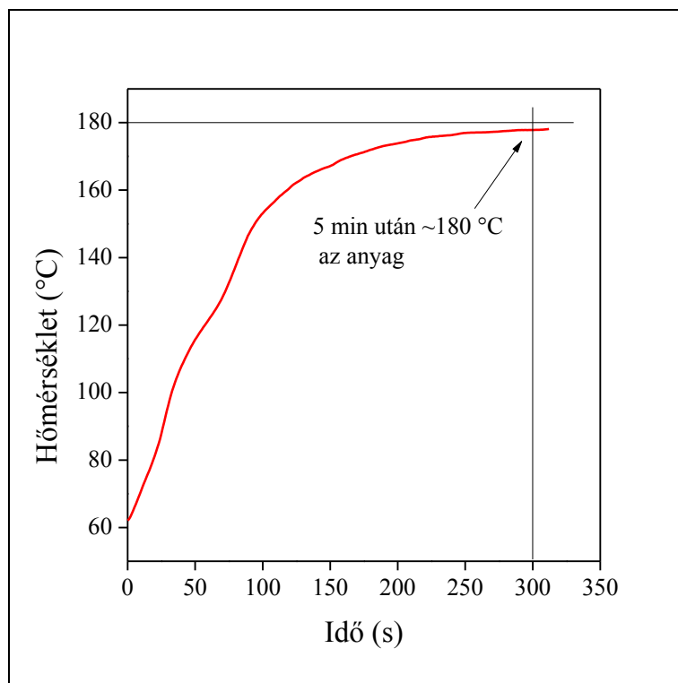
2. ábra: 1 g P-EPQ termoelemmel mért hőmérsékletváltozása 200 °C hőmérsékletű olajba merített gömblombikban
