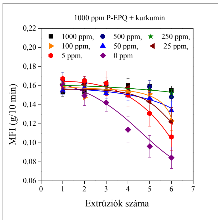
7. ábra: A folyókéesség változása a többszöri extrúzió során, 1. sorozat
