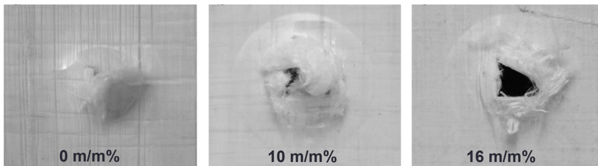
27. ábra: SR PLA és égésálló SR PLA kompozitok ejtésúlyos vizsgálata után készült fotók
