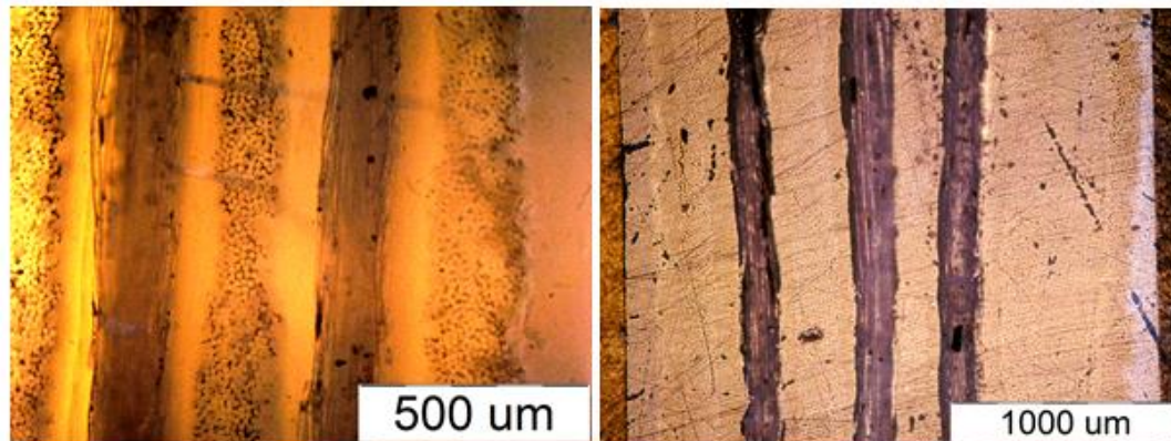
18. ábra: SR referencia kompozit keresztmetszetéről készült optikai mikroszkópos képek
