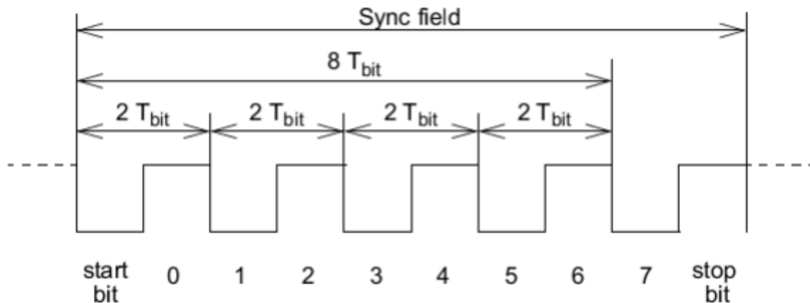
10. ábra: LIN szinkronizációs mező
