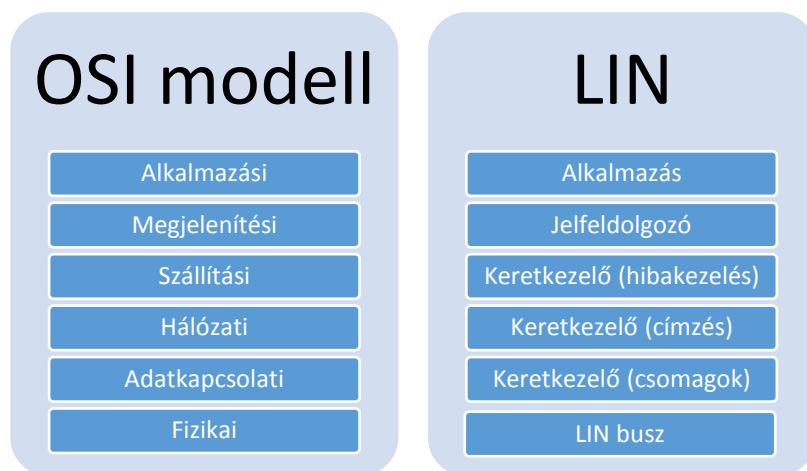
5. ábra: A LIN hálózat rétegei
