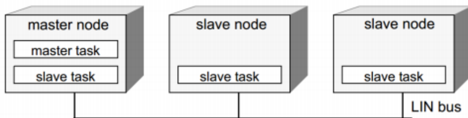
6. ábra: A LIN hálózat logikai felépítése
