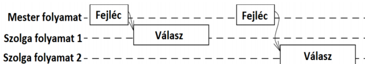
8. ábra: LIN kommunikáció vázlata
