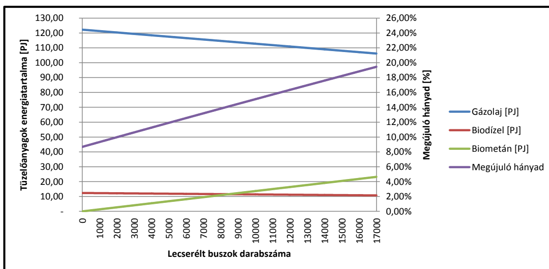
11. ábra: A változó energiamennyiségek és a megújuló hányad alakulása városi buszok lecserélése esetén – optimista változat
