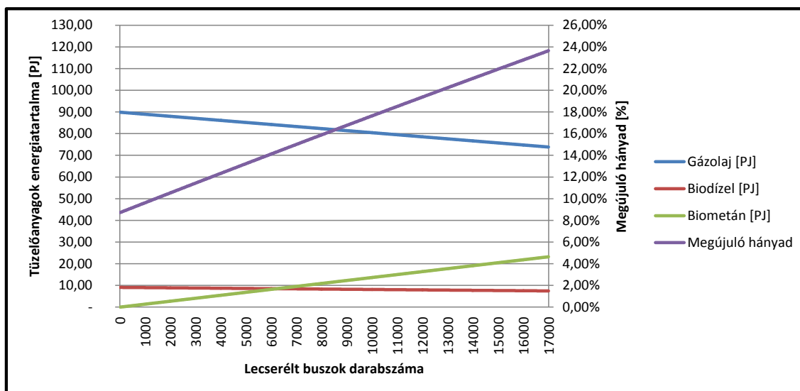
12. ábra: A változó energiamennyiségek és a megújuló hányad alakulása városi buszok lecserélése esetén – pesszimista változat
