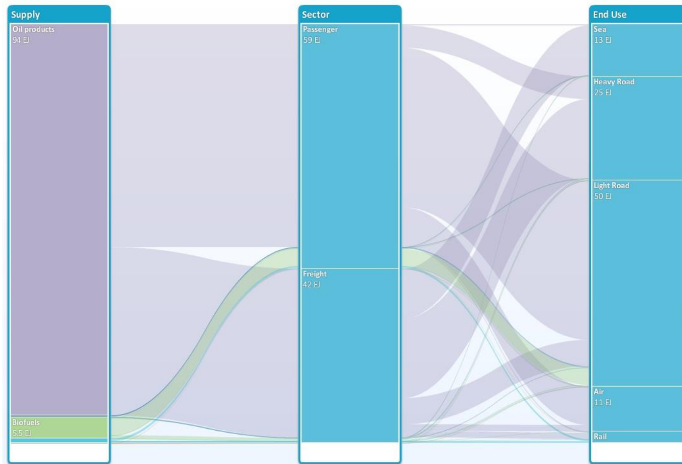
6. ábra: Közlekedésben felhasznált energiamennyiségek várható alakulása globálisan, 2020-ban
