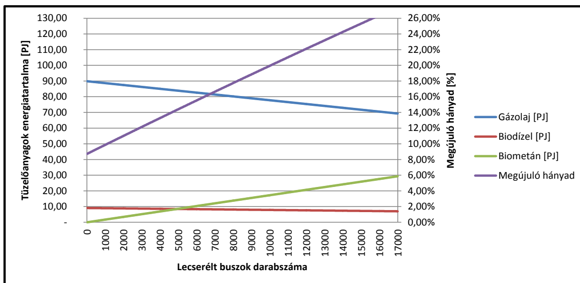
14. ábra: A változó energiamennyiségek és a megújuló hányad alakulása távolsági buszok lecserélése esetén – pesszimista változat
