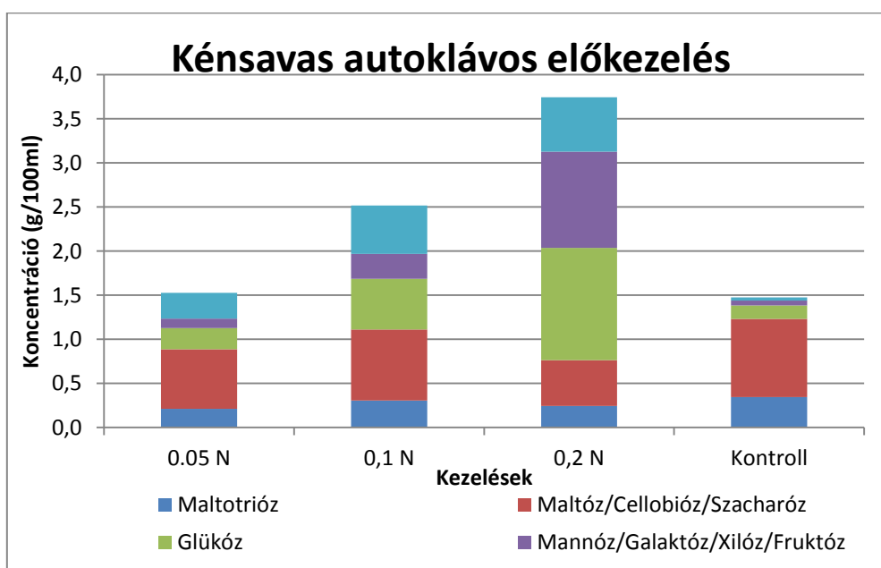
8. ábra: Kénsavas autoklávós előkezelések szénhidrát koncentrációi az enzimes hidrolízis előtt
