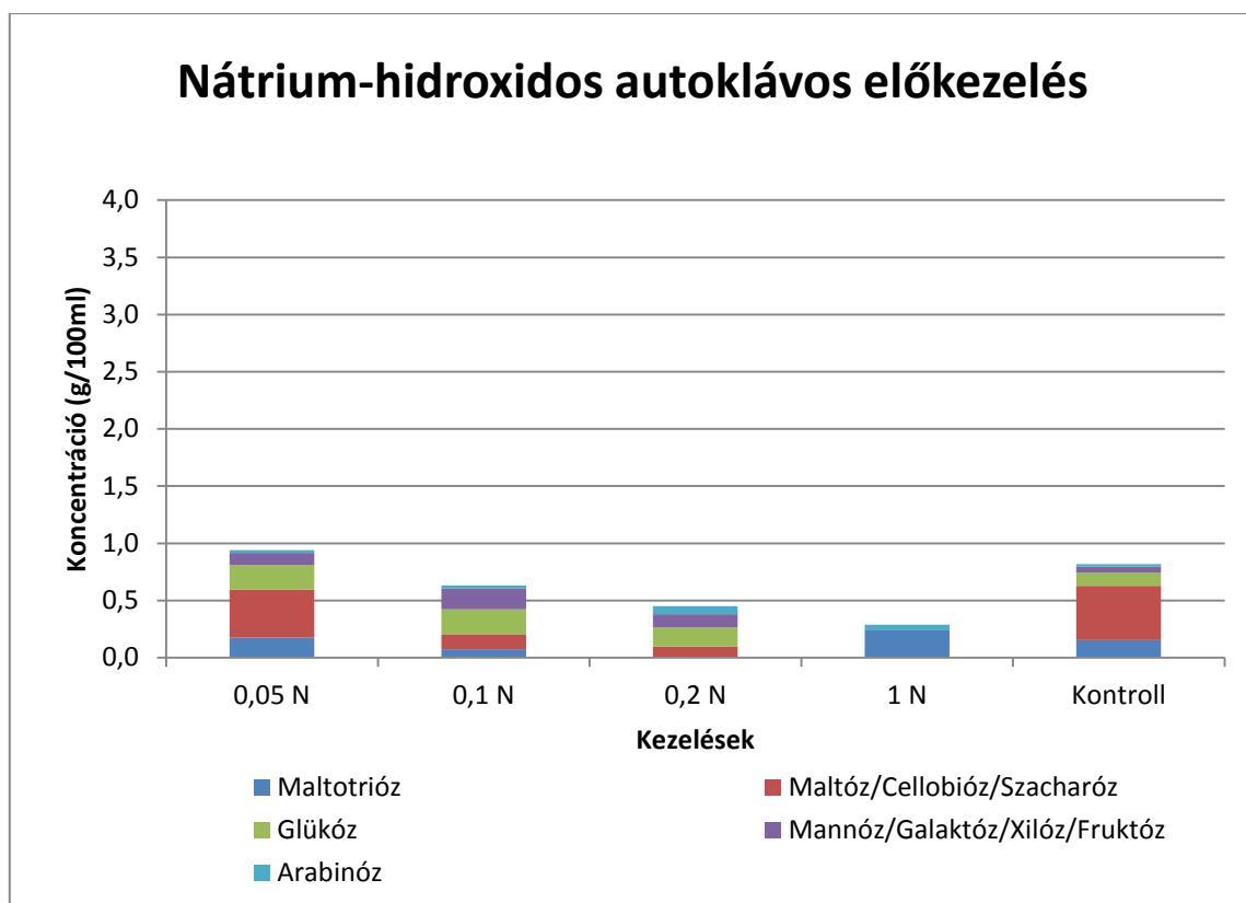
10. ábra: Nátrium-hidroxidos autoklávós előkezelések szénhidrát koncentrációi az enzim hidrolízis előtt
