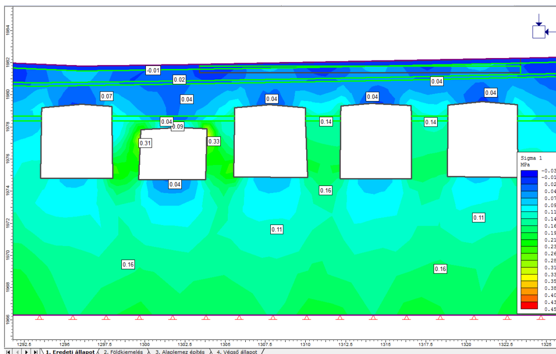
20. ábra. A \sigma_1 feszültség eredeti állapotban
