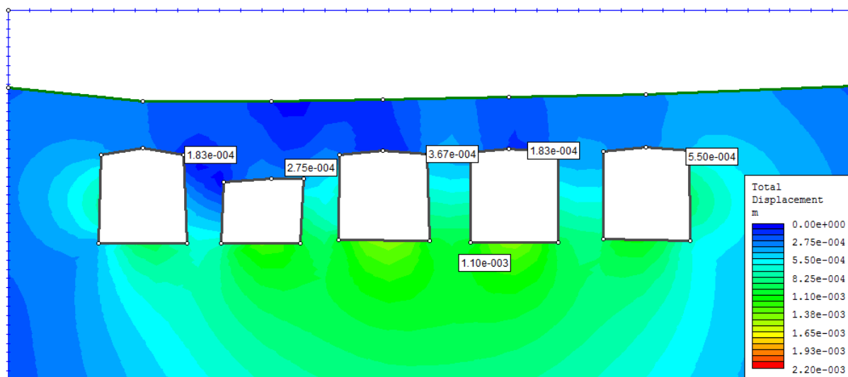
12. ábra. Az elmozdulások alakulása eredeti állapotban
