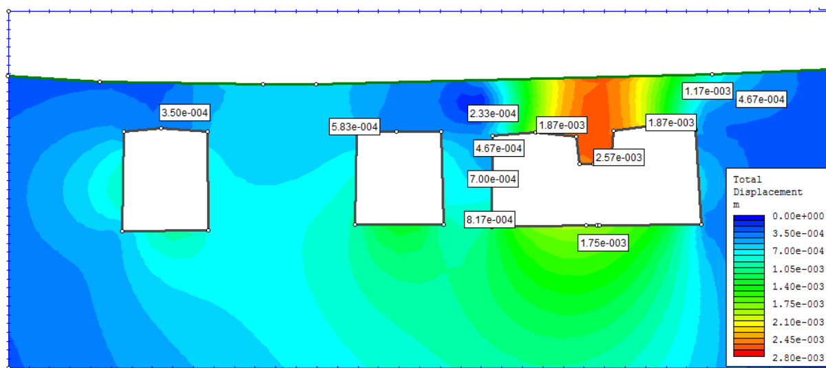
16. ábra. Az elmozdulások alakulása eredeti állapotban
