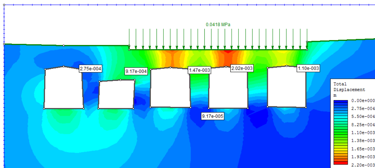
13. ábra. Az elmozdulások alakulása végleges állapotban
