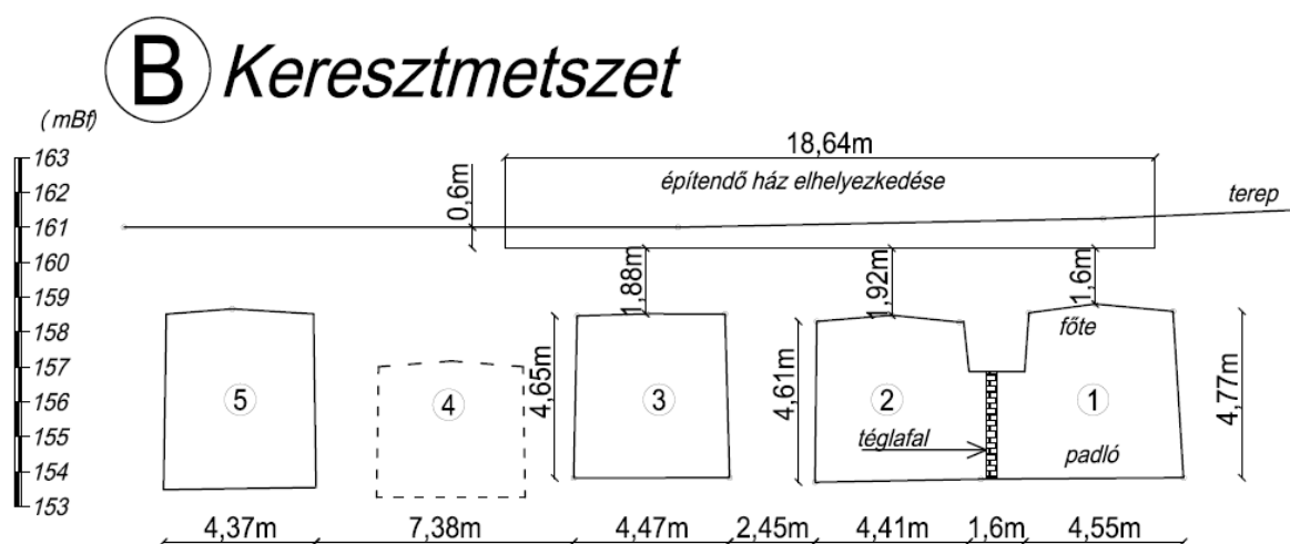
5. ábra. A B keresztmetszet
