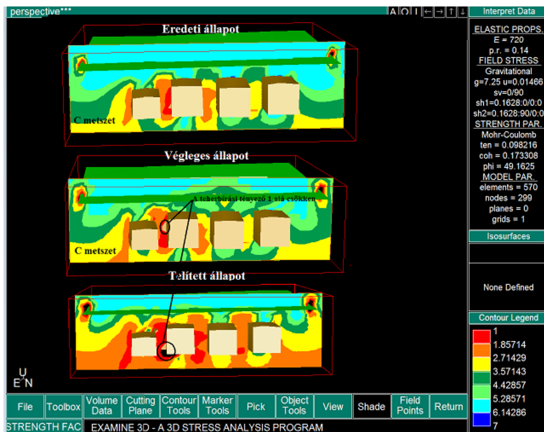
37. ábra. A teherbírési tényező változása a különböző állapotokban
