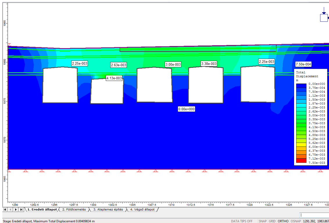
24. ábra. Az elmozdulások eredeti állapotban
