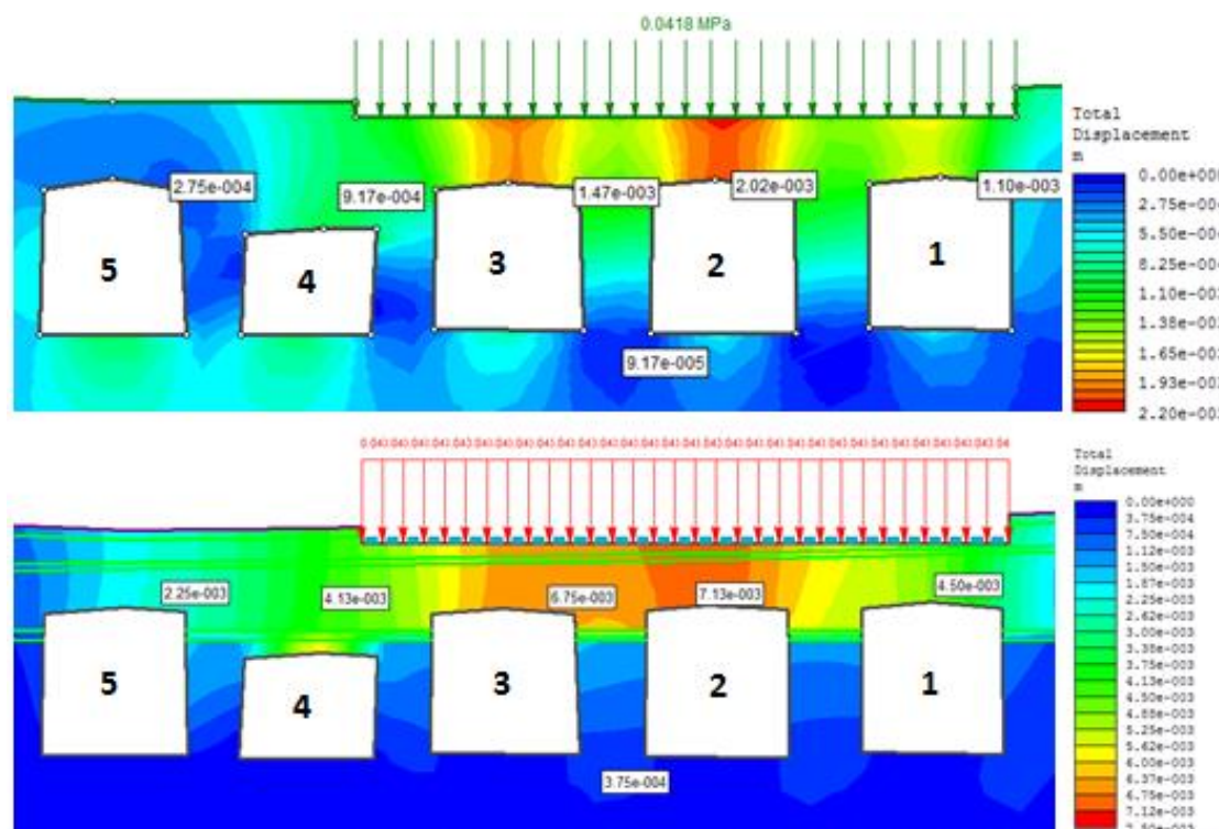
51.ábra. Az elmozdulások összehasonlítása végleges állapotban (C km)
