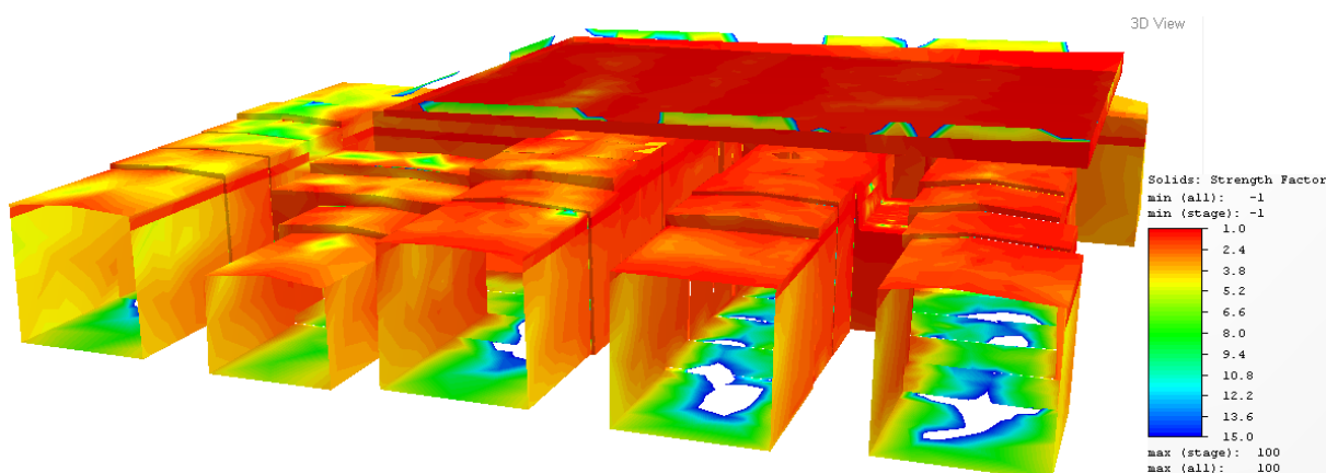
44. ábra. Az teherbírási tényező alakulása végső állapotban
