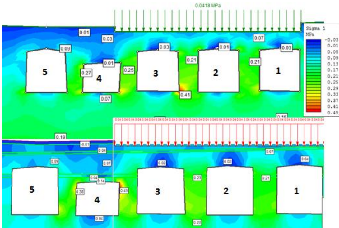
48.ábra. Az feszültségek összehasonlítása végleges állapotban
