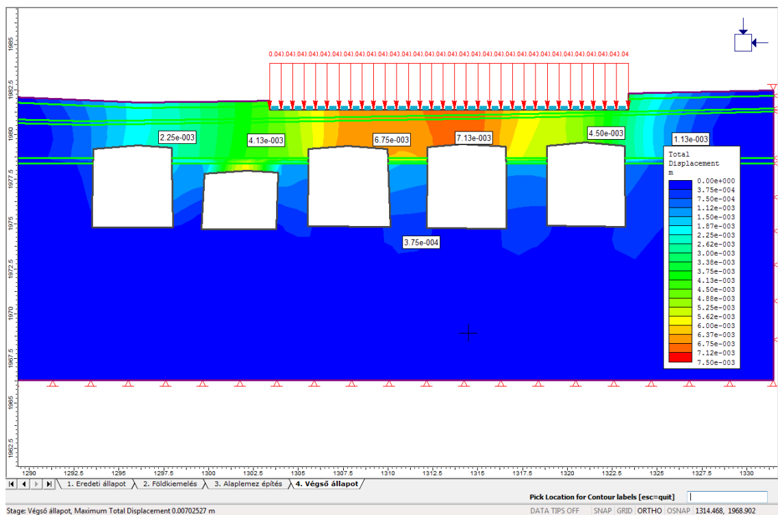
25. ábra. Az elmozdulások végző állapotban
