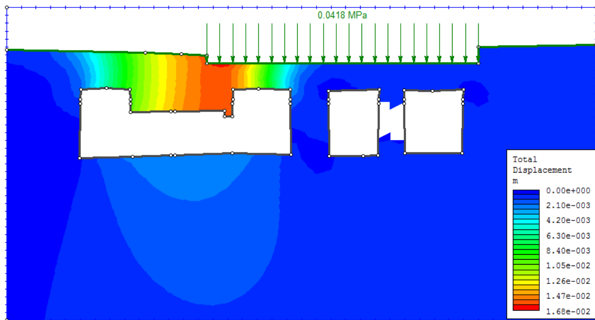
18. ábra. Az elmozdulások alakulása végleges állapotban (A km)
