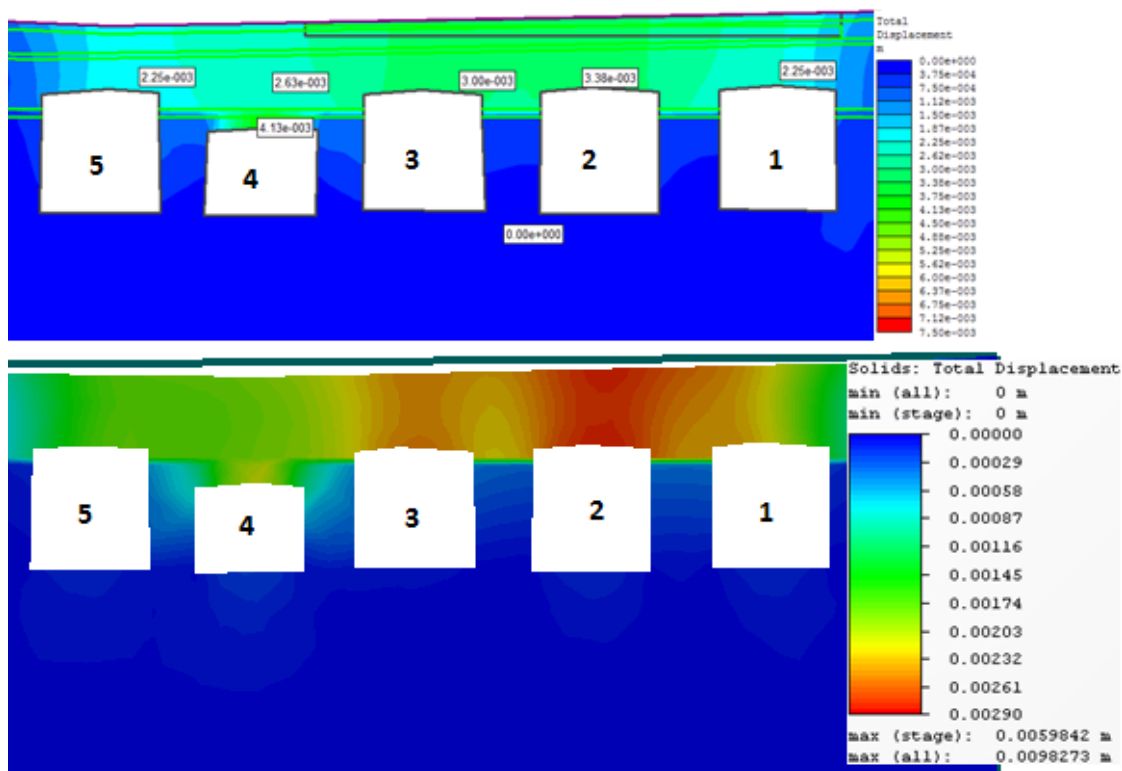
59. ábra. A elmozdulások összehasonlítása eredeti állapotban a (C km)
