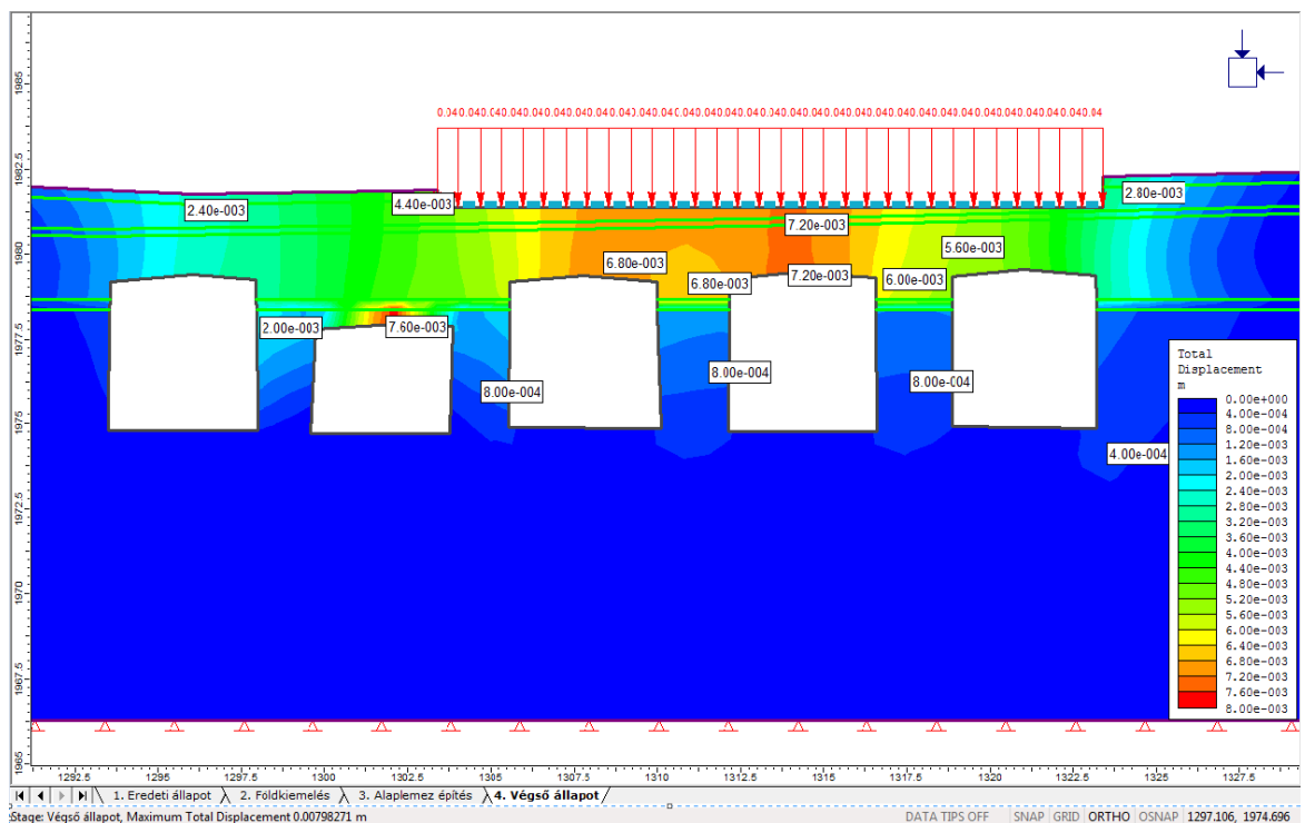
29. ábra. Az elmozdulások végső állapotban
