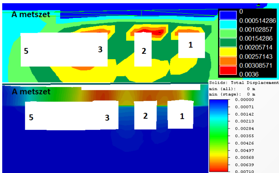
56. ábra. Az elmozdulások összehasonlítás végleges állapotban (A km)
