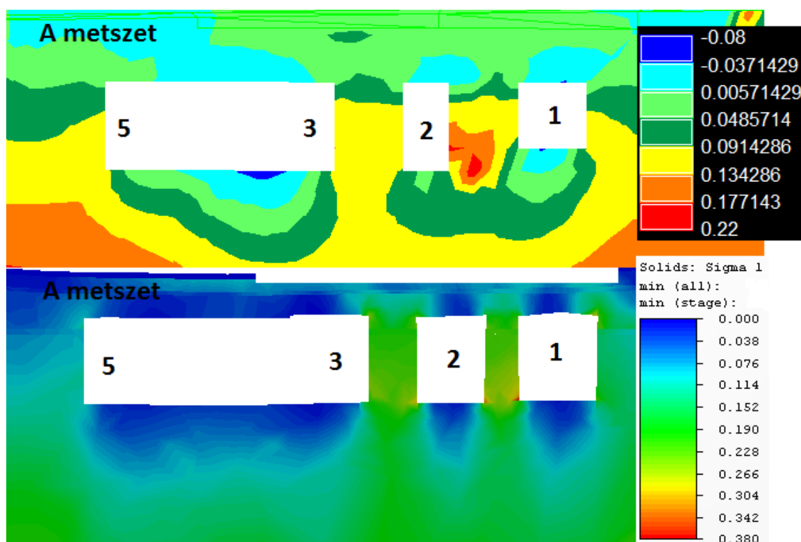
52.ábra. A feszültségek összehasonlítása végleges állapotban (A km)
