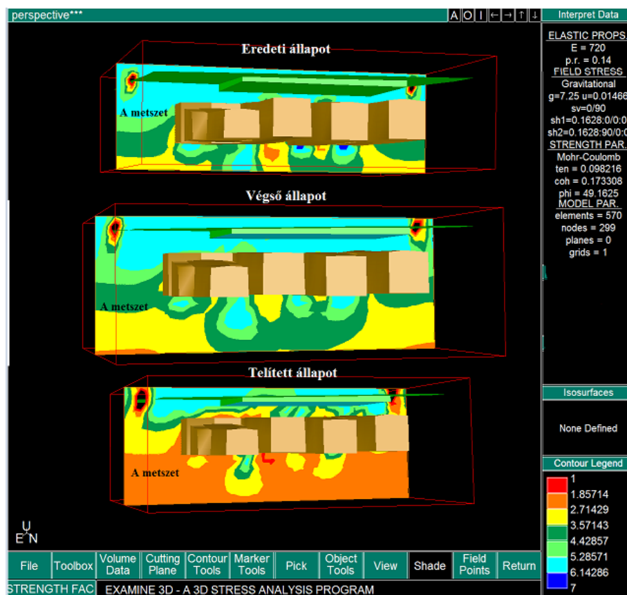
34. ábra. A teherbírási tényező változása a különböző állapotokban
