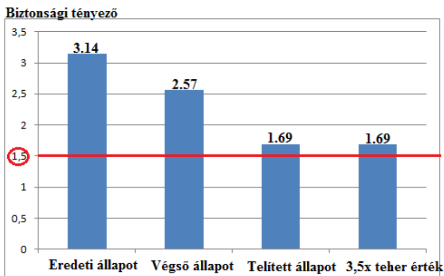
32. ábra. Biztonsági tényezők alakulása különböző esetekben
