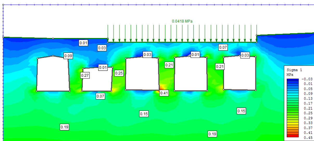
11. ábra. A \sigma_1 feszültség véleges állapotban
