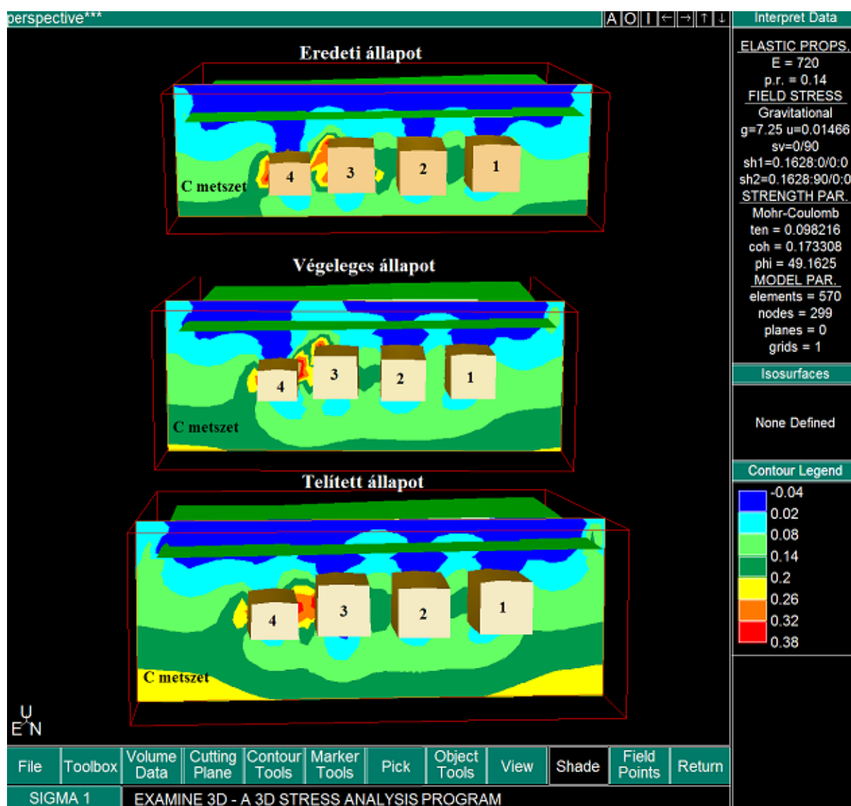
35. ábra. A \sigma_1 feszültség változása a különböző állapotokban
