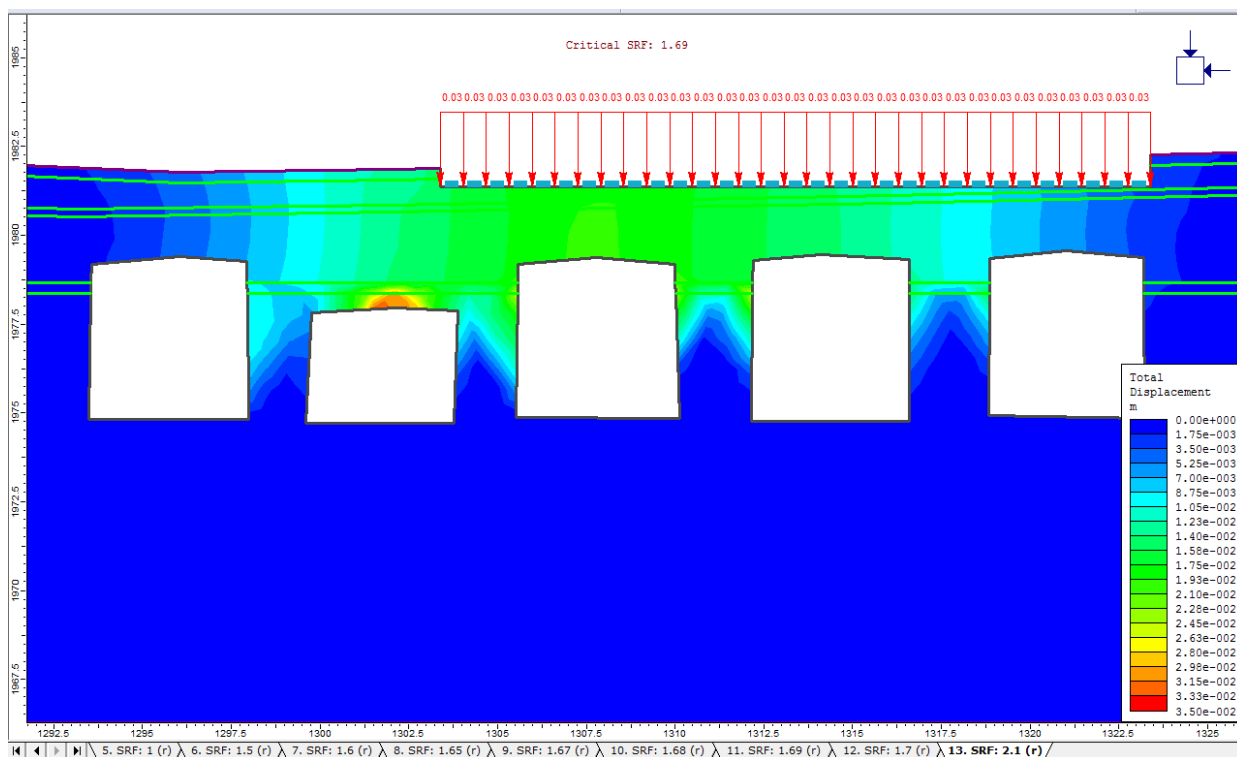
31. ábra. A biztonsági tényező végső állapotban
