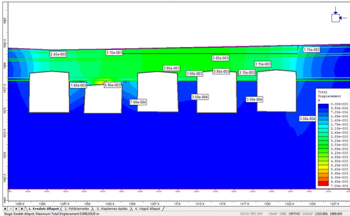
28. ábra. Az elmozdulások eredeti állapotban
