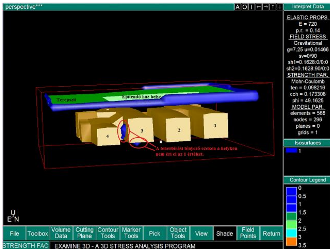
38. ábra. A teherbírási tényező 1 alatti értékeinek helye
