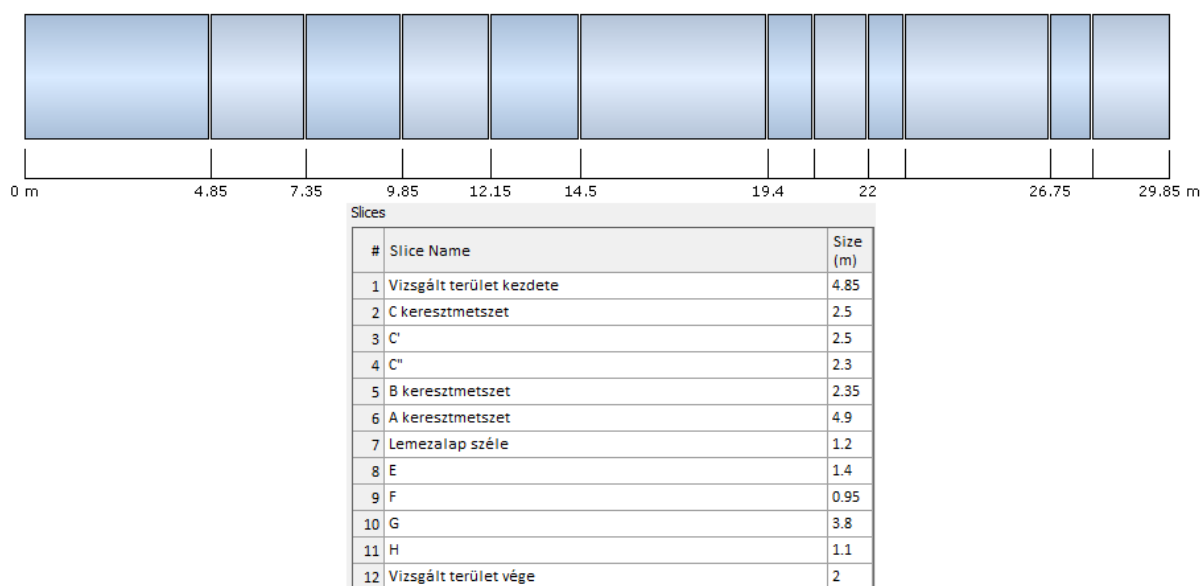
39. ábra. A definiált keresztmetszetek és a hosszai
