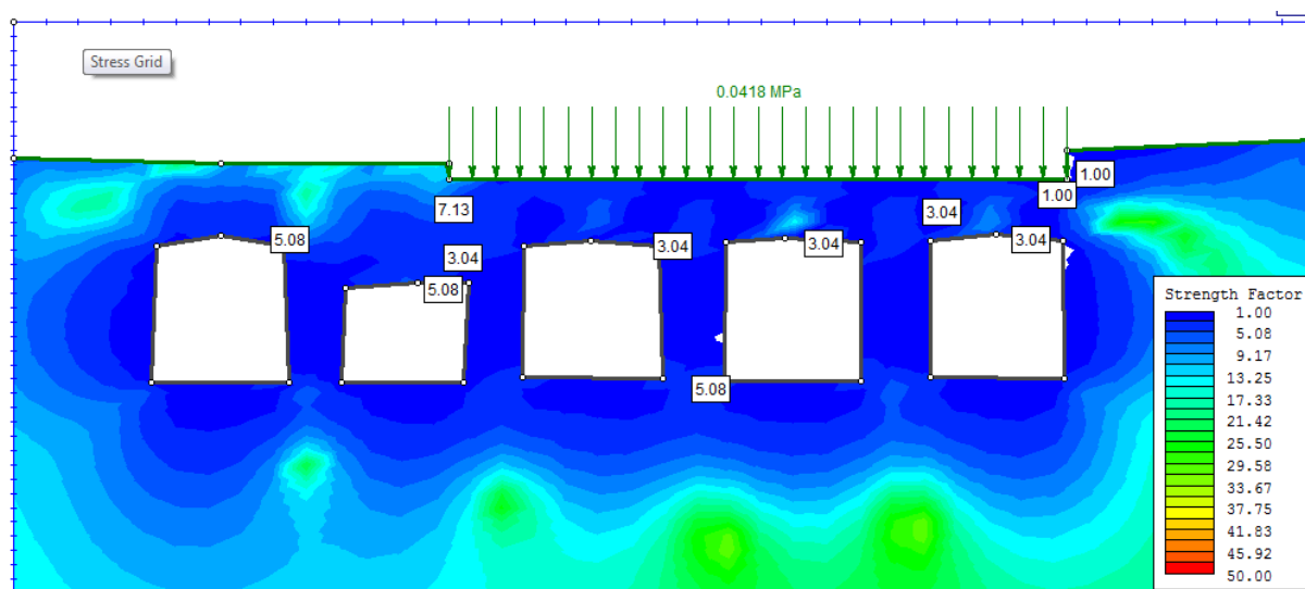
15. ábra. Az teherbírási tényező alakulása végleges állapotban
