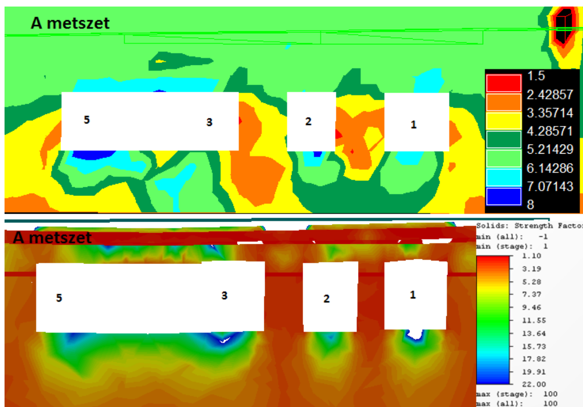
53. ábra. A teherbírési tényező összehasonlítás eredeti állapotban (A km)
