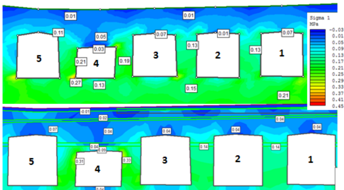
47. ábra. Az feszültségek összehasonlítása eredeti állapotban
