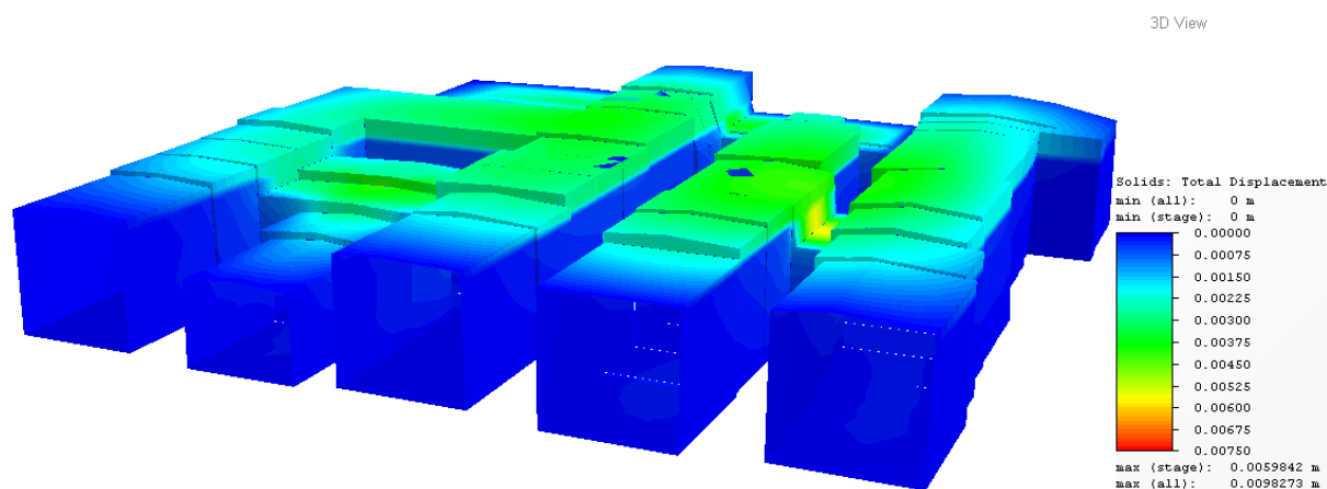
45. ábra. Az elmozdulások alakulása eredeti állapotban
