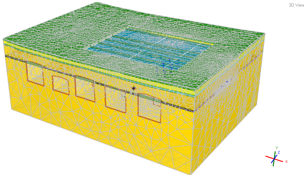
40. ábra. A 3D-s modell és a végelem háló
