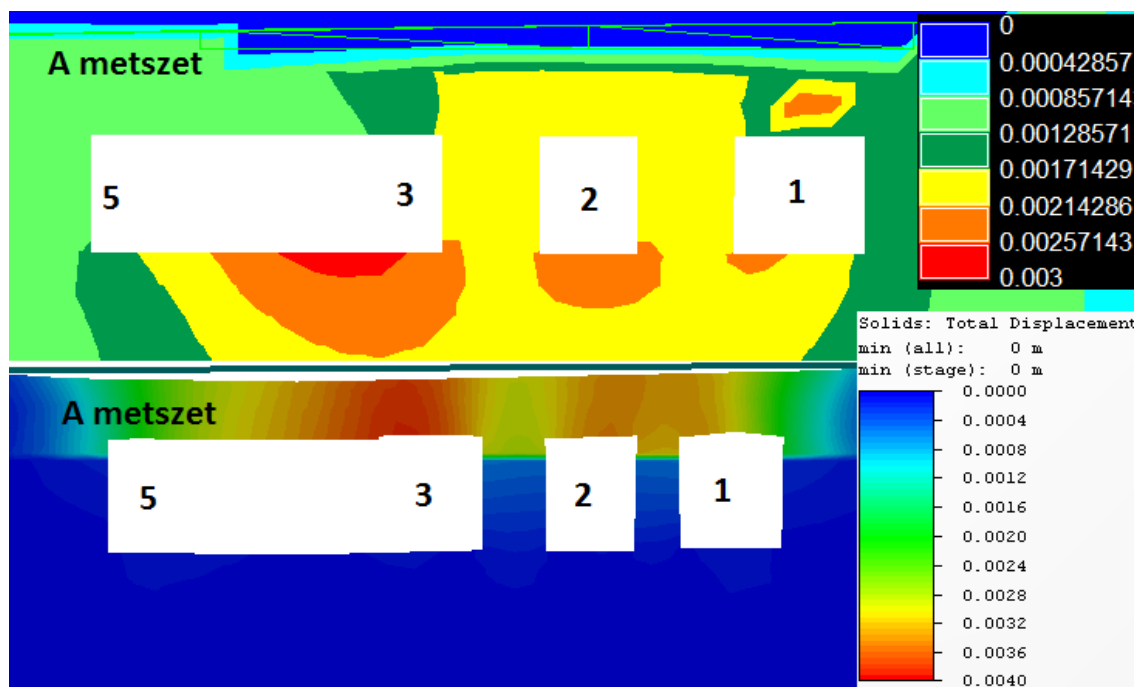
55. ábra. Az elmozdulások összehasonlítás eredeti állapotban (A km)
