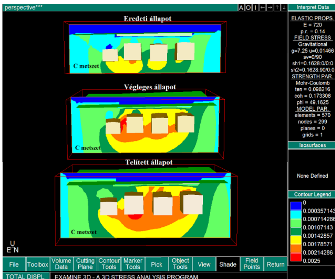
36. ábra. Az elmozdulások változása a különböző állapotokban
