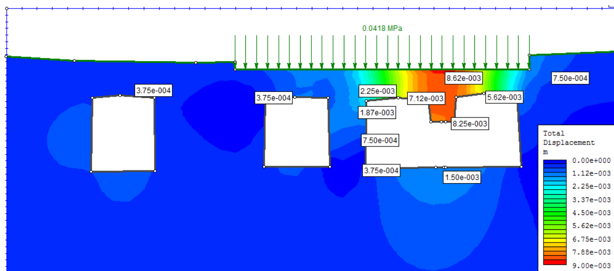
17. ábra. Az elmozdulások alakulása végleges állapotban (B km)
