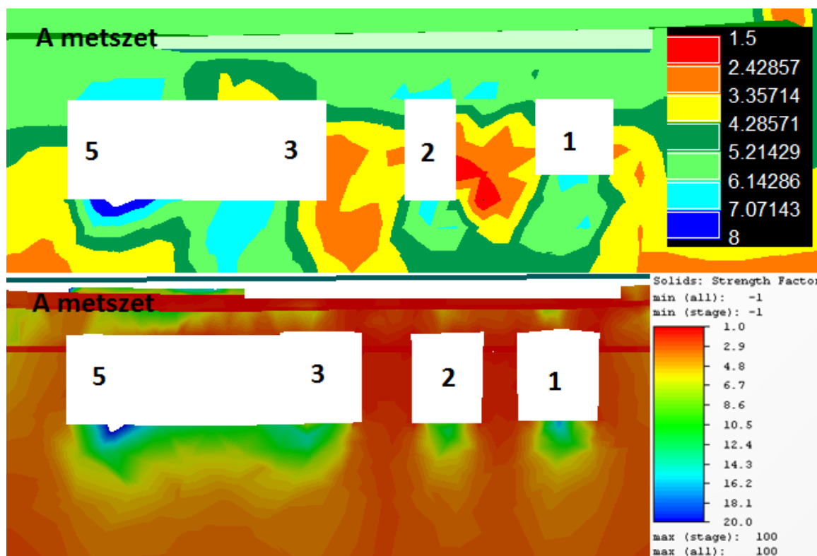
54. ábra. A teherbírési tényező összehasonlítás végleges állapotban (A km)
