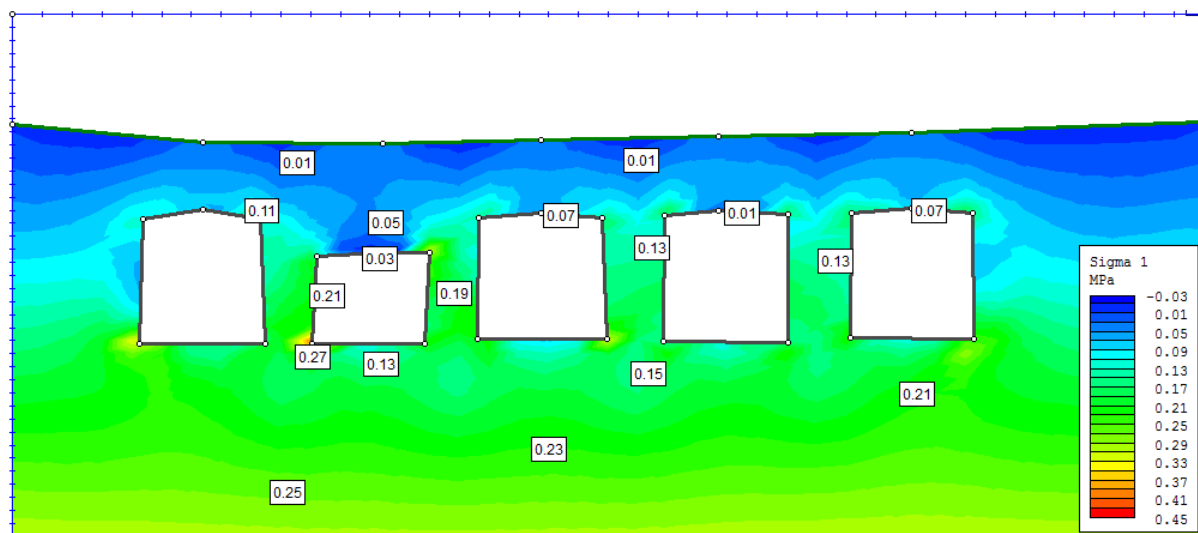
10. ábra. A \sigma_1 feszültség eredeti állapotban
