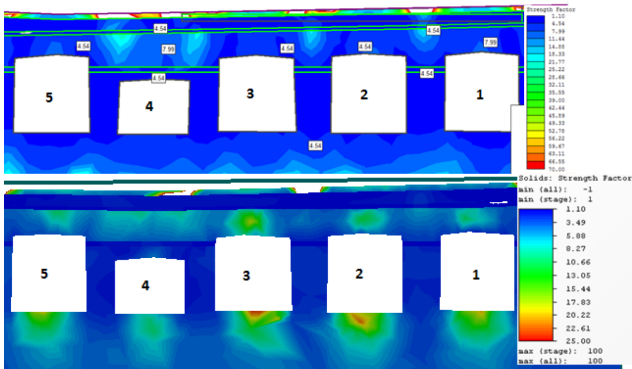
57. ábra. A teherbírési tényező összehasonlítás eredeti állapotban (C km)
