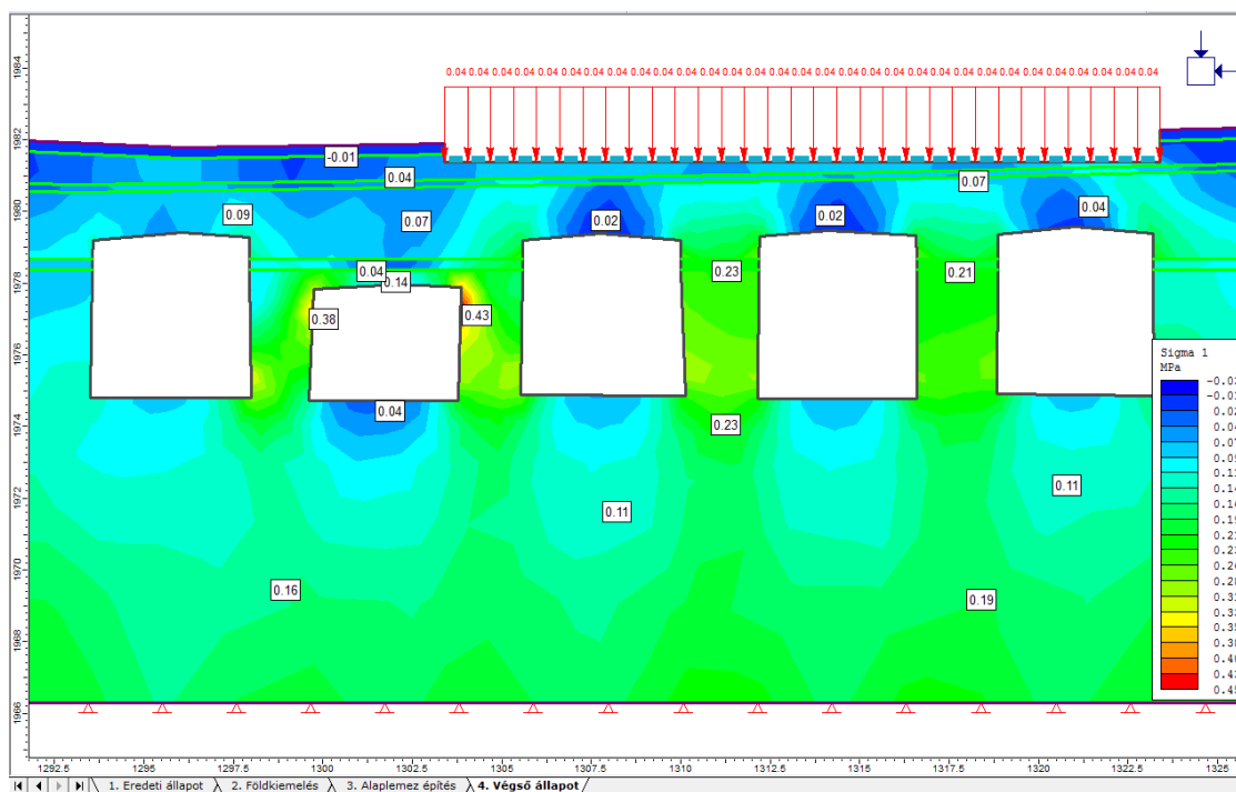
21. ábra. A \sigma_1 feszültség végső állapotban
