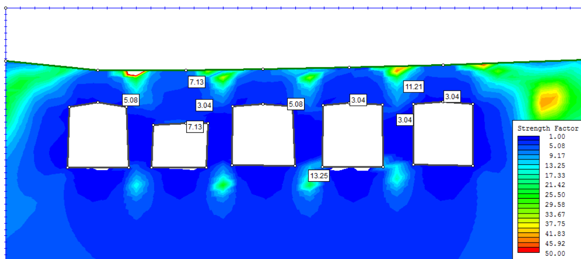
14. ábra. Az teherbírási tényező alakulása eredeti állapotban
