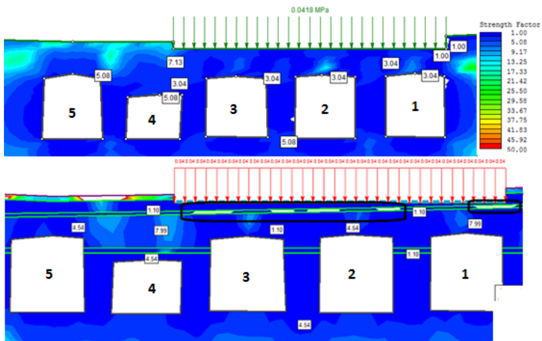
49.ábra. A teherbírási tényező összehasonlítása végleges állapotban
