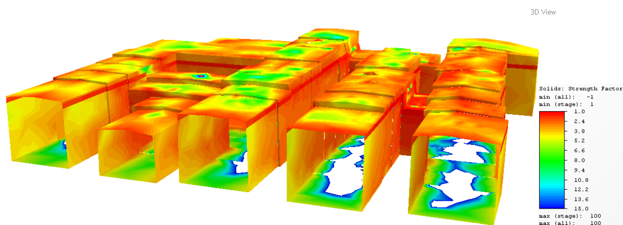
43. ábra. Az teherbírási tényező alakulása eredeti állapotban
