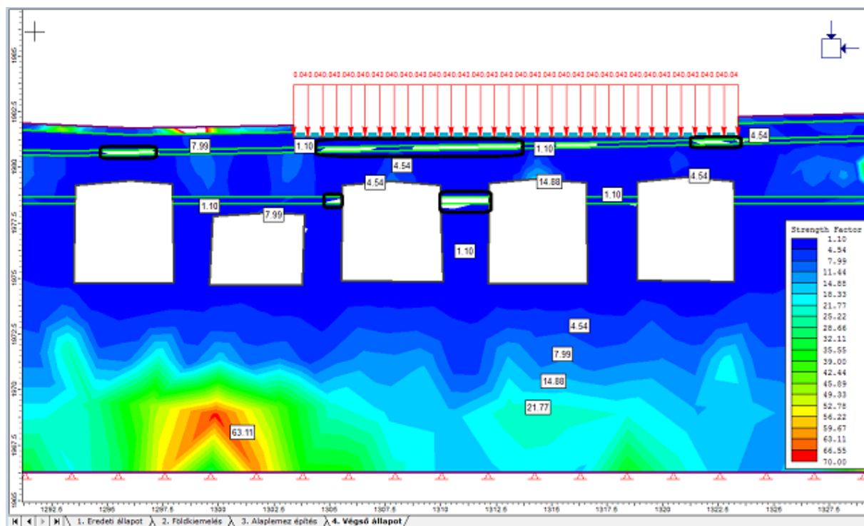
30. ábra. Az teherbírási tényező végső állapotban
