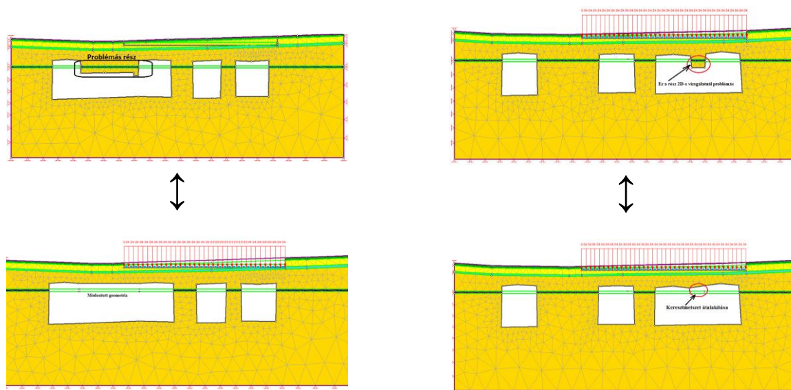
19. ábra. A pincék geometriájának módosítása
