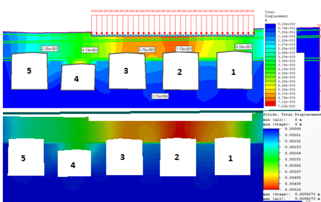
60. ábra. Az elmozdulások összehasonlítása végleges állapotban (C km)
