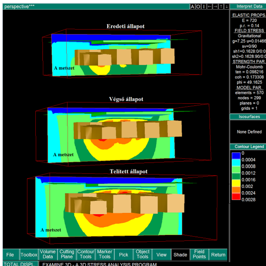
33. ábra. Az elmozdulások változása a különböző állapotokban
