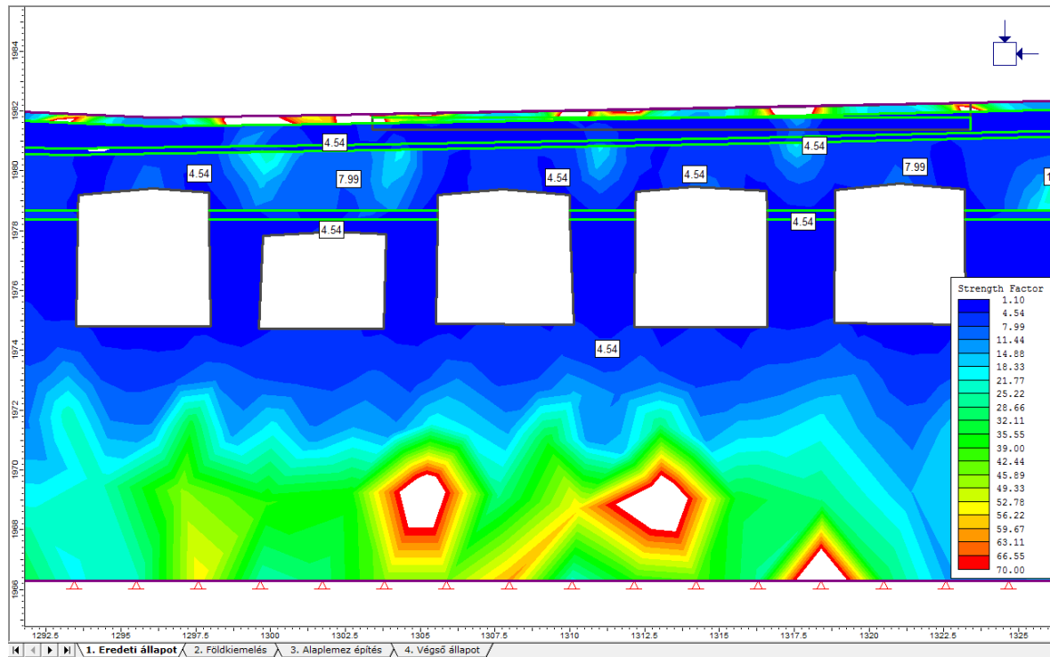
22. ábra. Az teherbírási tényező eredeti állapotban
