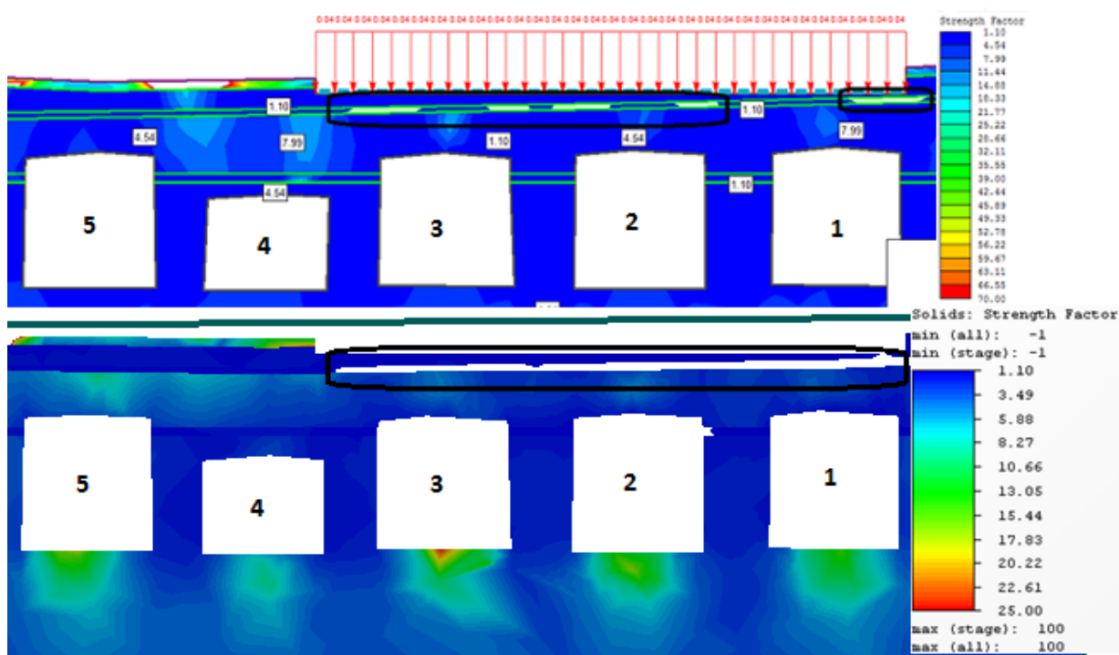
58. ábra. A teherbírési tényező összehasonlítás végleges állapotban (C km)
