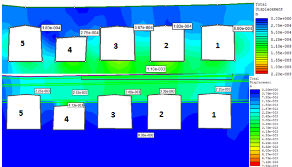
50.ábra. Az elmozdulások összehasonlítása eredeti állapotban
