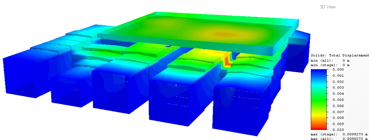
46. ábra. Az elmozdulások alakulása végső állapotban
