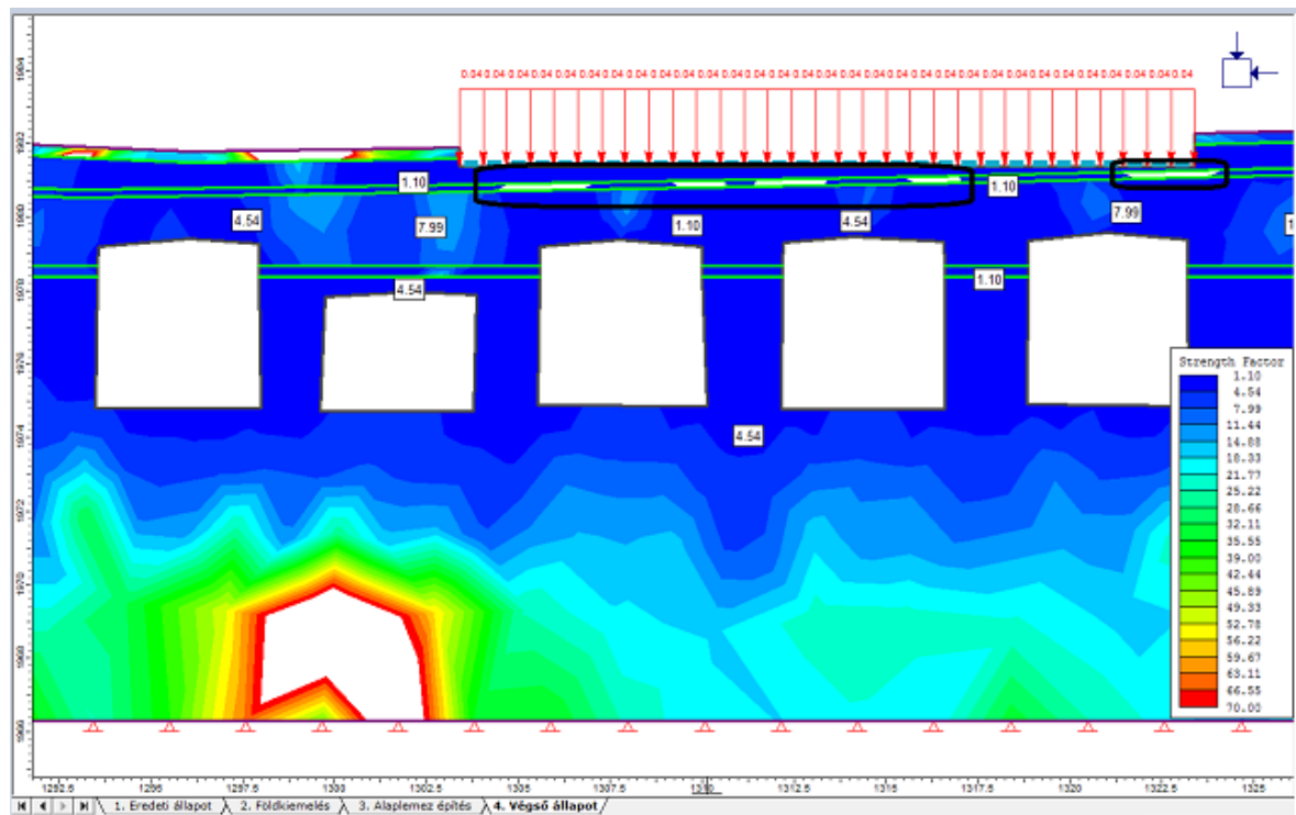
43. 23. ábra. A teherbírási tényező végső állapotban
