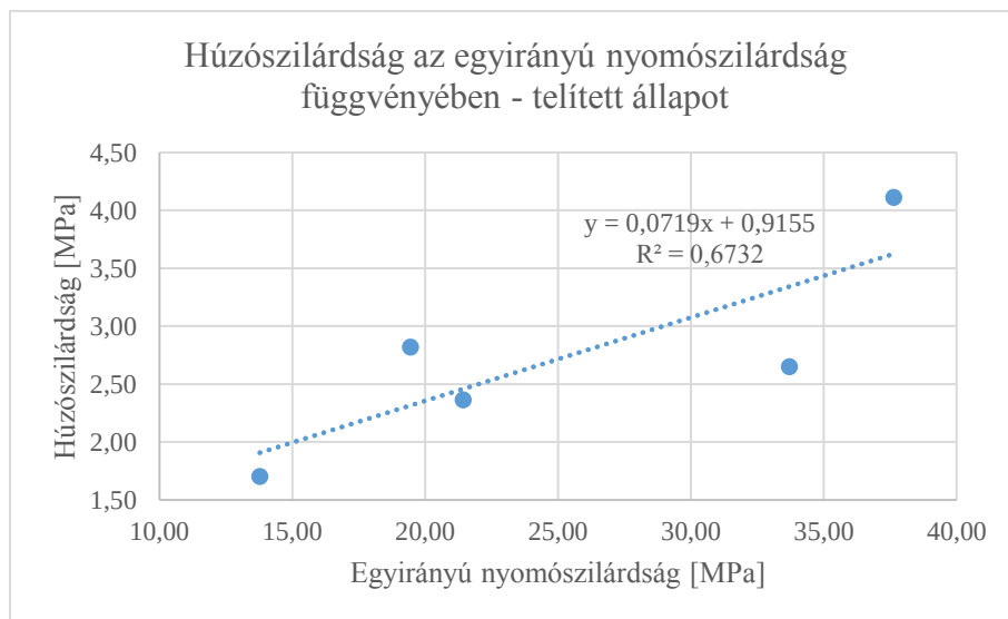
28. ábra: A szilárdsági jellemzők átlagértékeinek az összefüggése telített állapotban
