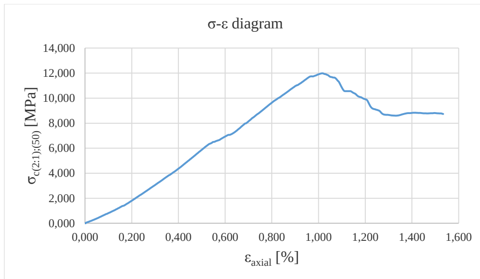
6. ábra: A VK-1/8-1 jelű próbatest feszültség-alakváltozás diagramja
