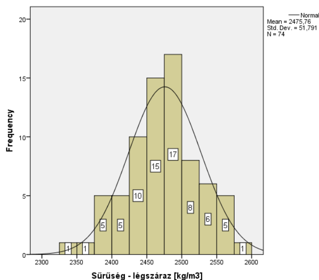
11. ábra: A légszár állapotban mért sűrűség eloszlása hisztogrammal ábrázolva (Várkert-2013, fakószürke mészmárga)
