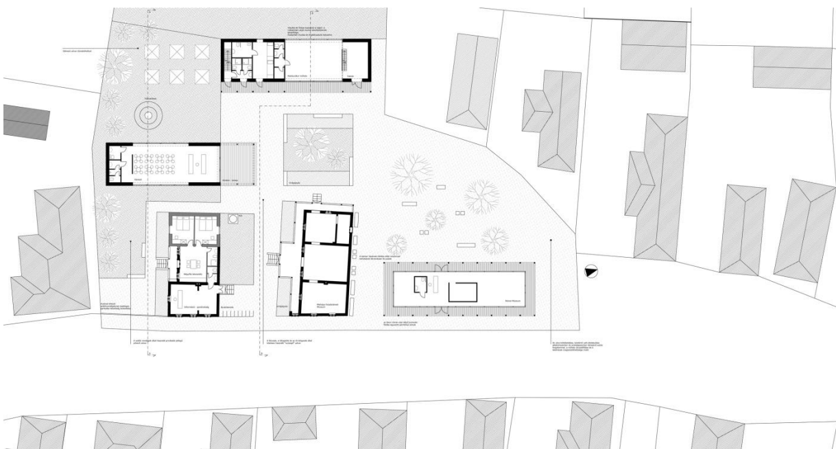
Helyszínrajz az új beépítésről
