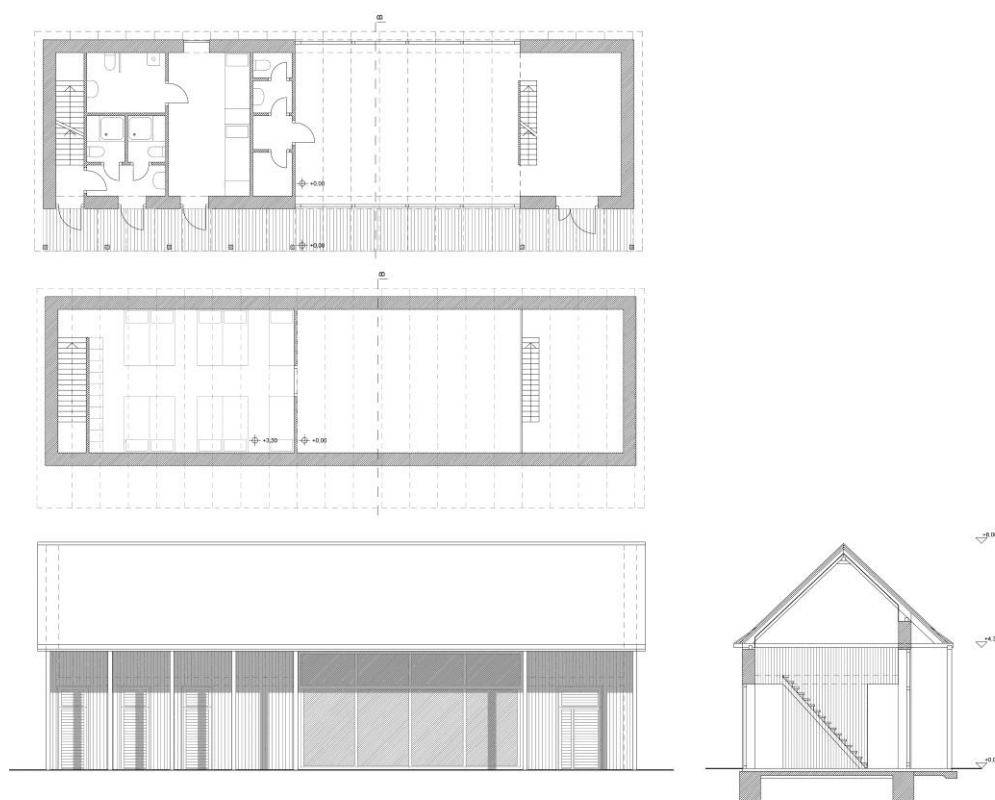
Alaprajzok, homlokzat és metszet
