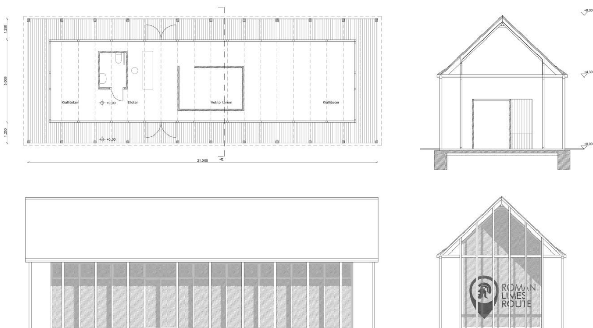
Alaprajz, metszet és homlokzatok
