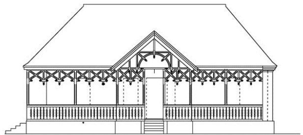
A meglévő épület felmérési rajzai
