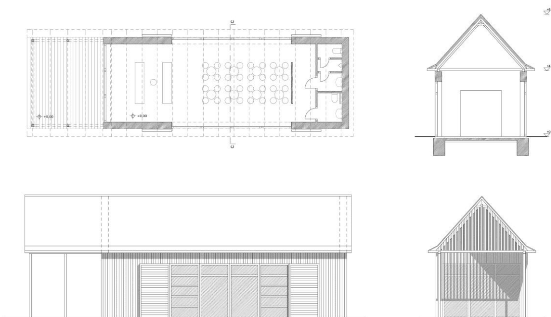
Alaprajz, metszet és homlokzatok
