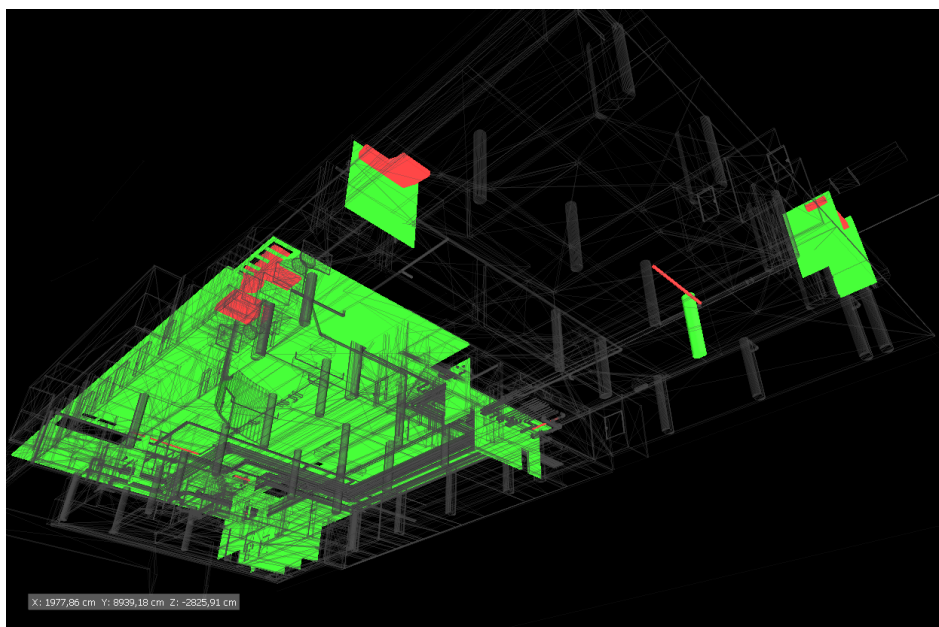
6.15. ábra: Az általunk előállított 3D-s modellben a légtechnika és a tartószerkezet ütközései a pinceszinten
