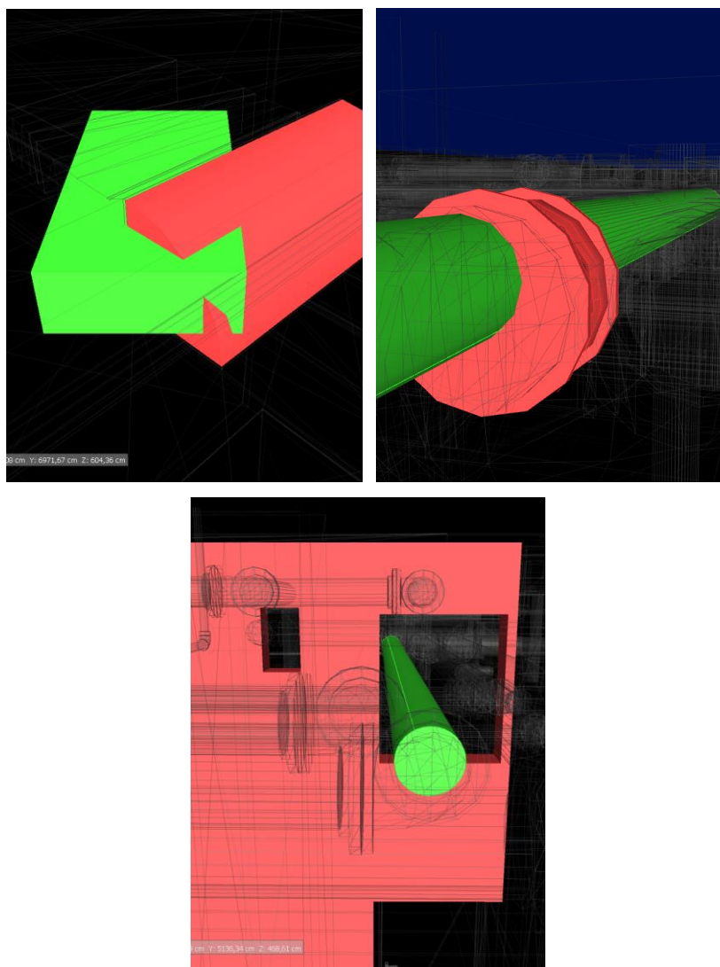
4.1. ábra: Tervek ütközésvizsgálatának kritériumai (bal oldali kép: egymásba metszések kimutatása, középső kép: egymáson belülségek kimutatása, jobb oldali kép: szükséges védőtávolságon belülség kimutatása)
