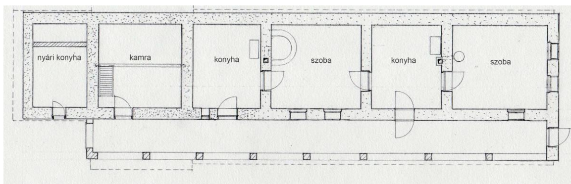
38. kép: A Mayer-ház '50-es években módosult állapota (forrás: saját ábra)
