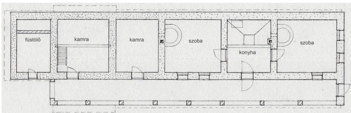
17. kép: A Greksa-ház építéskori alaprajza (forrás: saját ábra)
