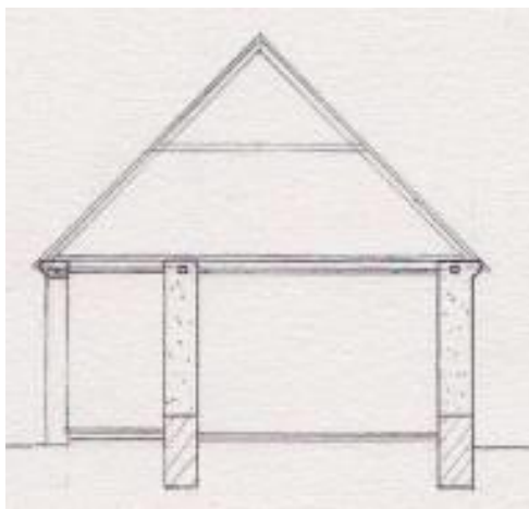
41. A Mayer-ház metszete az aláfalazás után
