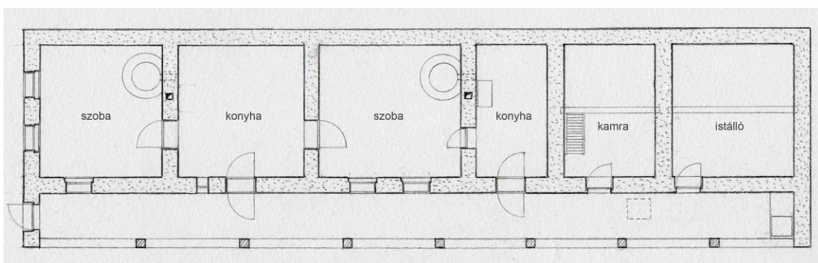
19. kép: A Huber-ház építéskori alaprajza (forrás: saját ábra)
