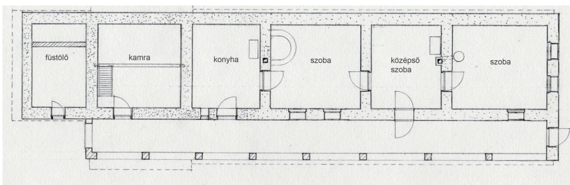
44. kép: A Mayer-ház 1960-ban módosult állapota (forrás: saját ábra)
