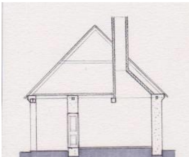
35. kép: Metszet a Mayer-ház ról (forrás: saját ábra)
