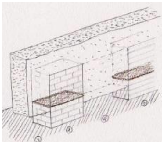
41. A Mayer-ház metszete az aláfalazás után
