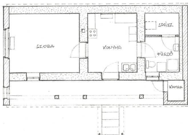
83. Az Ignéczi-házban kialakított fürdő (forrás: saját ábra)
