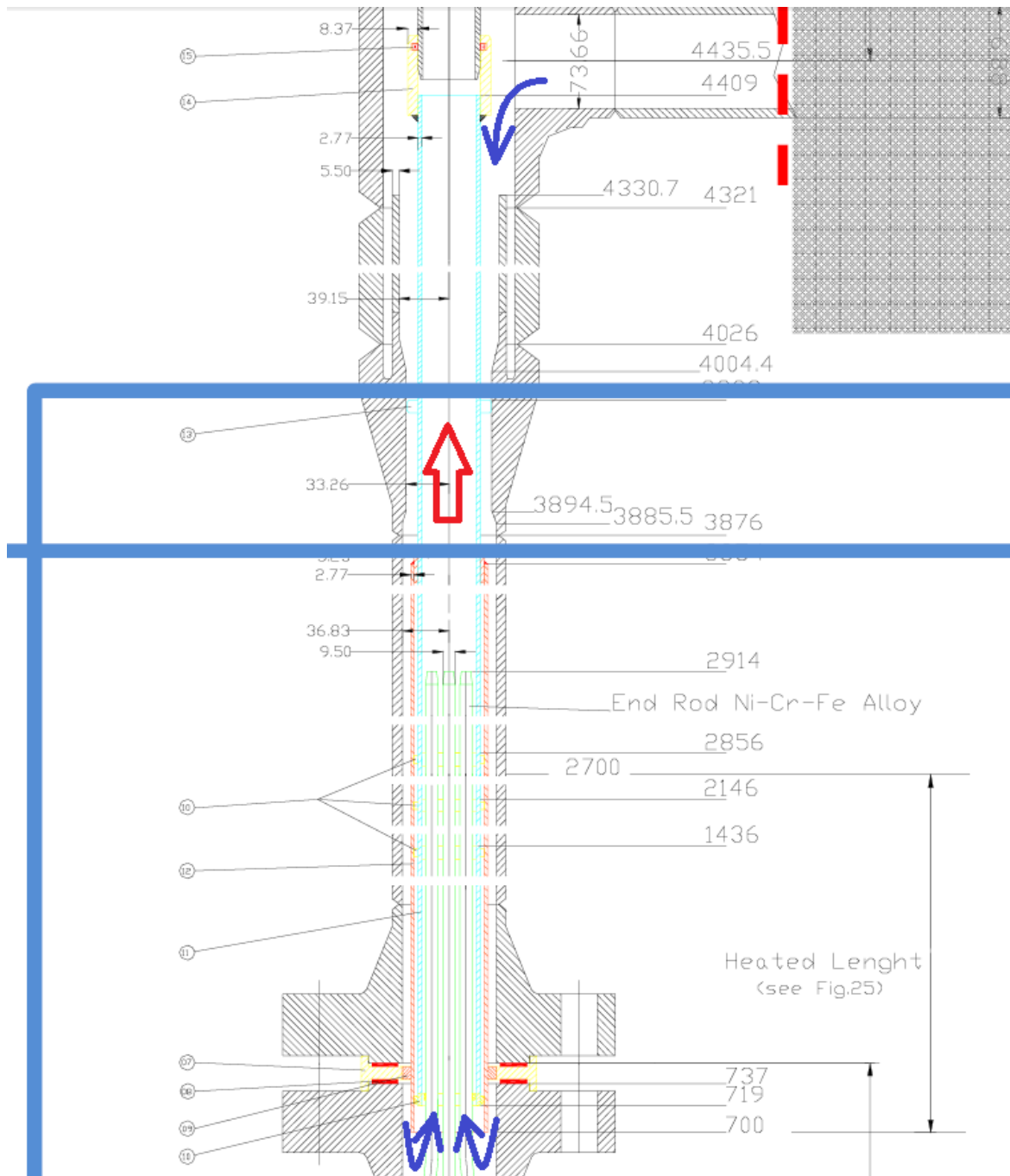
6. ábra: A teszszakasz hosszszelvényi képe (a kék vonal a teljes ábrán a kinagyított részeket jelöli. Lásd melléklet 1. ábra)
