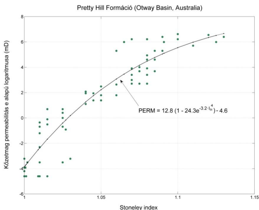
17. ábra: Pretty Hill formáció nemlineáris permeabilitás modellje
