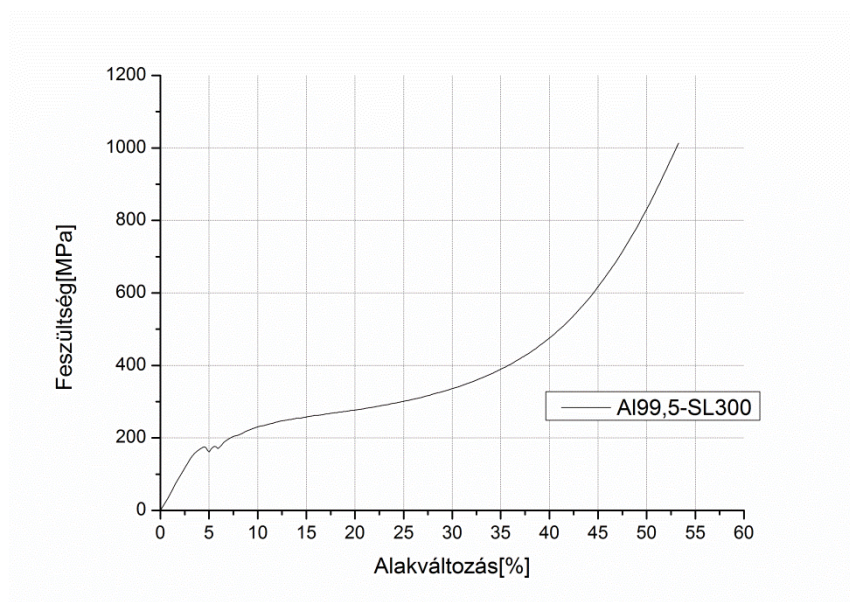
ábra, Al99,5-SL300 mátrixú fémhab
