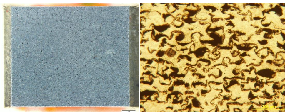
. ábra, Al99,5-SL150 mátrixú fémhab
