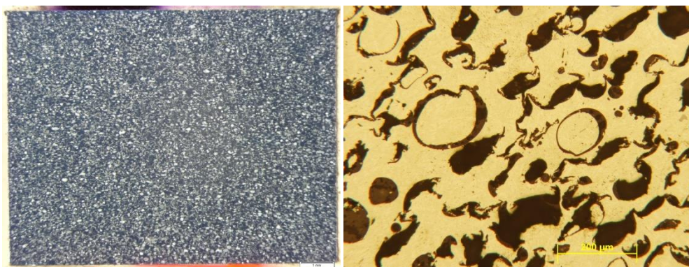
. ábra, AlSi12-SL300 mátrixú fémhab
