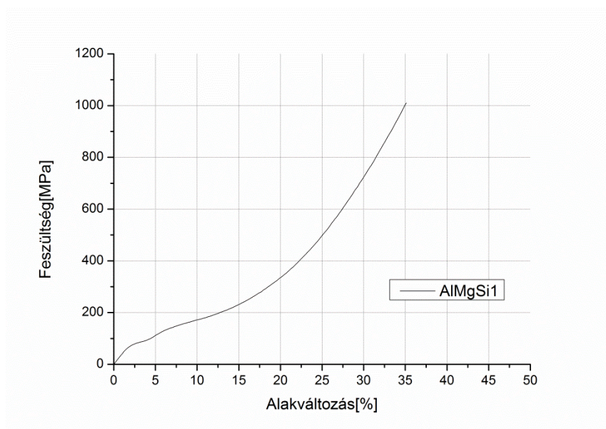
. ábra, AlMgSi1 mátrixú fémhab
