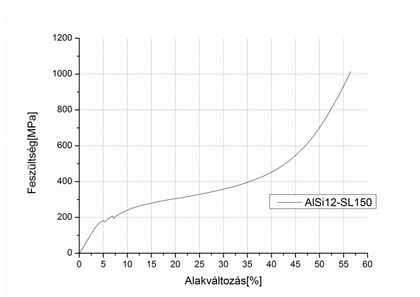
. ábra, AISi12-SL150 mátrixú fémhab
