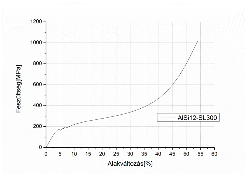
. ábra, AlSi12-SL300 mátrixú fémhab
