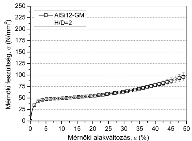
1.30. ábra AlSi12 – GM nyomógörbéinek átlaggörbéje
