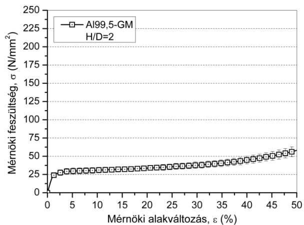
1.29. ábra Al99,5 – GM nyomógörbéinek átlaggörbéje
