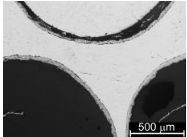
1.16. ábra Az AlCu5-GM próbatest polírozott mintájának fénymikroszkópos képe
