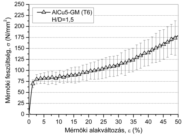
1.40. ábra AlCu5 – GM (T6) nyomógörbéinek átlaggörbéje
