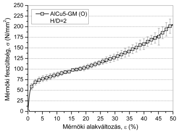
1.41. ábra AlCu5 – GM (O) nyomógörbéinek átlaggörbéje
