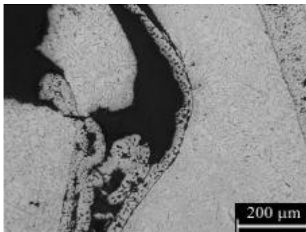
1.12. ábra Az AlSi12-GM zömített próbatest maratott mintájának fénymikroszkópos képe
