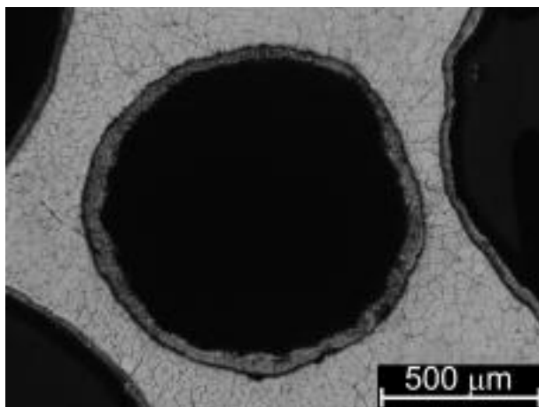
1.5. ábra Az Al99,5-GM próbatest maratott mintájának fénymikroszkópos fényképe
