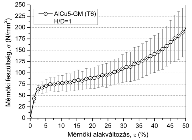
1.38. ábra AlCu5 – GM (T6) nyomógörbéinek átlaggörbéje
