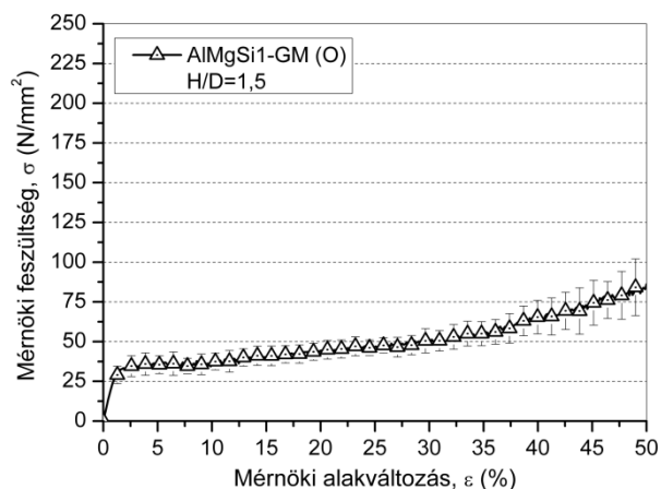
1.33. ábra AlMgSi1 – GM (O) nyomógörbéinek átlaggörbéje
