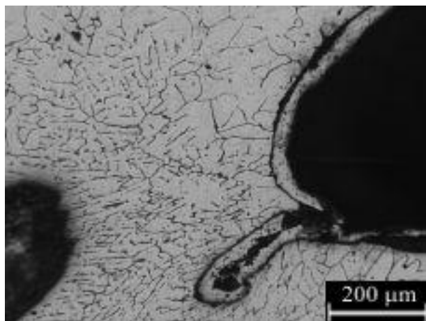
1.11. ábra Az Al99,5-GM zömített próbatest maratott mintájának fénymikroszkópos képe
