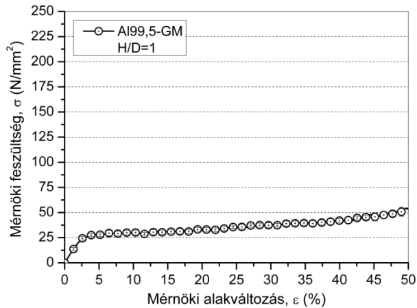
1.25. ábra Al99,5 – GM nyomógörbéinek átlaggörbéje
