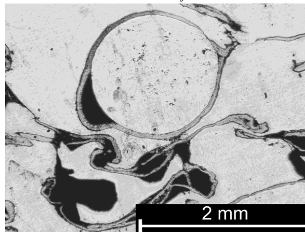
1.22. ábra Az AlCu5-GM zömített próbatest polírozott mintájának fénymikroszkópos képe
