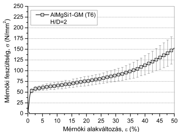
1.36. ábra AlMgSi1 – GM (T6) nyomógörbéinek átlaggörbéje
