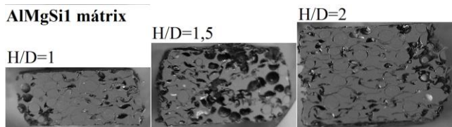
1.19. ábra Az AlMgSi1-GM zömített próbatest mintájának makrofotója
