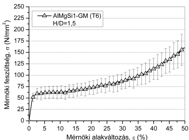
1.34. ábra AlMgSi1 – GM (T6) nyomógörbéinek átlaggörbéje
