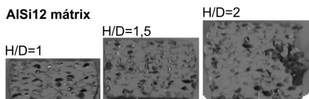
1.8. ábra Az AlSi12-GM zömített próbatest mintájának makrofotója
