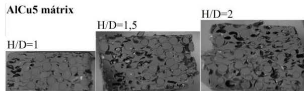
1.20. ábra Az AlCu5-GM zömített próbatest mintájának makrofotója
