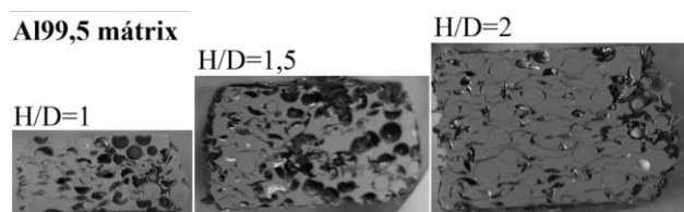
1.7. ábra Az Al99,5-GM zömített próbatest mintájának makrofotója
