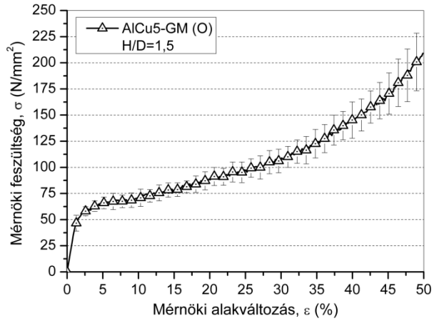
1.39. ábra AlCu5 – GM (O) nyomógörbéinek átlaggörbéje
