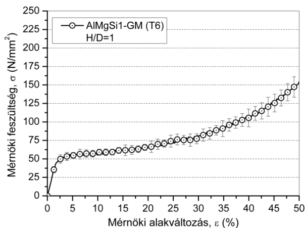
1.32. ábra AlMgSi1 – GM (T6) nyomógörbéinek átlaggörbéje
