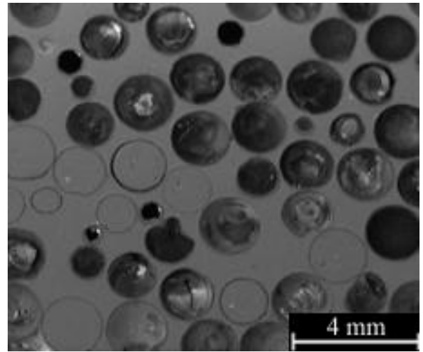
1.14. ábra Az AlCu5-GM próbatest polírozott mintájának makrofotója
