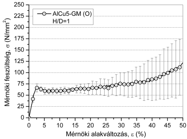
1.37. ábra AlCu5 – GM (O) nyomógörbéinek átlaggörbéje
