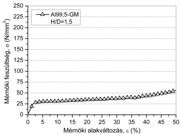
1.27. ábra Al99,5 – GM nyomógörbéinek átlaggörbéje
