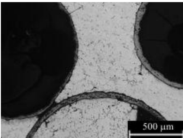
1.17. ábra Az AlMgSi1-GM próbatest maratott mintájának fénymikroszkópos fényképe
