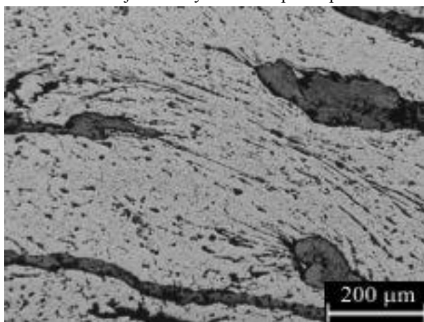
1.23. ábra Az AlMgSi1-GM zömített próbatest maratott mintájának fénymikroszkópos képe
