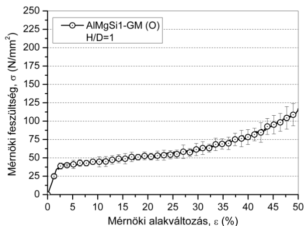
1.31. ábra AlMgSi1 – GM (O) nyomógörbéinek átlaggörbéje
