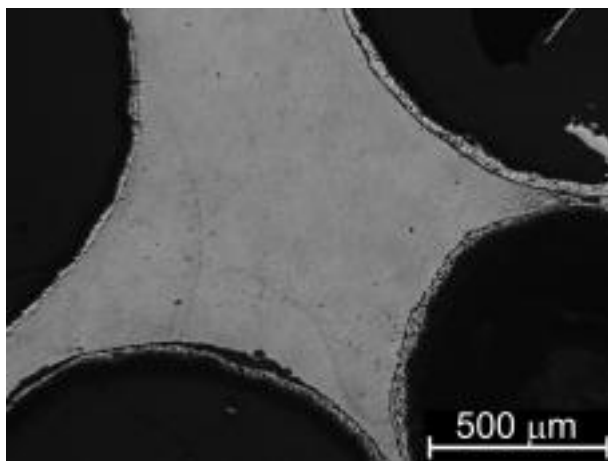
1.3. ábra Az Al99,5-GM próbatest polírozott mintájának fénymikroszkópos képe
