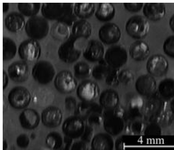
1.2. ábra Az AlSi12-GM próbatest polírozott mintájának makroszkópikus fényképe
