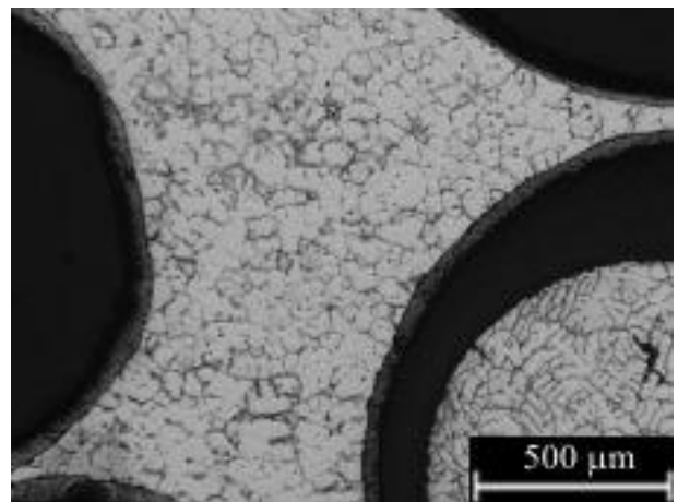
1.18. ábra Az AlCu5-GM próbatest maratott mintájának fénymikroszkópos fényképe
