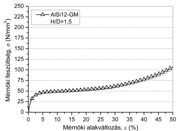
1.28. ábra AlSi12 – GM nyomógörbéinek átlaggörbéje
