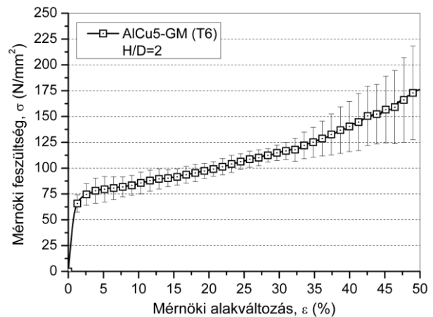
1.42. ábra AlCu5 – GM (T6) nyomógörbéinek átlaggörbéje
