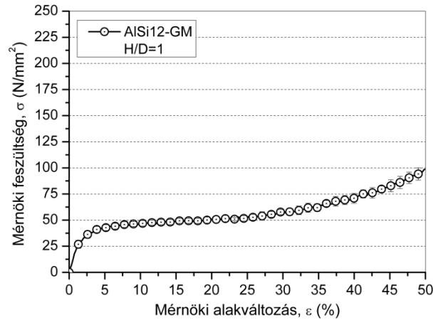
1.26. ábra AlSi12 – GM nyomógörbéinek átlaggörbéje
