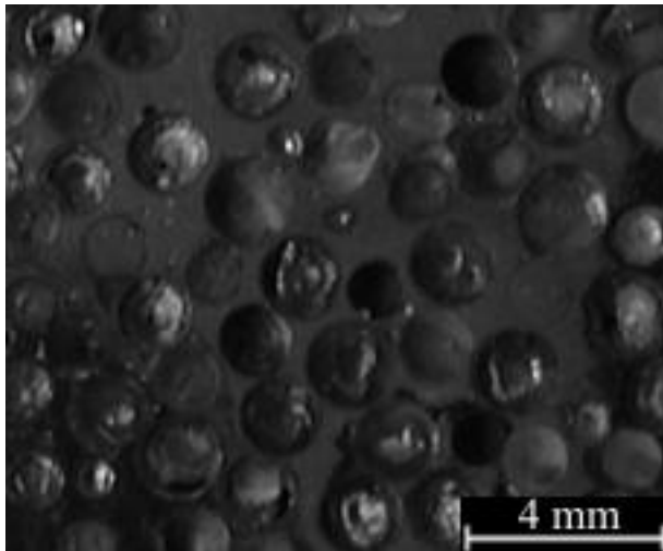
1.13. ábra Az AlMgSi1-GM próbatest polírozott mintájának makrofotója
