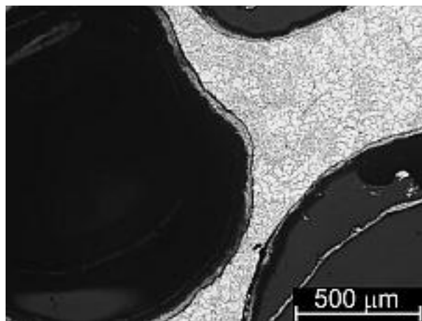
1.6. ábra Az AlSi12-GM próbatest maratott mintájának fénymikroszkópos fényképe
