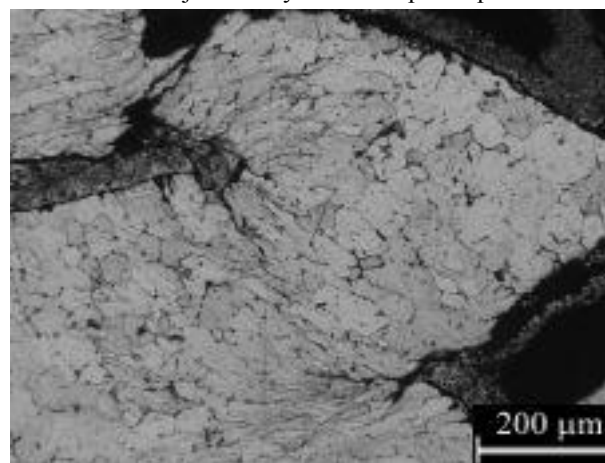
1.24. ábra Az AlCu5-GM zömített próbatest maratott mintájának fénymikroszkópos képe
