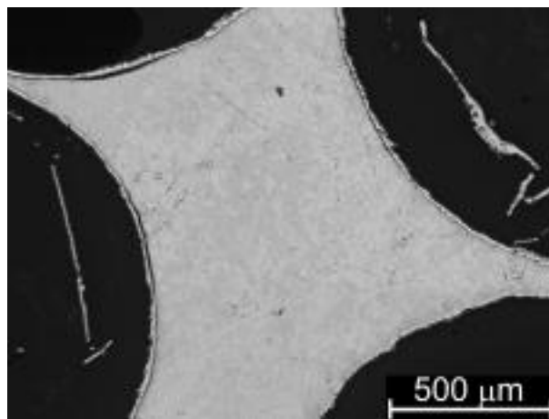
1.4. ábra Az AlSi12-GM próbatest polírozott mintájának fénymikroszkópos képe
