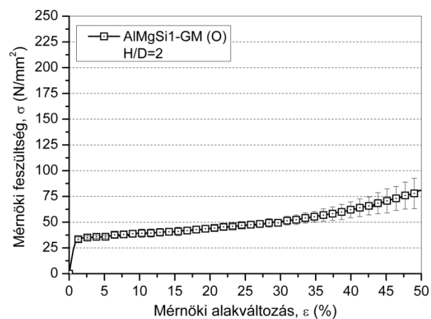
1.35. ábra AlMgSi1 – GM (O) nyomógörbéinek átlaggörbéje
