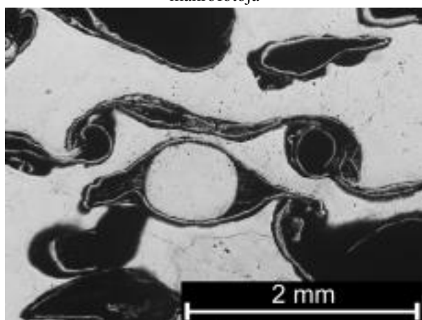
1.9. ábra Az Al99,5-GM zömített próbatest polírozott mintájának fénymikroszkópos képe
