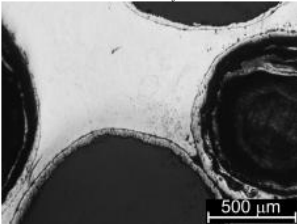
1.15. ábra Az AlMgSi1-GM próbatest polírozott mintájának fénymikroszkópos képe
