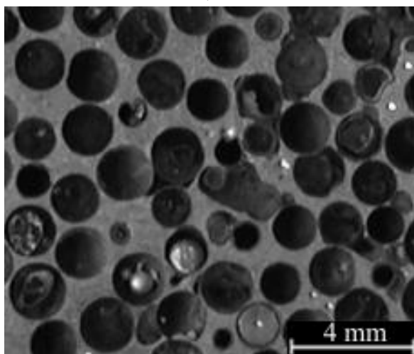
1.1. ábra Az Al99,5-GM próbatest polírozott mintájának makrofotója
