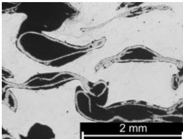
1.21. ábra Az AlMgSi1-GM zömített próbatest polírozott mintájának fénymikroszkópos képe
