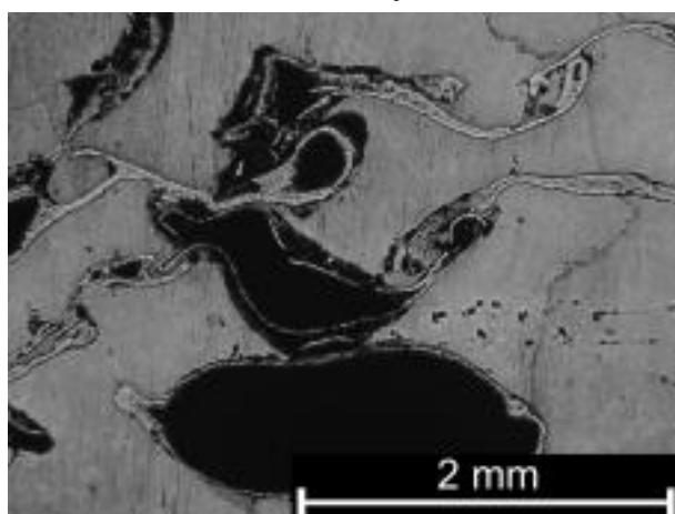
1.10. ábra Az AlSi12-GM zömített próbatest polírozott mintájának fénymikroszkópos képe
