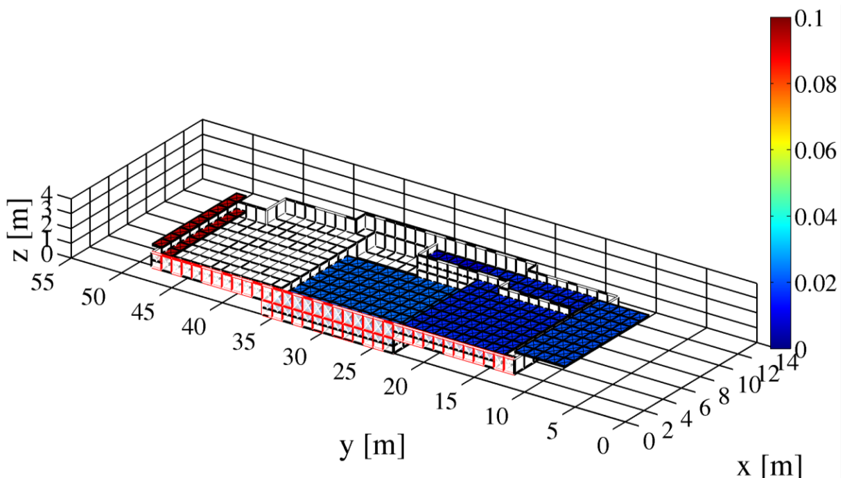
7.8. ábra: Irányfüggetlen befűjt és elszívott tömegáram peremfeltételek a vizsgált térben. A színskala mértékegysége [kg/s].
