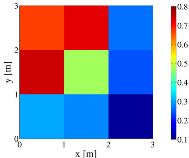
6.7. ábra: A sebesség kontúrjai a 2-es számú teszhelyiségben. A színskála mértékegysége [\text{m/s}] . A fal mellett nem nullának ábrázoltam jelen esetben a sebességet
