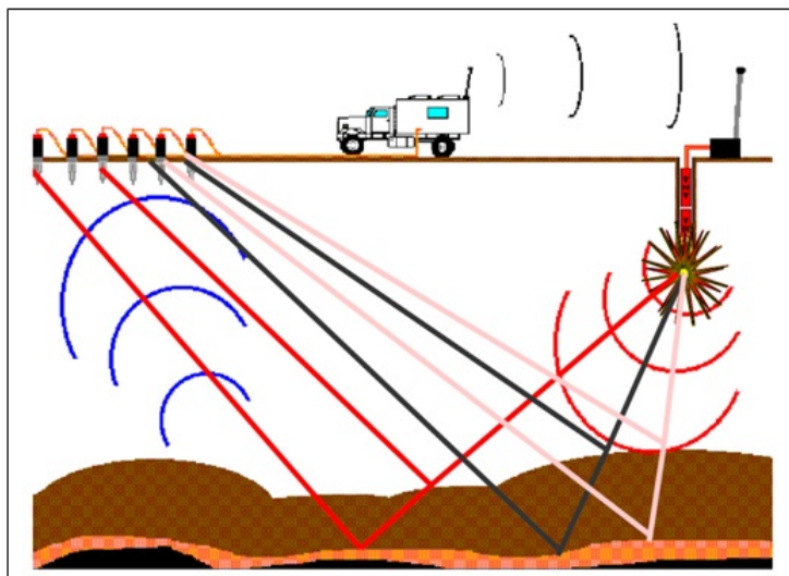
2.1. ábra. Szeizmikus mérés elvi vázlata (Forrás: Szűcs-,2006)
