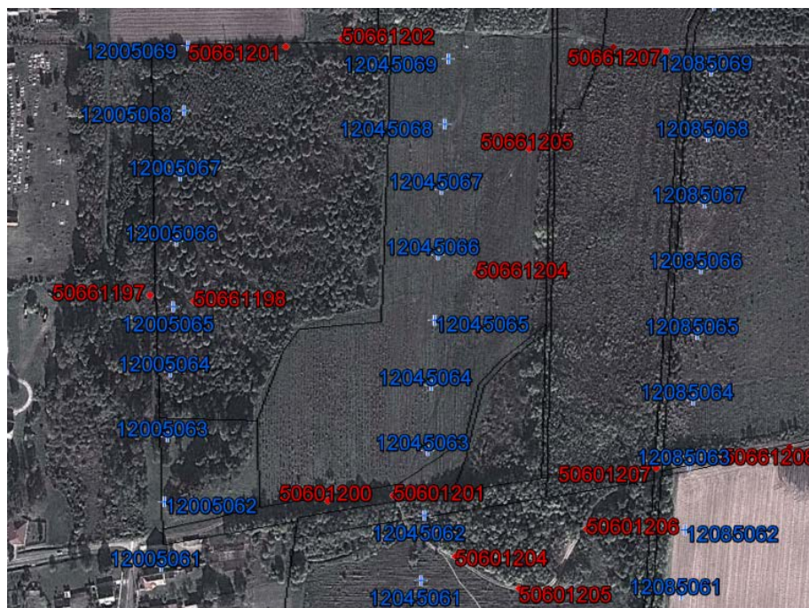
4.2. ábra. Földrészlet határok, megvalósult vibro és elméleti geofon pontok megjelenítése Google Earth segítségével (Forrás: MOL Görgeteg 3D projekt)
