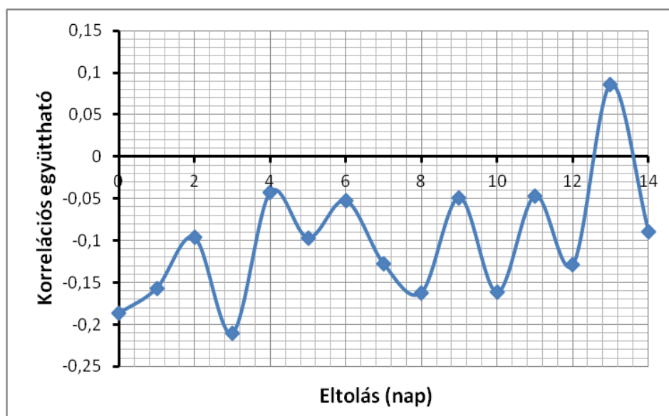
6.1. ábra Archív csapadék és vízhőmérséklet adatok keresztkorreláció függvénye
