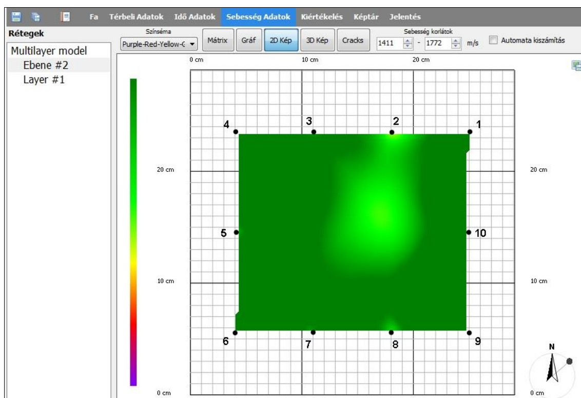
4. melléklet: A FAKOPP program képernyőképe négyzög keresztmetszetre történő alkalmazás közben
