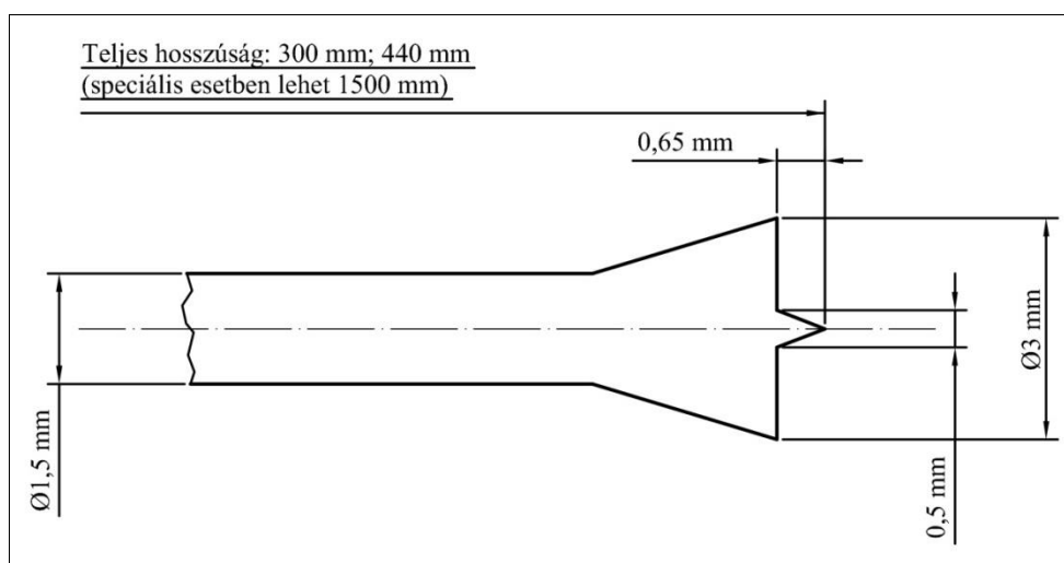
8. ábra: A Resistograph fúrójának speciális hegye (DÍVÓS, 2003)
